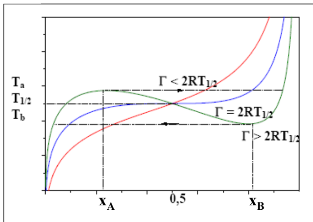
Figure I.5: Variation de la température en fonction de la fraction molaire HS : \Delta H = 600 \text{ cm}^{-1} et \Delta S = 4 \text{ cm}^{-1} \text{ K}^{-1} .
