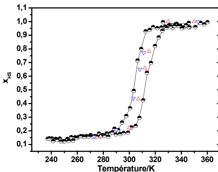
Figure IV.23: Comparaison des évolutions de la fraction HS en fonction de la température déduites de l'analyse magnétique (○) et de la spectroscopie Raman à basse fréquence (▲, ▼) pour les nanoparticules de [\text{Fe}(\text{NH}_2\text{-trz})_3](\text{Br})_2 \cdot 3\text{H}_2\text{O} \cdot 0,03(\text{tensioactif}) . Pour le magnétisme la fraction molaire en ions fer(II) HS, x_{\text{HS}} , est directement déduite du produit \chi_{\text{M}}T grâce à l'expression x_{\text{HS}} = \chi_{\text{M}}T / (\chi_{\text{M}}T)_{\text{HT}} où (\chi_{\text{M}}T)_{\text{HT}} est la valeur à la température limite, typiquement de 360 K. Pour la spectroscopie Raman, la fraction HS est obtenue à partir de la différence d'intensité du pic à 244 cm -1 , caractéristique de la sphère de coordination Fe-N de l'état BS.
