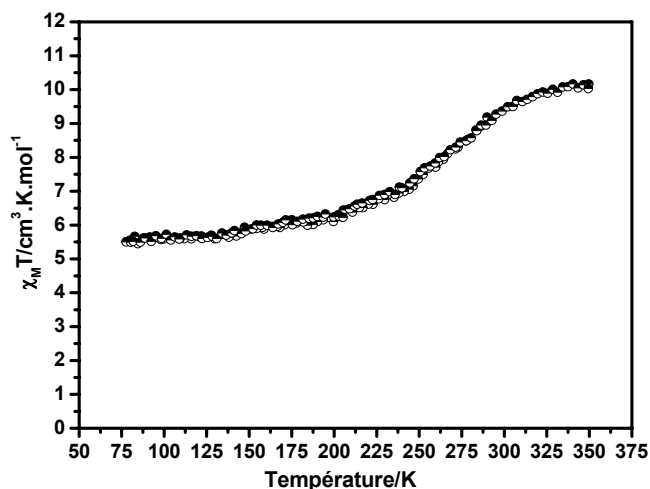
Figure II.7: Comportement magnétique du complexe trinuélaire [\text{Fe}_3\text{L}_6(\text{H}_2\text{O})_6](\text{tos})_6\cdot 4\text{H}_2\text{O} .
