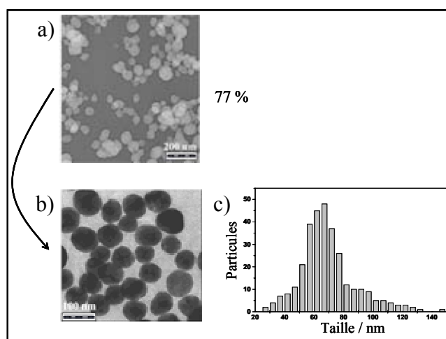
Figure IV.20: a) Image MET du lot de nanoparticules de [\text{Fe}(\text{NH}_2\text{-trz})_3](\text{Br})_2 \cdot 3\text{H}_2\text{O} \cdot [\text{ifralan}]_{0,03} préparé par voie micellaire inverse avant traitement et b) du lot après traitement (image en négatif). c) Distribution statistique évaluée sur environ 300 particules d'images MET, taille moyenne 69 nm, taille minimale et maximale, respectivement, de 26 et 147 nm, écart moyen de 15%. 243
