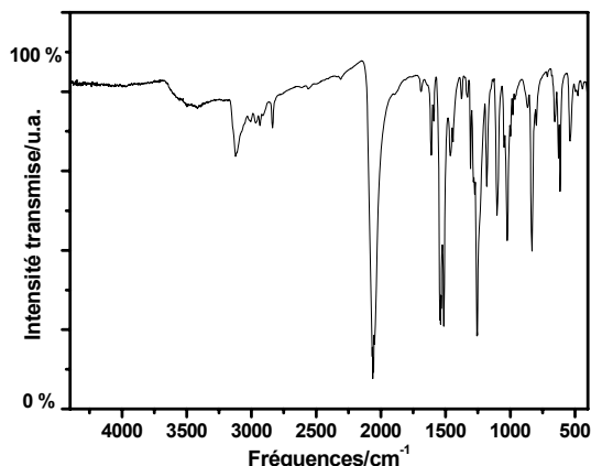
Figure II.10: Spectre IR du complexe trinuécléaire [\text{Fe}_3\text{L}_6(\text{NCS})_4(\text{H}_2\text{O})_2]\text{Br}.\text{(NCS)} .
