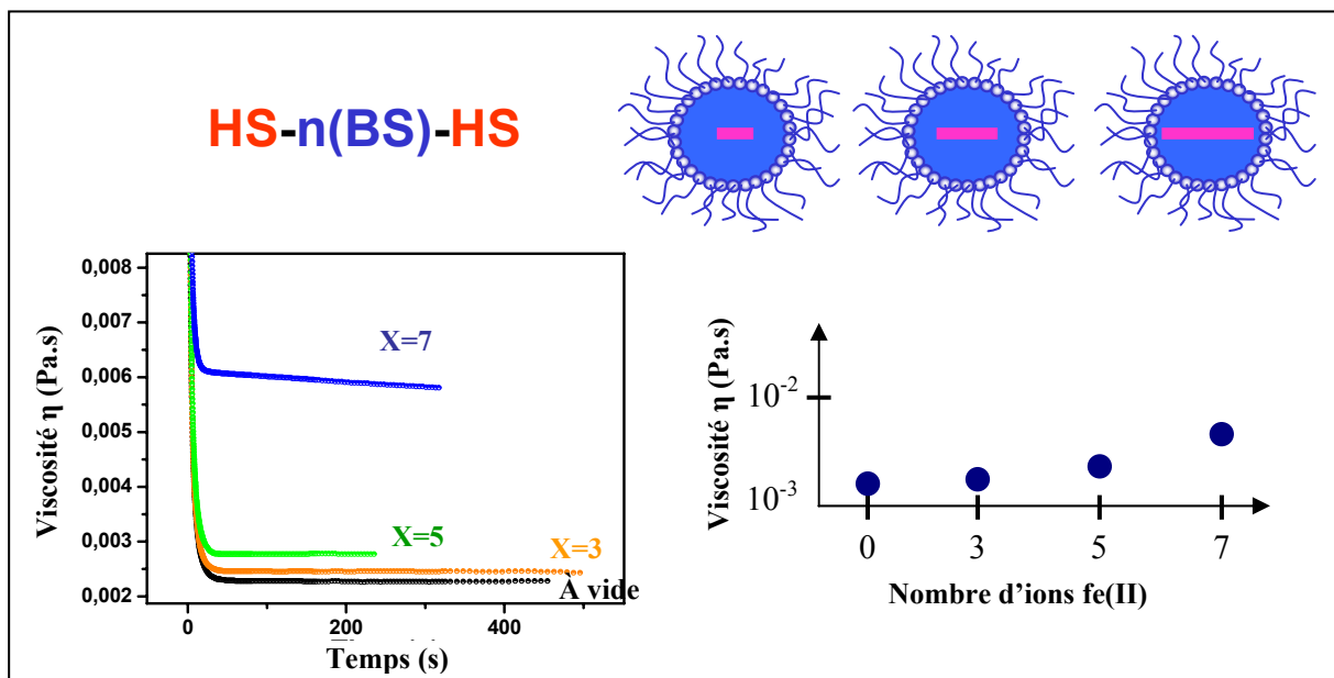
Figure III.11: Etude de viscosité des différents systèmes micellaires contenant les oligomères insaturés.
