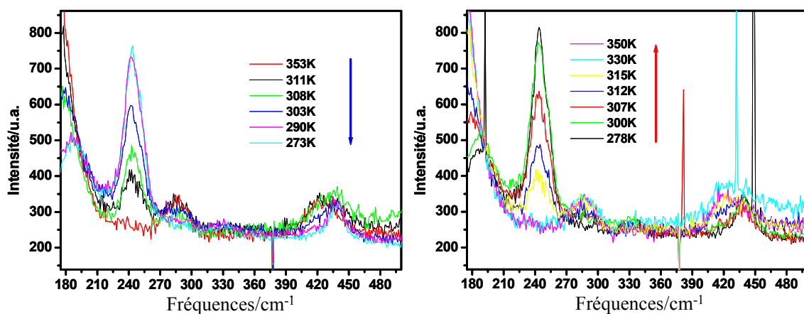
Figure IV.22: Etude Raman en température du lot issu d'une synthèse à 77 % de tensioactif (laser Ar + à 514,5 nm et à 8,1 mW/cm 2 ). Expériences réalisées dans l'équipe du Pr. K. Tanaka (Kyoto, Japon).
