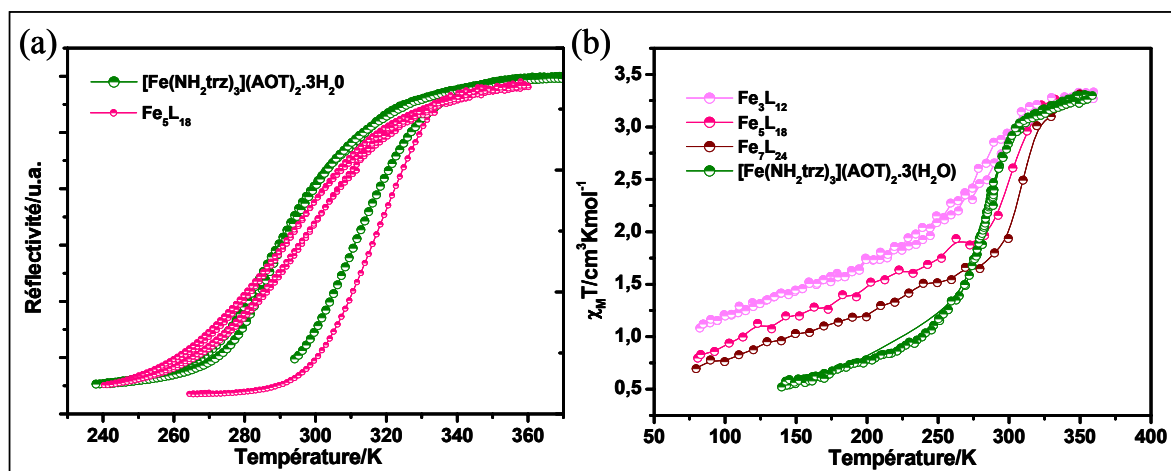
Figure III.23: (a) Superposition normalisée des spectres de réflectivité du composé traditionnel et du \text{Fe}_5\text{L}_{18} . (b) Courbe de magnétisme des différents oligomères saturés et du complexe traditionnel.
