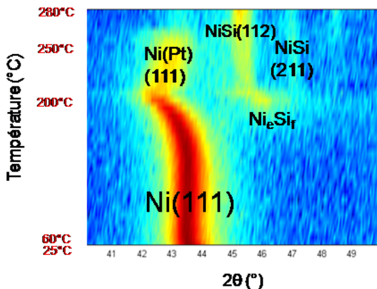
Figure 9 : Diagrammes de DRX in situ en géométrie Bragg-Brentano ( \lambda=1.54\text{\AA} ) réalisés sur 50nm de \text{Ni(13\%Pt)/Si(100)} par étape
