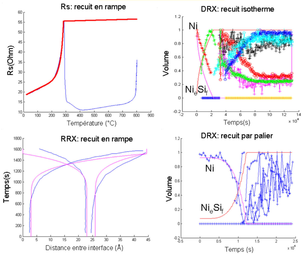
Figure 5 : Simulation de la croissance de la 1 ère phase des expériences réalisées sur des échantillons codéposés de Ni(25nm, 13%Pt) : DRX, RRX, Rs.
