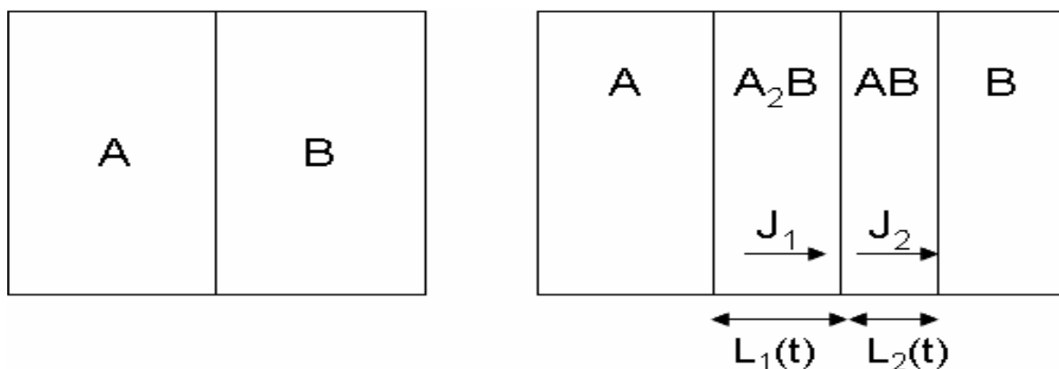
Figure 10 : Représentation schématique de la croissance simultanée de deux phases \text{A}_2\text{B} et AB par réaction à l'état solide entre deux éléments A et B.
