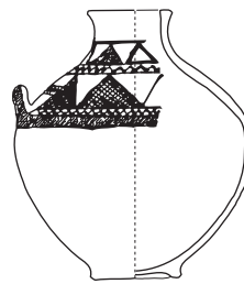
Hama, période I (1200 - 1075) Jarre à une anse de G IV 19 (5A 922). 1:10 Riis, p. 54, fig. 41
