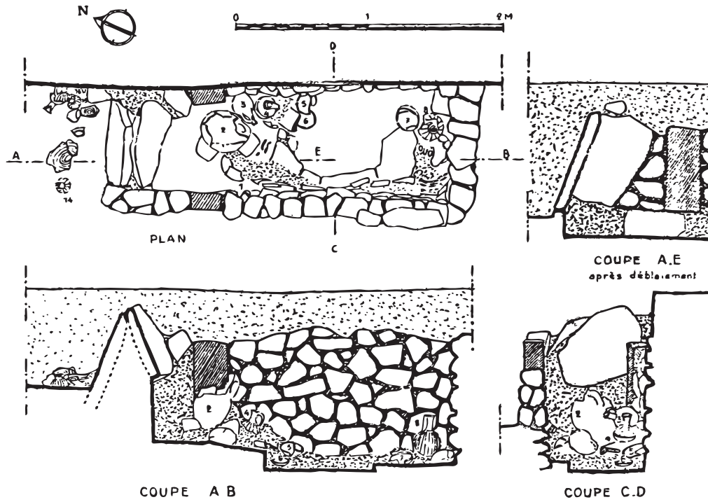
Fig. 87. — Enkomi (1947). Plan et coupes de la tombe 1. Chypriote Fer I. (Cf. § 77).
