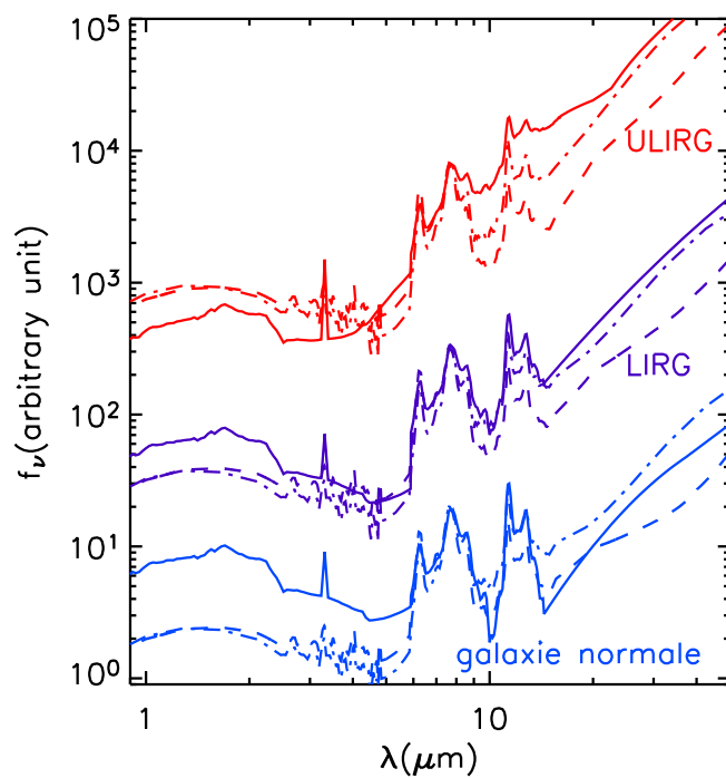
FIG. 4.8 – Comparaison des distributions spectrales d'énergie d'une galaxie normale ( L_{IR} \sim 10^{10} L_\odot ), d'une LIRG ( L_{IR} \sim 5 \times 10^{11} L_\odot ), d'une ULIRG ( L_{IR} \sim 5 \times 10^{12} L_\odot ). trait plein : CE, pointillés : LDP, pointillés-points : DH.
