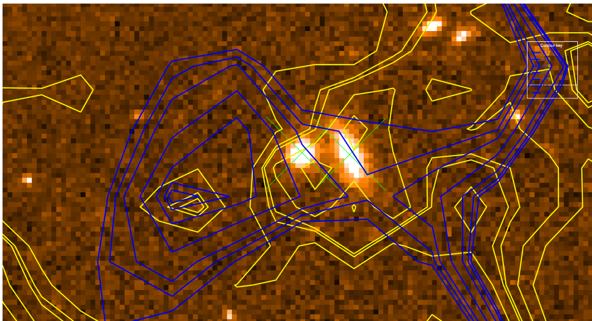
FIG. 5.5 – Source détectée à 15 \mu\text{m} par ISOCAM (contours bleus), à 24 \mu\text{m} par MIPS (contours jaunes), à 1.4 \text{ GHz} (carré rouge), à 8.5 \text{ GHz} (rond rouge). Les croix vertes sont associées à des sources qui ont un redshift spectroscopique. L'image a une taille de 11' \times 7' .
