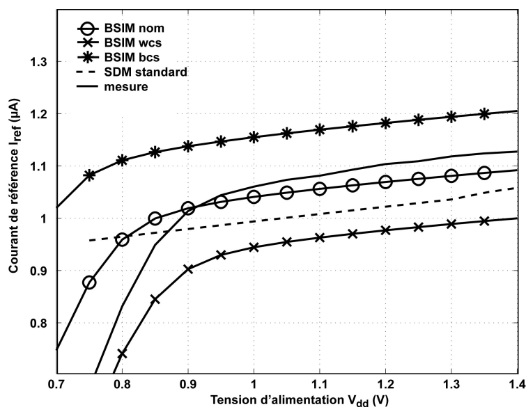
Fig. IV.23 – Caractéristique simulée en modèle standard de la référence de courant Camacho-Galeano 1uA
