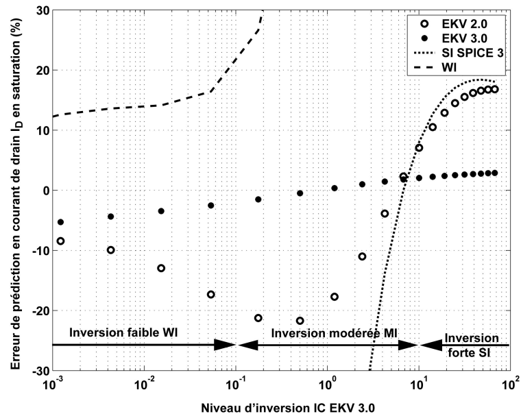
Fig. II.9 – Comparaison du courant de drain en saturation des différents noyaux avec le modèle de feuille de charge.
