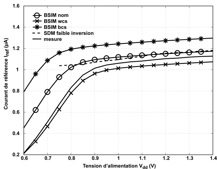
Fig. IV.27 – Caractéristique mesurée et simulée en modèle faible inversion de la référence de courant Camacho-Galeano 1 \mu A
