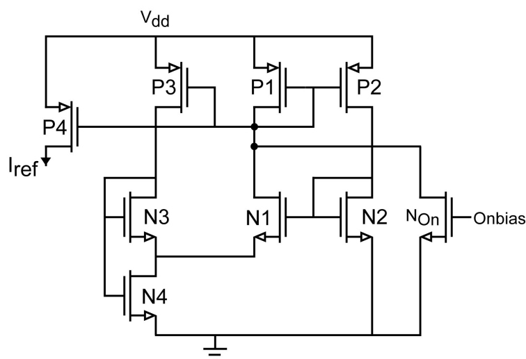
Fig. IV.20 – Schéma de la référence de courant Camacho-Galeano
