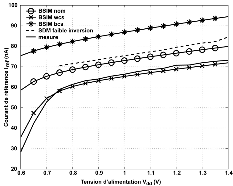
Fig. IV.17 – Caractéristique mesurée et simulée en modèle faible inversion de la référence de courant Oguey 50nA
