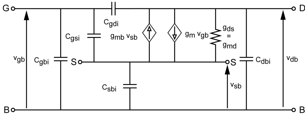
Fig. II.7 – Schéma petit signal du transistor MOS
