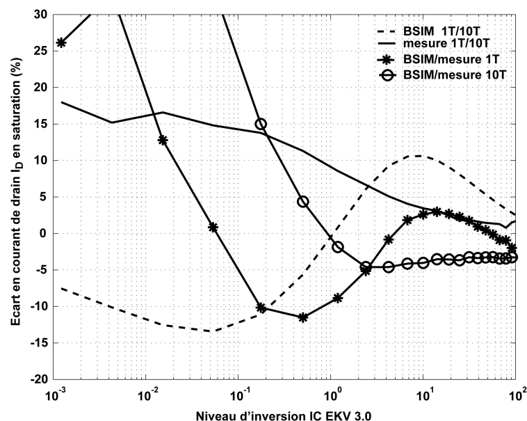
Fig. III.34 – Comparaison du courant de drain en saturation à grande longueur de grille
