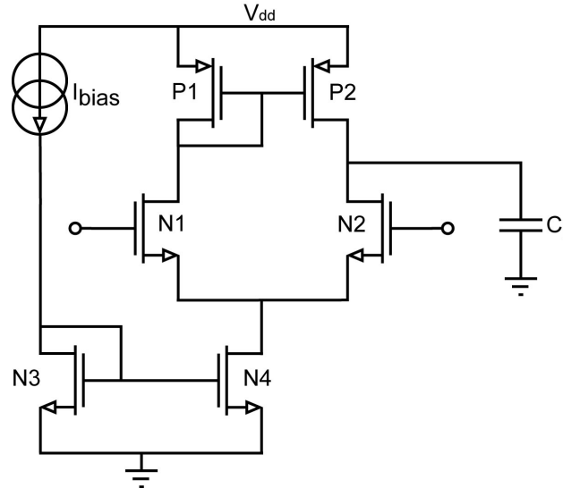
Fig. A.1 – Schéma de l'OTA charge miroir
