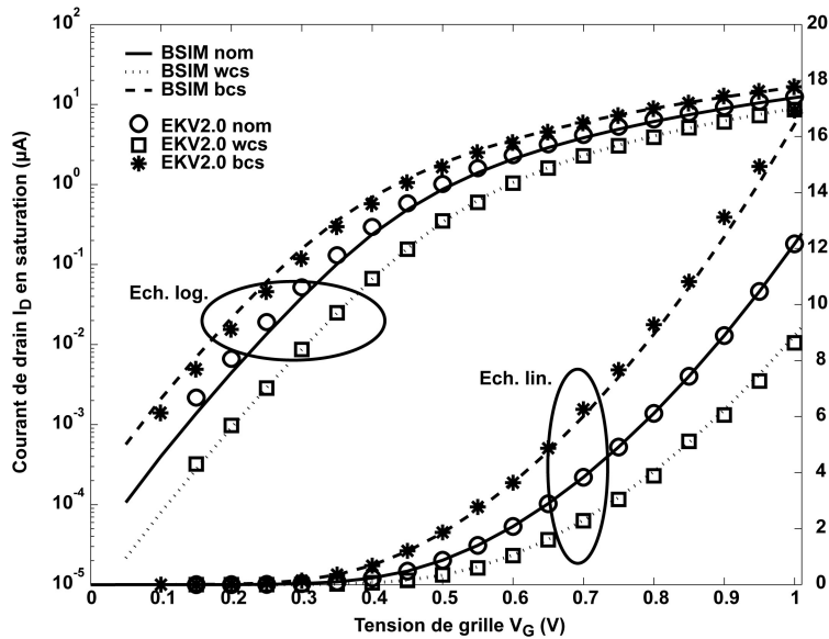
Fig. III.36 – Prédiction du drain en saturation
