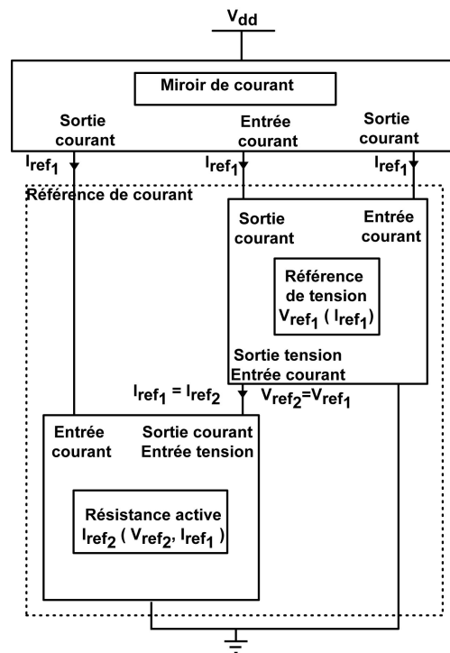
Fig. III.7 – Principe des références de courant autopolarisées à résistance active
