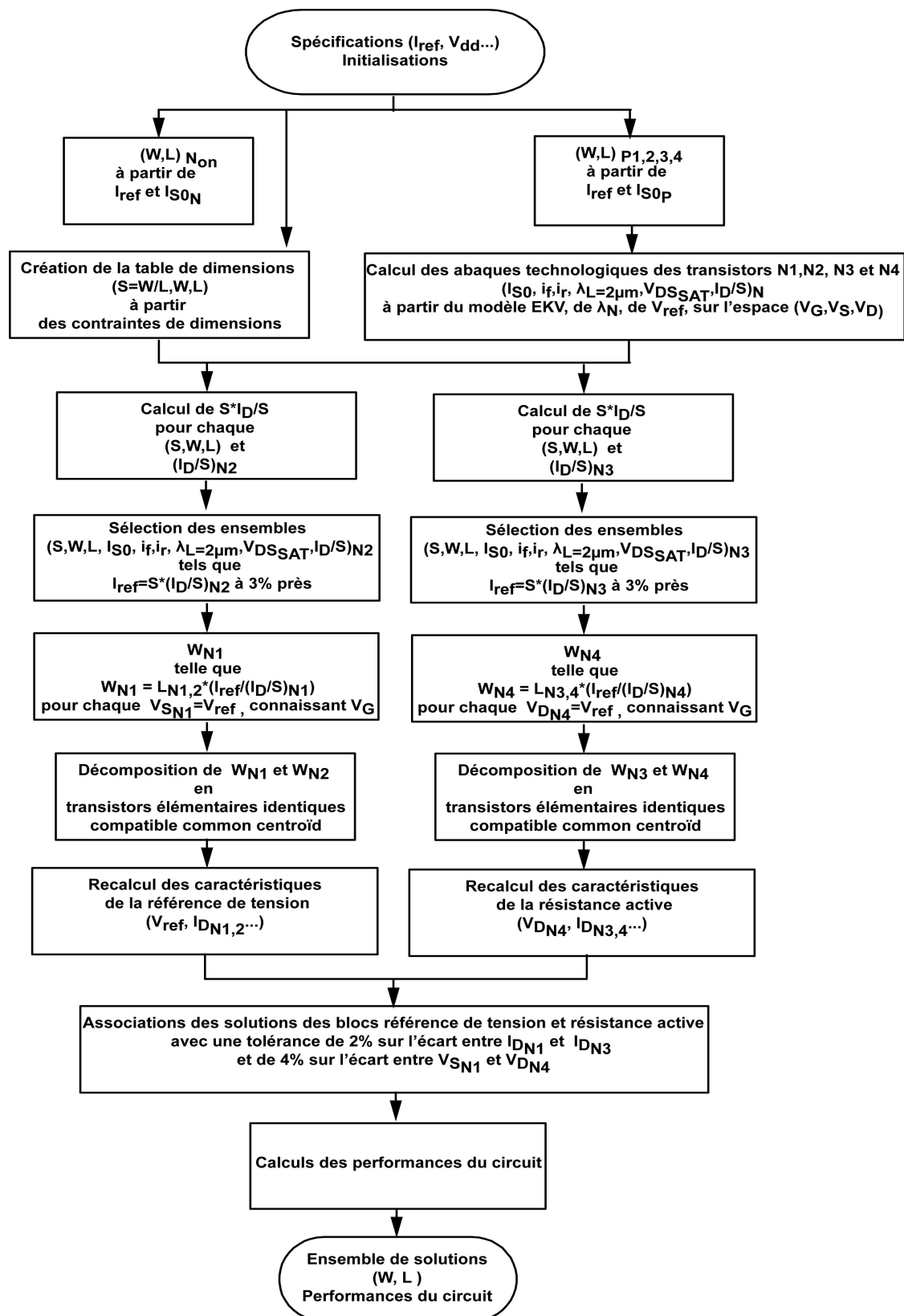
Fig. IV.11 – Plan de conception de la référence de courant Oguey
