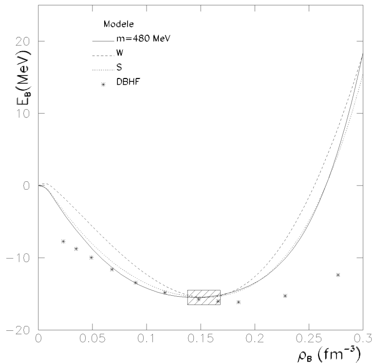
Figure 5.4 - Energie de liaison E_B en fonction de la densité baryonique \rho_B pour : notre modèle avec m = 480 MeV (ligne pleine), le modèle de Walecka W (ligne tiretée), le modèle de Song S (ligne pointillée) et le résultat du calcul DBHF-BonnA (étoiles). La zone hachurée représente la zone empirique du point de saturation.
