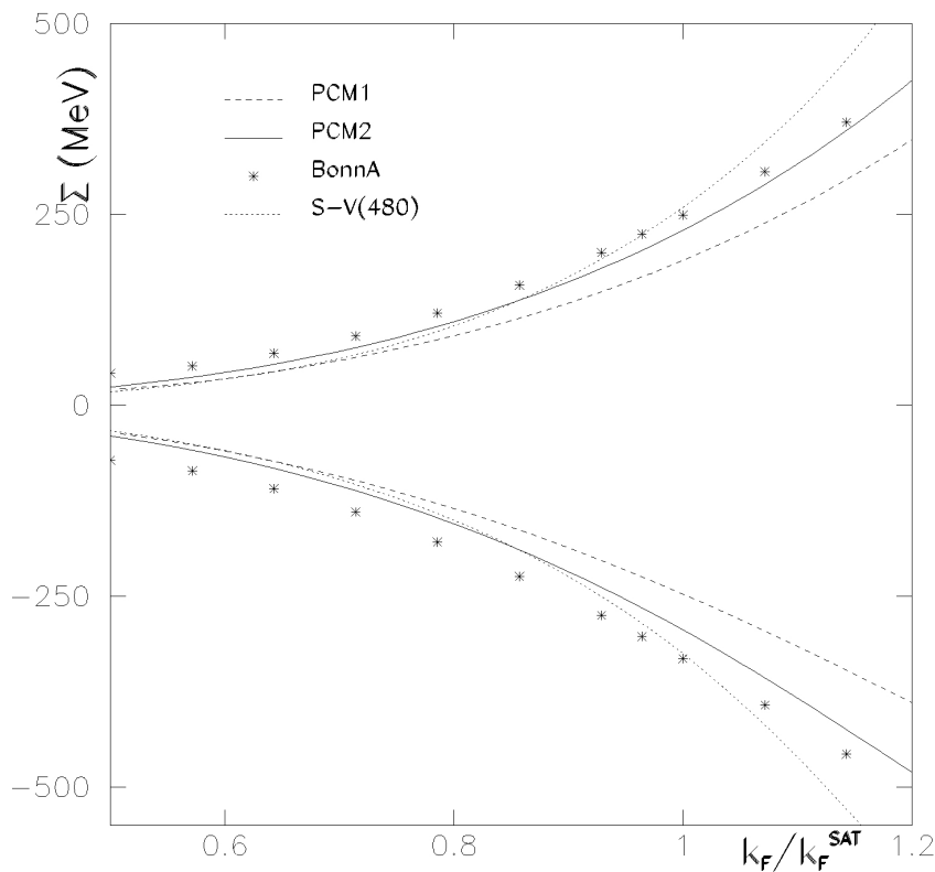
Figure 8.7 - Self-énergies du nucléon en fonction du moment de Fermi normalisé k_F/k_F^{\text{sat}} pour les paramétrisations pcm1 (ligne tiretée) et pcm2 (ligne pleine), le modèle S-V(480) (ligne pointillée) et un calcul DBHF basé sur un potentiel Bonn A (étoiles).
