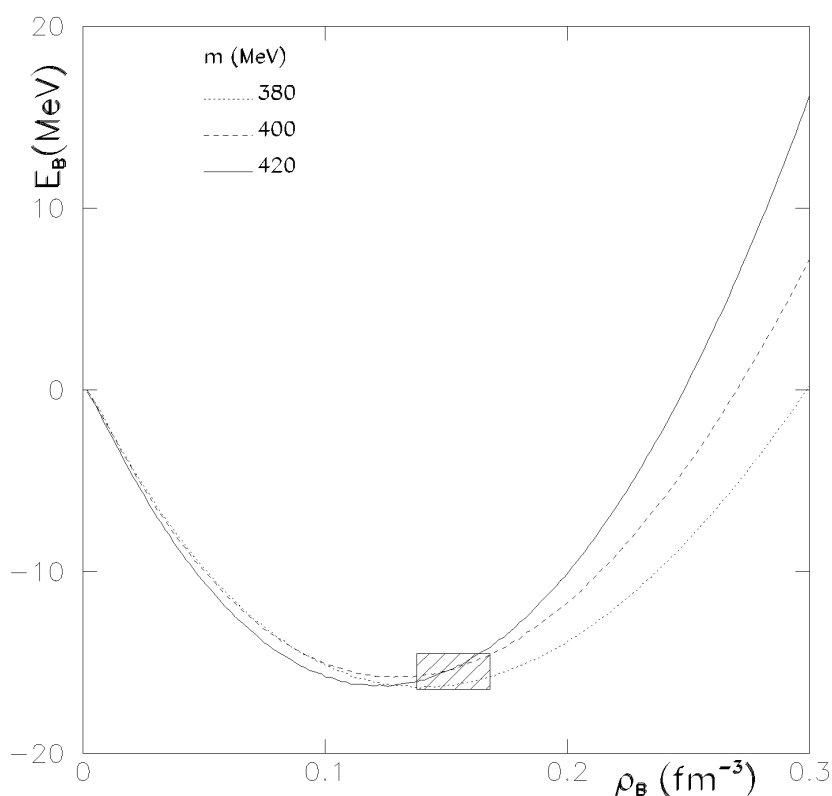
Figure 8.2 - Énergie de liaison E_B en fonction de la densité baryonique \rho_B pour trois valeurs de la masse du quark dans le vide : m = 380 MeV (ligne pointillée), m = 400 MeV (ligne tiretée) et m = 420 MeV (ligne pleine). La zone hachurée représente la zone empirique du point de saturation.
