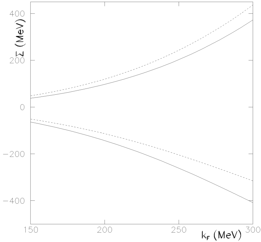
Figure 8.4 - Self-énergies en fonction de k_F aux différentes étapes du calcul : contributions de NJL + échanges de pions (ligne tiretée) et self-énergies avec la correction en k_F^3 (ligne pleine).
