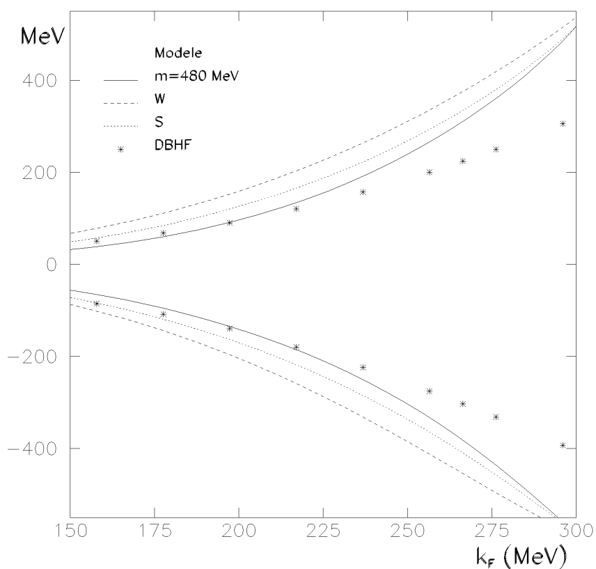
Figure 5.5 - Self-énergies du nucléon en fonction du moment de Fermi k_F pour : notre modèle avec m = 480 MeV (ligne pleine), le modèle de Walecka W (ligne tiretée), le modèle de Song S (ligne pointillée) et le résultat du calcul DBHF-BonnA (étoiles).
