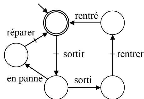
Figure 2.8 : assemblage du modèle de comportement du vérin
