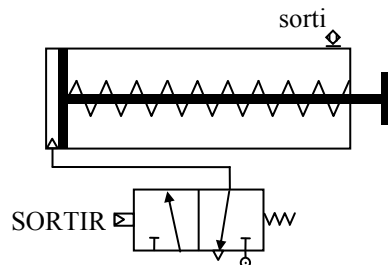
Figure 4.13 : chaîne fonctionnelle « vérin pneumatique avec distributeur monostable et un capteur de fin de course »
