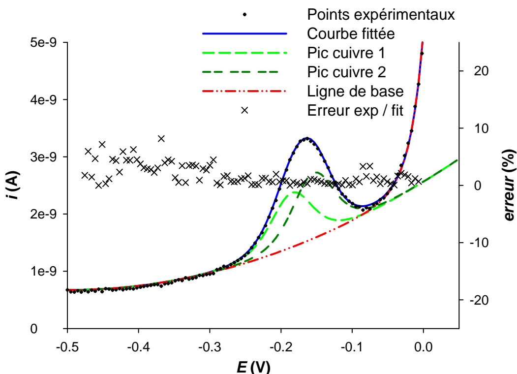
Figure II-11 : Exemple de déconvolution d'un voltammogramme afin d'en extraire l'aire du ou des pics caractéristiques de l'espèce étudiée. Exemple avec 2 pics de cuivre
