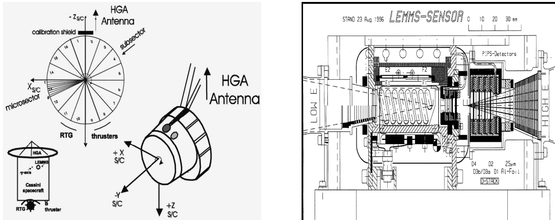
FIG. 2.3 – A gauche : Géométrie et position de l'instrument MIMI/LEMMS dans le repère de la sonde ( x_{SC}, y_{SC}, z_{SC} ). La direction de l'antenne grand gain ( HGA ), des générateurs radioactifs thermiques ( RTG ), des propulseurs ( thrusters ), obscurcissent en partie le champ de vue de l'instrument (Krimigis et al., 2004). A droite : Configuration du détecteur MIMI/LEMMS. Les particules de basse énergie entrant dans la partie basse énergie ( LOW E ) sont enregistrées au niveau des détecteurs E et F (pour les électrons) et A et B (pour les ions). La partie haute énergie ( HIGH E ) mesure les particules via les détecteurs D.
