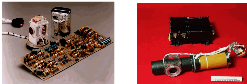
FIG. 2.10 – A gauche : Le magnétomètre à saturation de flux FGM. A droite : Le magnétomètre à hélium à mode scalaire/vectériel VSHM (Dougherty et al., 2004).
