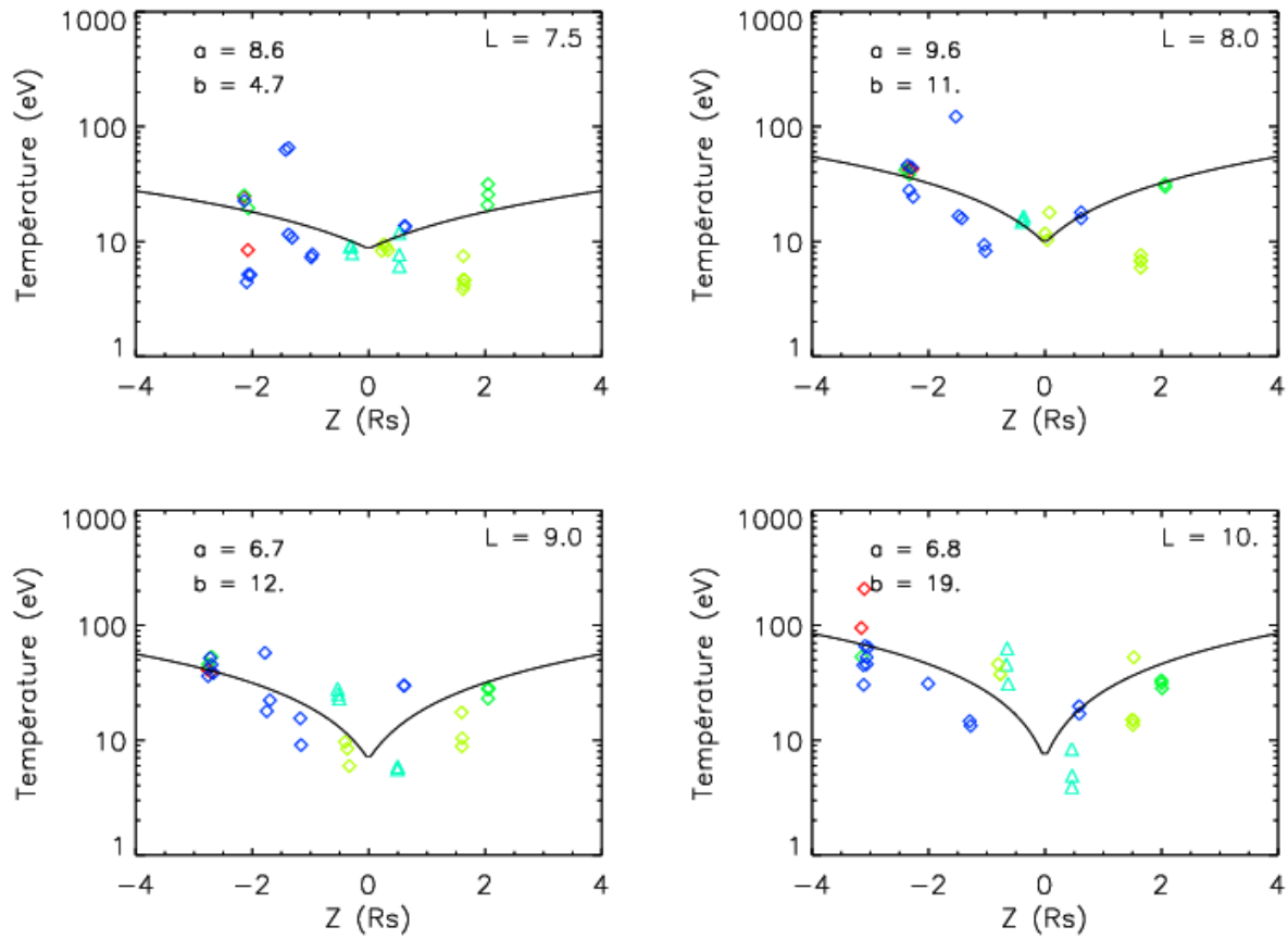
FIG. 3.48 – Profil de la température de la population thermique en fonction de l'altitude z (repère équatorial) à différents Lshell. Pour chacun des profils en altitude, nous avons ajusté un modèle empirique du type T_{e_{th}} = a + bZ . A L=7.5 : (a,b)=(8.6,4.7) . A L=8 : (a,b)=(9.6,11.2) . A L=9 : (a,b)=(6.7,12.3) . A L=10 : (a,b)=(6.8,19) .
