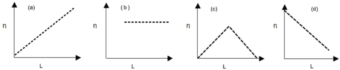
FIG. 4.1 – Profils radiaux types du contenu du tube de flux du plasma dans une magnétosphère. (a) le profil est ascendant vers l’extérieur, ce qui signifie une source externe et une perte vers l’intérieur. (b) le profil est constant, le transport du plasma est exempt de source et de perte. (c) le profil maximise à un L intermédiaire, signifiant à cette région. (d) le profil est descendant, signifiant à cette région une source interne associée à un transport avec pertes vers l’extérieur.
