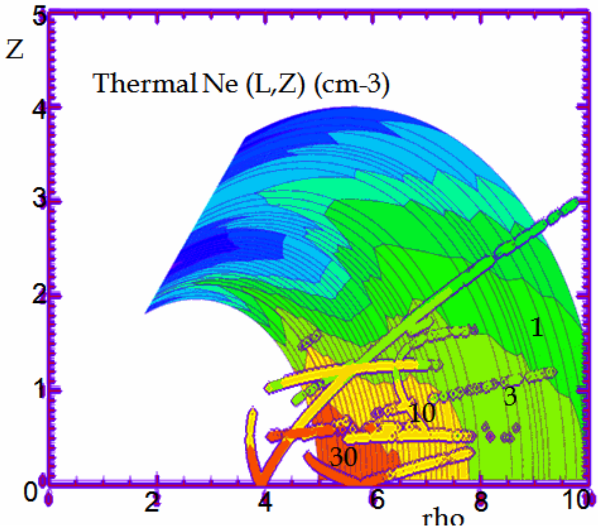
FIG. 3.51 – Cartographie dans le plan (\rho, z) de la densité des électrons thermiques dans la magnétosphère interne de Saturne (région 1) à partir de notre modèle d'équilibre diffusif. Les densités obtenues par Persoon et al. (2005) le long de quelques orbites de Cassini sont superposées à notre carte.
