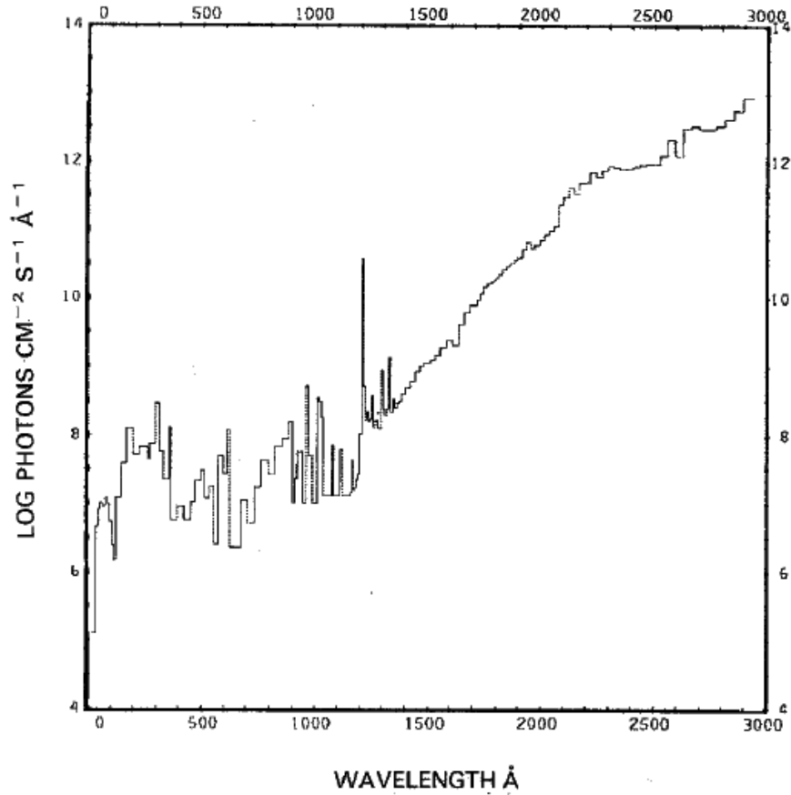
FIG. 3.9 – Spectre du flux solaire ( cm^{-2}s^{-1} ) à une distance d'1 Unité Astronomique en fonction de la longueur d'onde (en Angström ) (Huebner et al., 1992).
