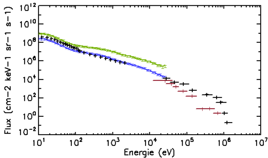
FIG. 2.17 – Flux composite à 15 min de résolution des instruments PLS-LECP de Voyager (en noir) et des instruments CAPS/ELS-MIMI/LEMMS de Cassini (en bleu : flux calculés sur base des nouveaux facteurs géométriques, en vert : flux calculés sur base des anciens facteurs géométriques, en rouge : flux de MIMI/LEMMS).
