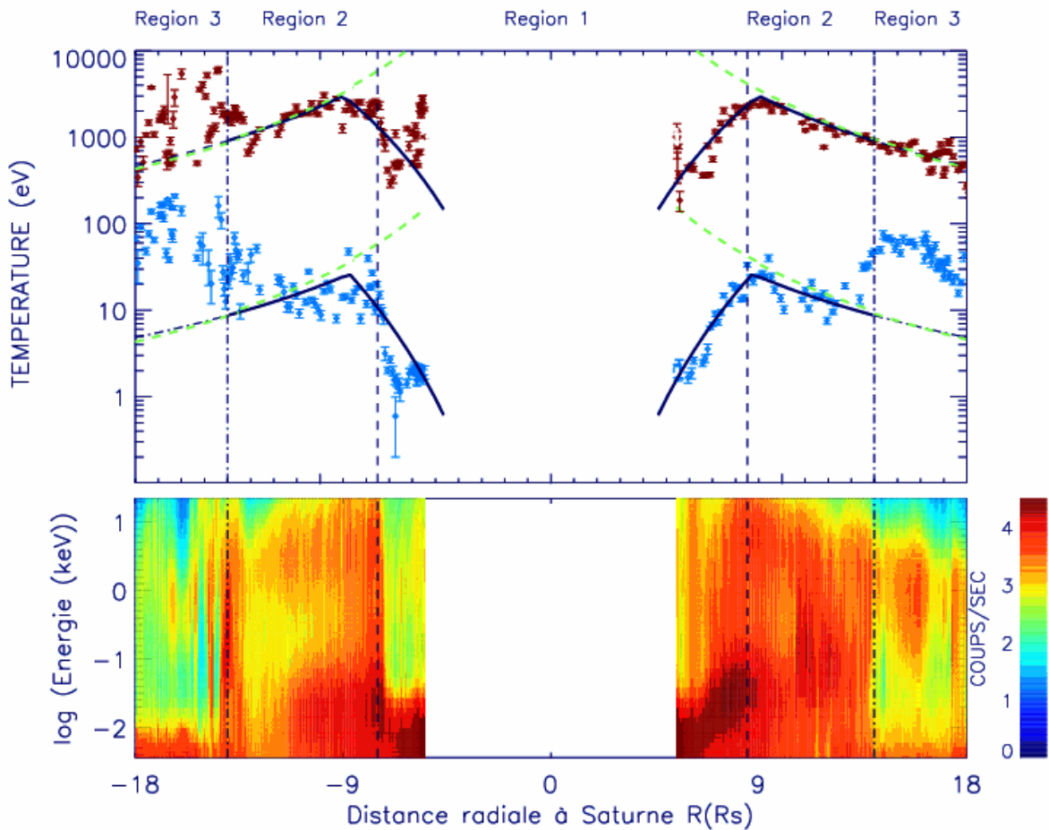
FIG. 3.17 – Haut : Profil radial de température des populations thermique T_{eth} (en bleu) et suprathermique T_{esth} (en rouge), orbite rev 24. Les modèles en loi de puissance aL^n sont ajustés aux profils dans les régions magnétosphériques 1 et 2. Bas : Spectrogramme de CAPS/ELS.
