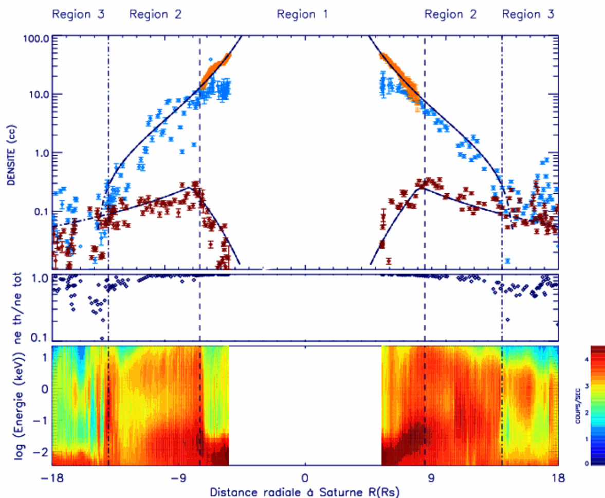
FIG. 3.16 – Haut : Profil radial de densité des populations thermique ne_{th} (en bleu), suprathermique ne_{sth} (en rouge), ainsi que les données densité ne_{fUH} déduites de la fréquence hybride haute (en orange), orbite rev 24. Les modèles en loi de puissance aL^n sont ajustés aux profils dans les régions magnétosphériques 1 et 2 (en traits pleins). Milieu : Profil radial du rapport de la densité de la population thermique et de la densité totale ( f_{UH} ). Bas : Spectrogramme de CAPS/ELS, pour référence.
