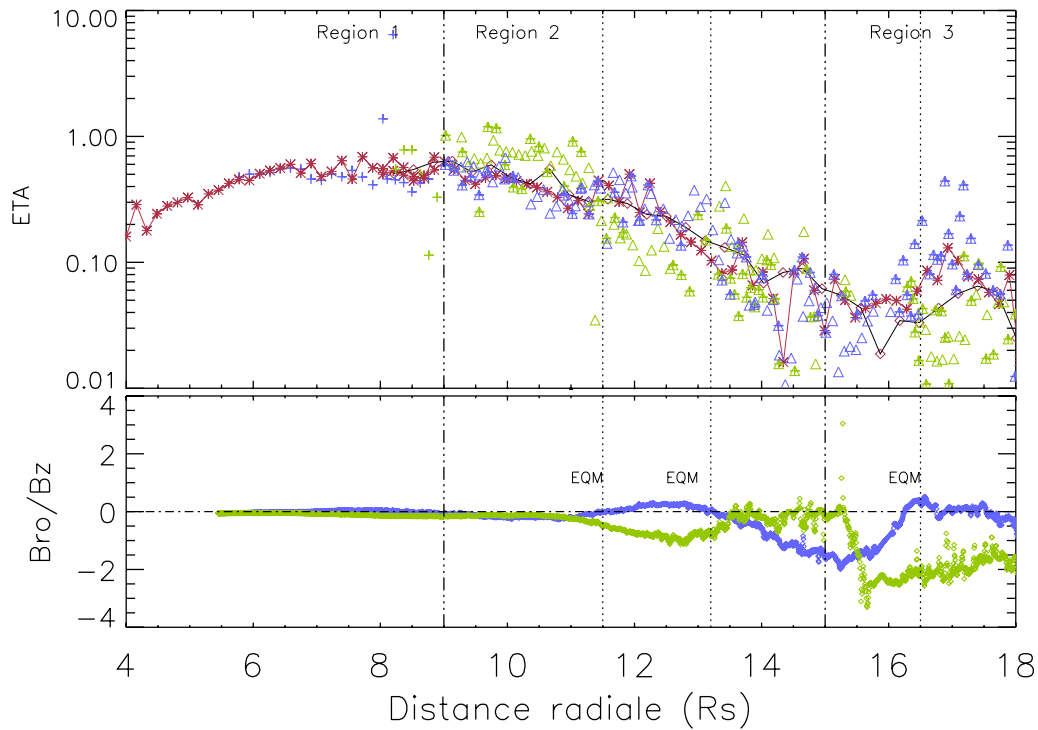
FIG. 4.14 – Haut : Profil du contenu du tube de flux approché de la population thermique dans la magnétosphère. Les données de la partie entrante de l'orbite sont en vert, les données de la partie sortante en bleu. Le modèle moyen est superposé en rouge. Les frontières à 9 R_S et 15 R_S sont superposées en traits discontinus, ainsi que les passages à l'équateur magnétique (notés EQM). Bas : Profil du paramètre R_{B(z,\rho)} = B_{\rho}/B_z .
