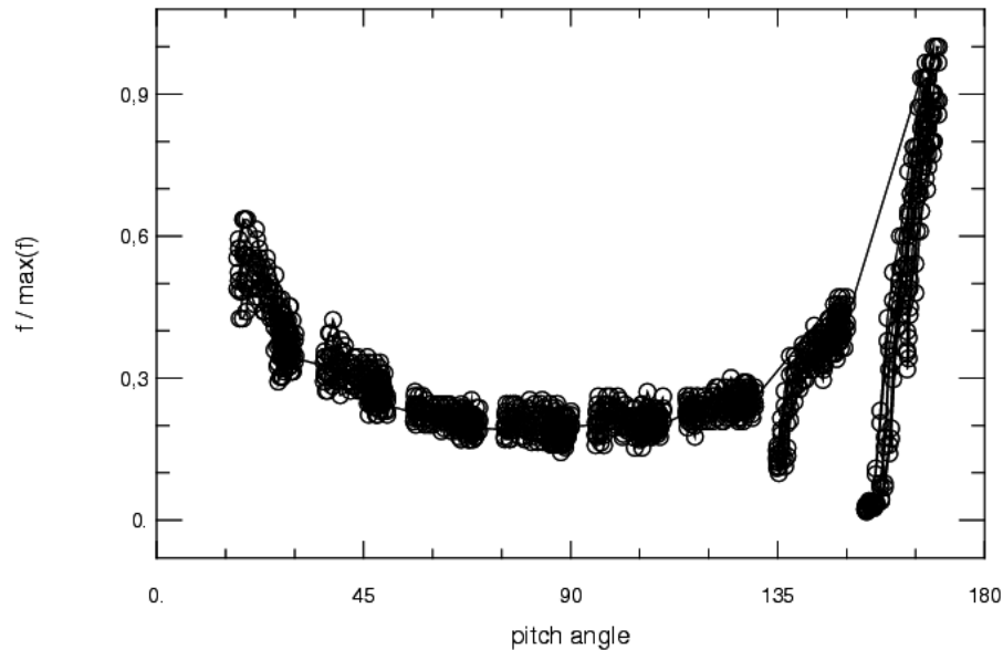
FIG. 4.9 – Distribution en angle d’attaques normalisée par rapport aux maximum local, à une énergie de 500 eV (CAPS/ELS), orbite REV 24, Jour 143 de l’année 2006 à 14H44, R = 15.5 R_S . La distribution apparaît comme la superposition d’une distribution isotrope et d’une distribution alignée au champ magnétique.
