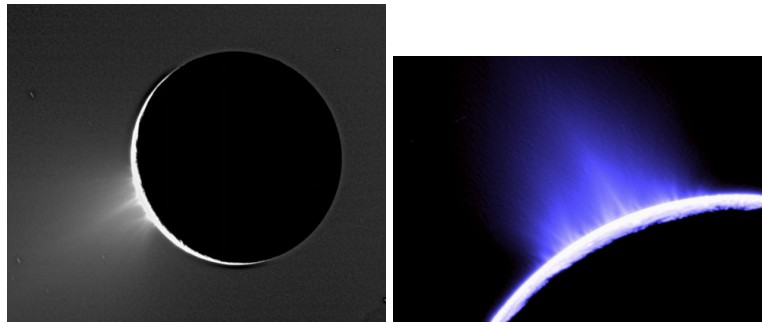
FIG. 1.25 – Geysier de particules de glace et de vapeur d'eau éjectés depuis le pôle sud du satellite Encelade photographié par la caméra ISS (Cassini) le 5 décembre 2005 (Image NASA/ESA).
