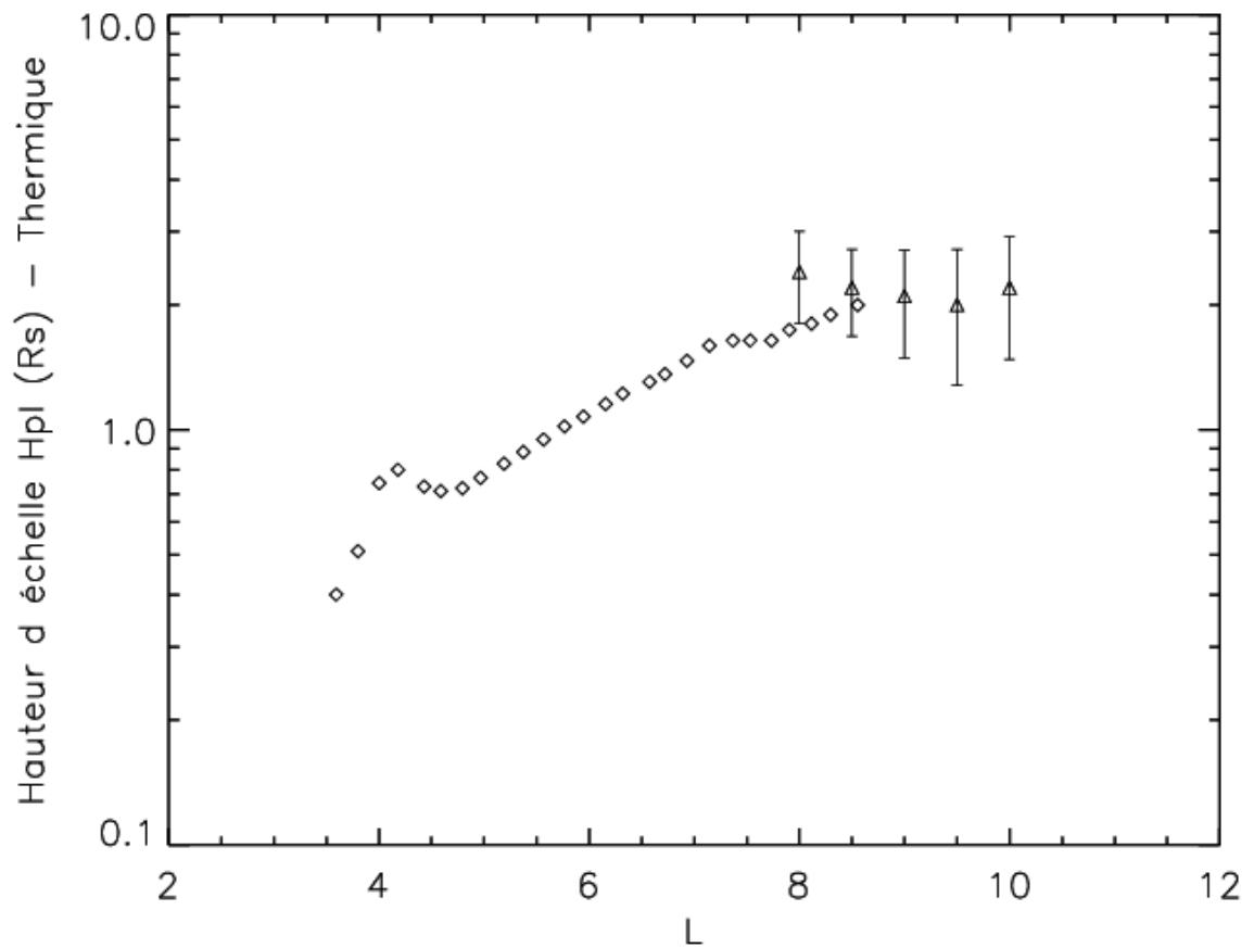
FIG. 3.47 – Echelle de hauteur de la couche de la population d'électrons thermiques de (Persoon et al., 2006) (en losanges), et échelle de hauteur que nous avons déduit de notre analyse au-delà de 8 R_S (en triangles).
