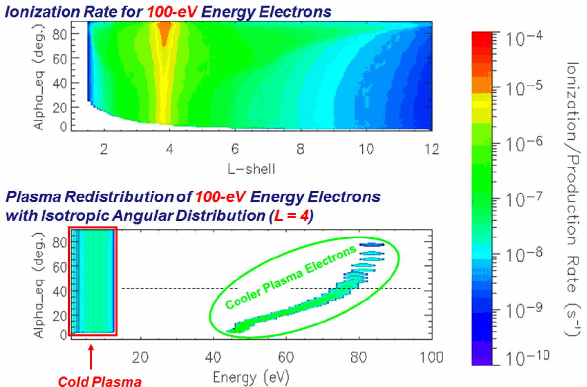
FIG. 4.17 – Haut : Simulation du taux d’ionisation d’un électron d’énergie incidente de 100 eV en fonction de la distance radiale et de l’angle d’attaque à l’équateur (Santos-Costa et al. (2007)). Bas : Simulation de la distribution émergente des électrons suite à l’impact électronique de l’électron à 100 eV dans un nuage de neutres à L=4 Santos-Costa et al. (2007). Le modèle de tore de neutres utilisé est celui de Johnson et al. (2006).
