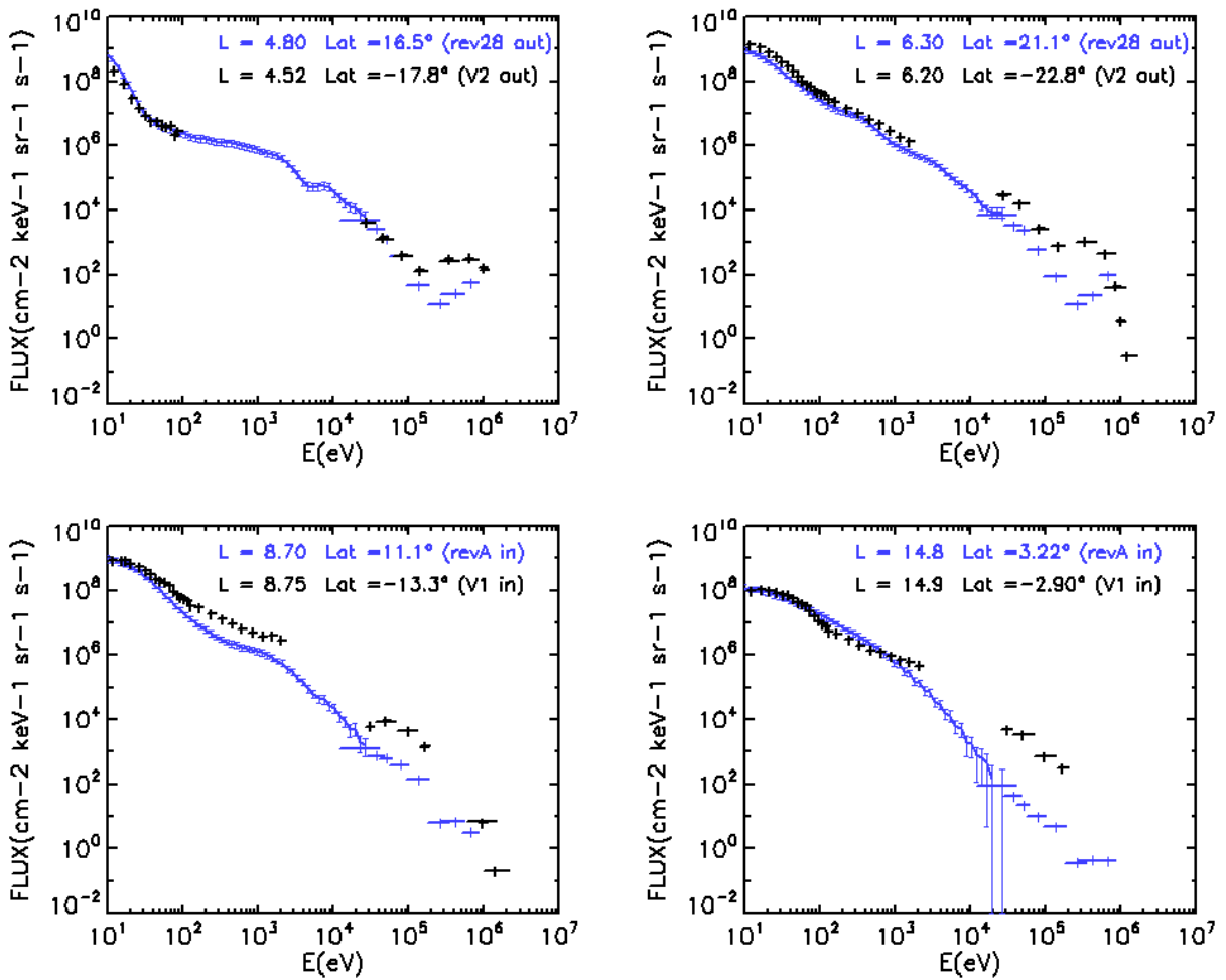
FIG. 2.18 – Flux composites des instruments PLS-LECP de Voyager (en noir) et des instruments CAPS/ELS-MIMI/LEMMS de Cassini (en bleu), pour différentes distances radiales.
