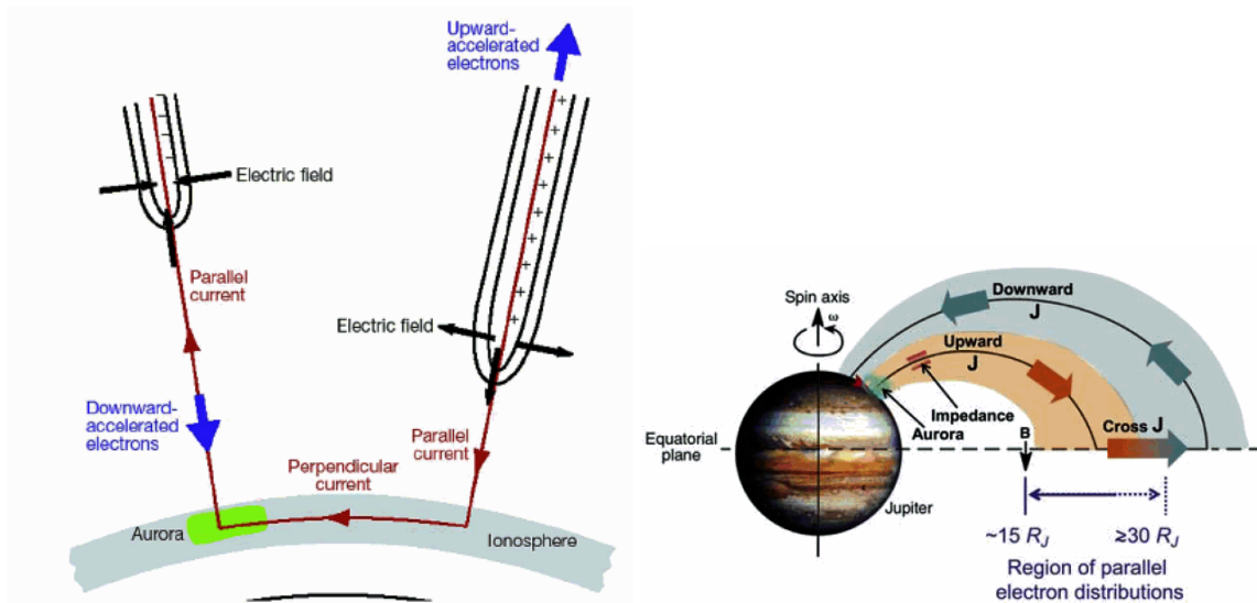
FIG. 1.16 – A gauche : les courants alignés à l’ionosphère terrestre par Mauk & Saur (2007). A droite : Représentation du couplage ionosphère-magnétosphère dans la magnétosphère joviennne. Les courants alignés forcent la magnétosphère à tourner en corotation avec l’ionosphère. Les courants alignés se referment au niveau de l’équateur magnétique et ionosphérique par des courants perpendiculaires j_{\perp} . Ils se composent d’une zone de courant alignée upward , associée aux électrons downward , et d’une zone de courant downward associée à des électrons upward .
