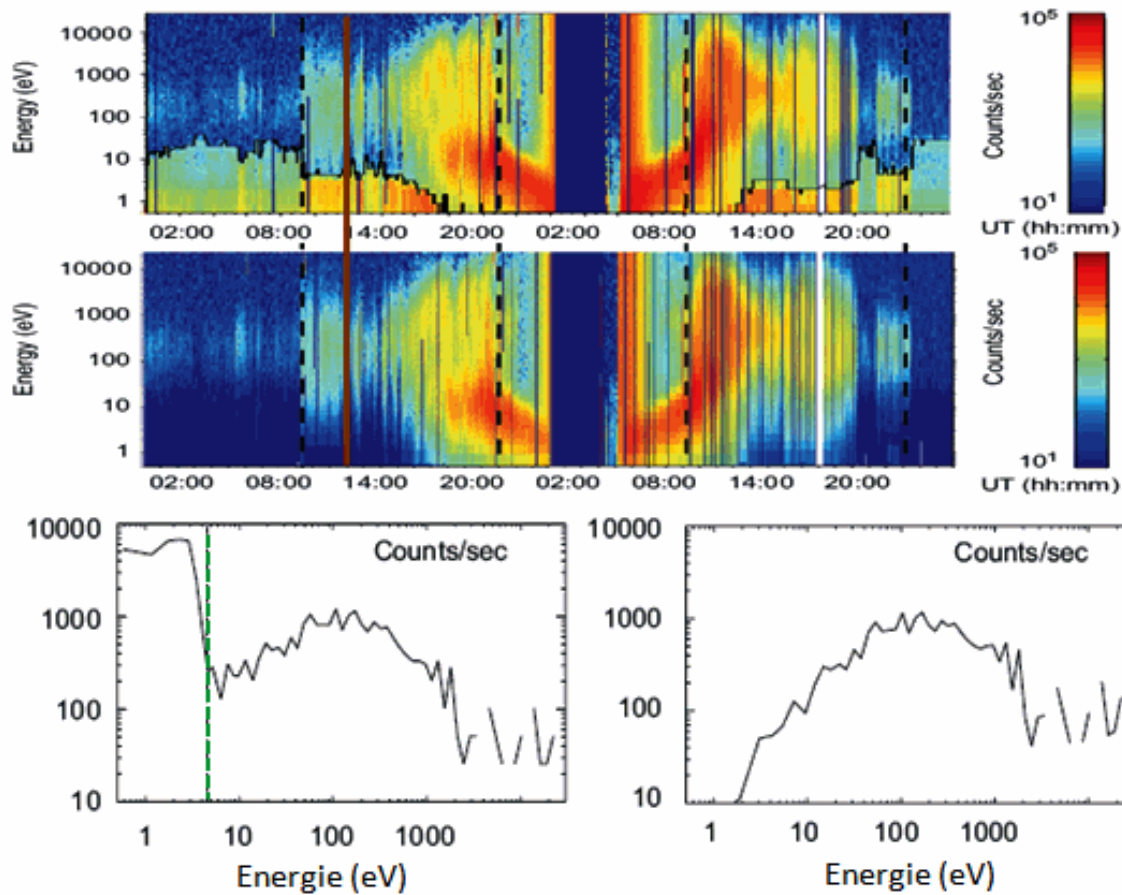
FIG. 2.13 – En haut : Spectrogramme de CAPS/ELS en coups/sec enregistré lors de l'orbite SOI non corrigé du potentiel photoélectrique du satellite. Milieu : Même spectrogramme corrigé du potentiel photoélectrique de satellite. En bas : Coupe du spectrogramme le jour 182 à 12h30 UT (trait vertical brun sur le spectrogramme), non corrigé (à gauche) et corrigé de l'effet du potentiel (à droite) (Lewis et al., 2008). Le trait vertical vert correspond à la valeur du potentiel photoélectrique. A gauche de ce trait, nous observons le spectre des photoélectrons 'artificiels'.
