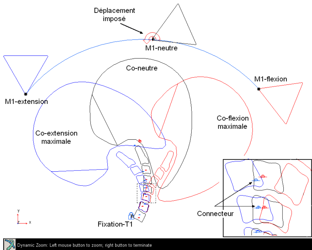
Figure 2.17: Modèle ostéo-articulaire de corps rigides (Msc.Adams)
