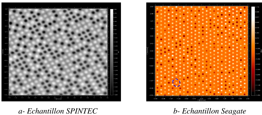
Figure.2: Images MFM, (a) 3x3 \mu\text{m}^2 d'une multicouche de \text{Pt}_{15}/(\text{Co}_{0.6}/\text{Pt}_{1.8})_4 déposée sur un réseau de plots carrés de 80x80nm 2 espacés de 65nm. (b) 5x5 \mu\text{m}^2 de plots circulaires de 100nm de diamètre espacés de 100nm et répartis en pistes circulaires dans une géométrie hexagonale gravés dans une couche de CoCrPt.
