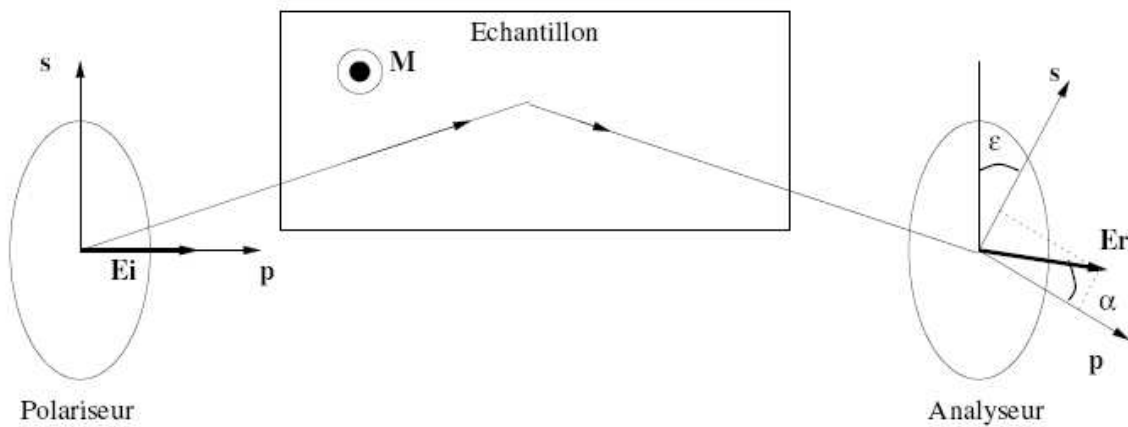
Figure.2 : Chemin parcouru par une onde lumineuse en réflexion sur un échantillon. Le polariseur permet d'aligner \mathbf{E} selon (O,p). L'analyseur sélectionne les composantes (O,p) et (O,s). La désorientation entre le polariseur et l'analyseur permet de dissymétriser le signal magnétique.
