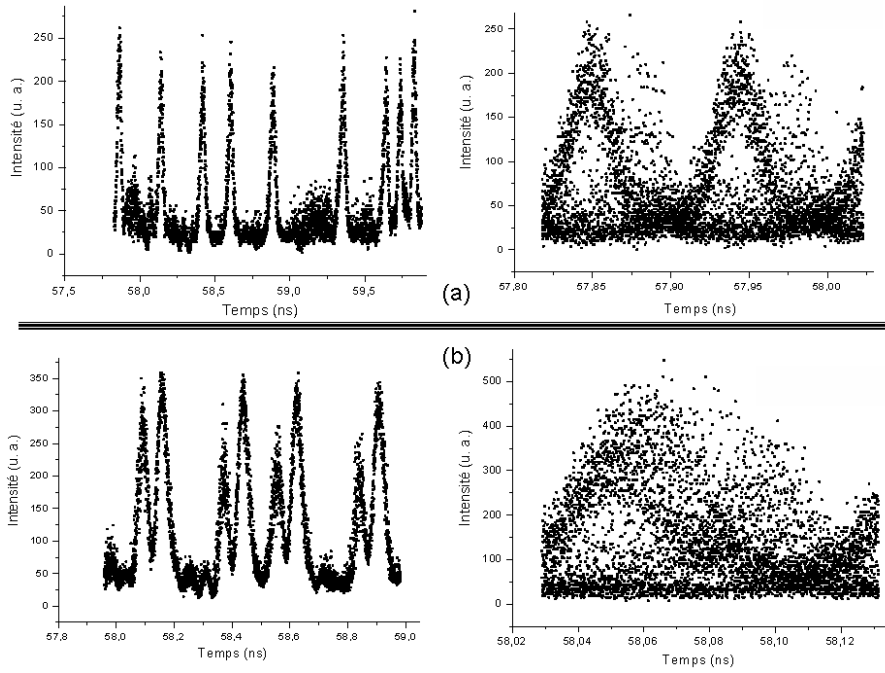
Figure 5.19 : Etude expérimentale de l'impact du paramètre \Delta T sur la sortie transmission du NOLM-SOA du point de vue de la séquence (à gauche) et du diagramme de l'œil correspondant (à droite).
