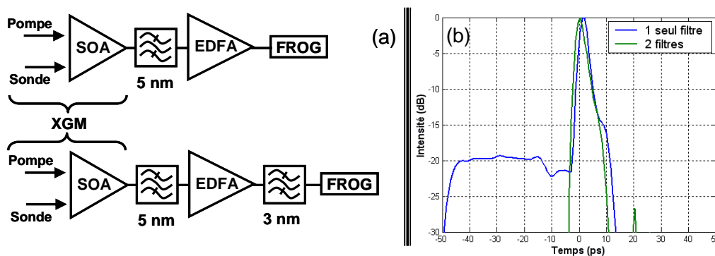
Figure 6.30 : Impact de l'introduction d'un second filtre. (a) : Schémas de montages ; (b) : Caractérisation au FROG.
