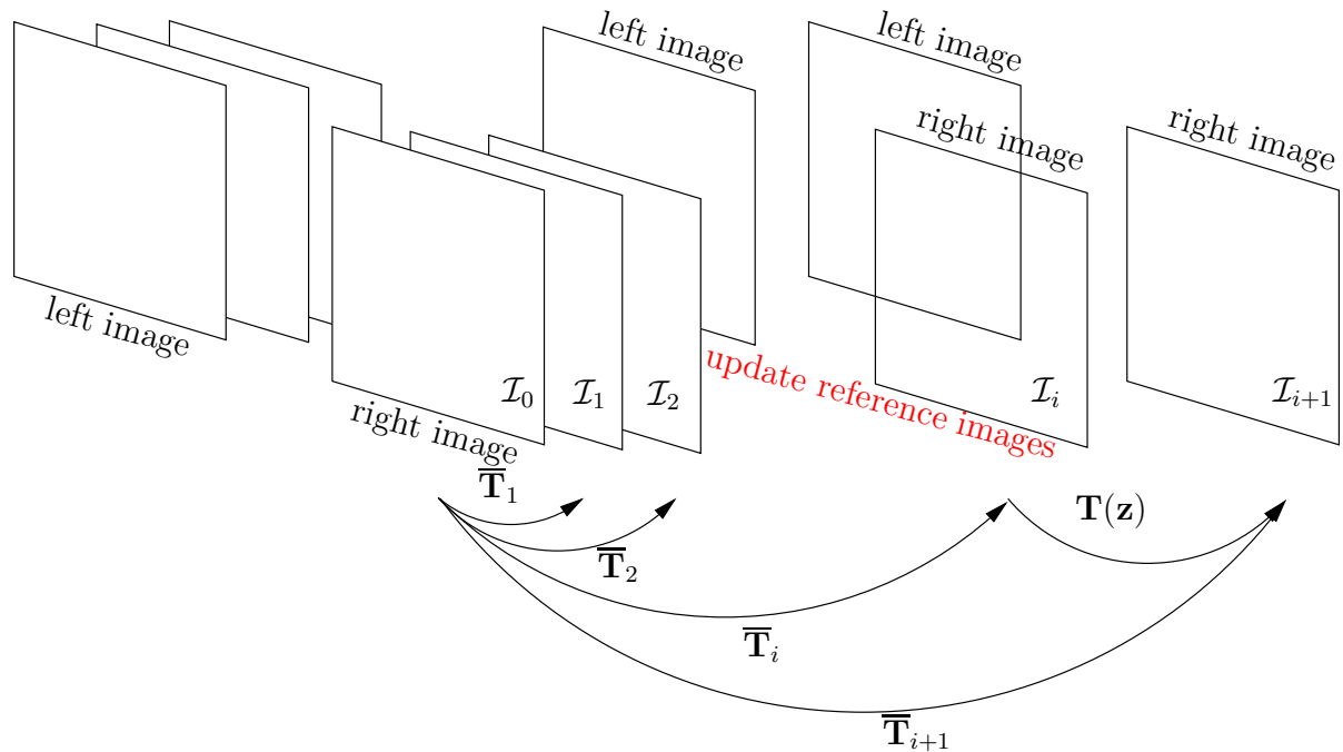
FIG. 3.12 – Incremental stereo visual SLAM.
