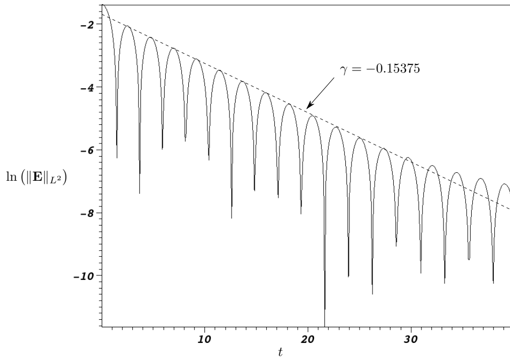
FIGURE 4.5 – Energie électrique en échelle logarithme pour un amortissement Landau linéaire avec \alpha = 0.05 , k_x = 0 , k_y = 0.5 , sur un maillage de \Omega_v de taille 128 \times 128 .
