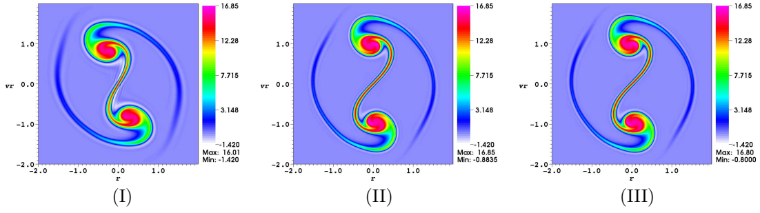
FIGURE 3.16 – Simulations (I), (II) et (III) d'un faisceau semi-gaussien au temps t = 5.984 , avec \omega_1 = 1 , H_1(\tau) = \cos^2(\tau) , \epsilon = 10^{-2} , et r_m = 1.85 .
