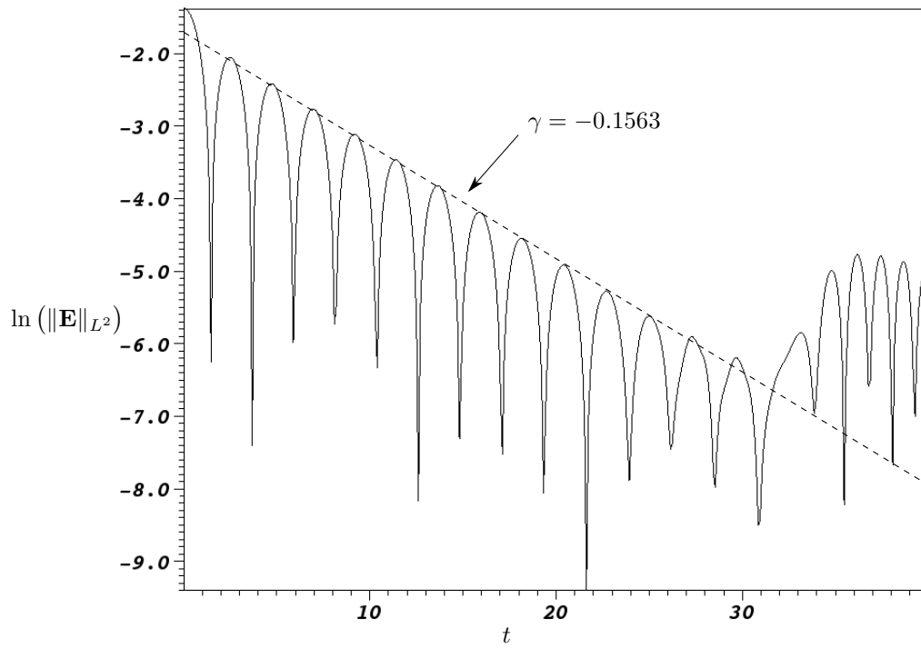
FIGURE 4.4 – Energie électrique en échelle logarithme pour un amortissement Landau linéaire avec \alpha = 0.05 , k_x = 0 , k_y = 0.5 , sur un maillage de \Omega_v de taille 64 \times 64 .
