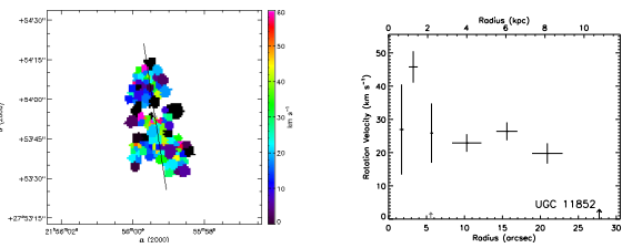
(186) UGC 11852
