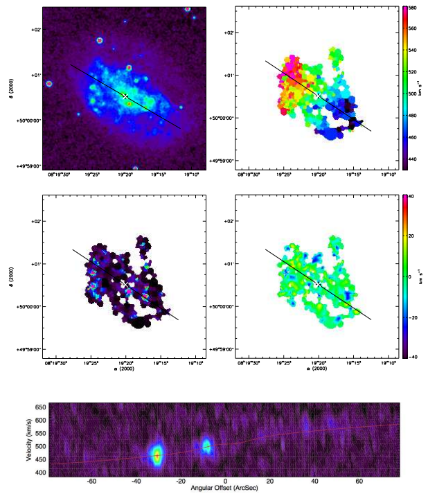
(62) UGC 04325
