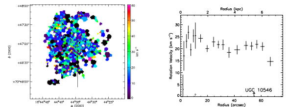
(160) UGC 10546
