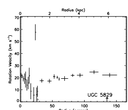
(92) UGC 05829
