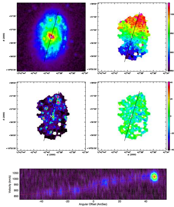
(121) UGC 07876
