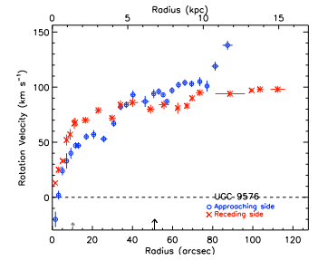
(123) UGC 09576
