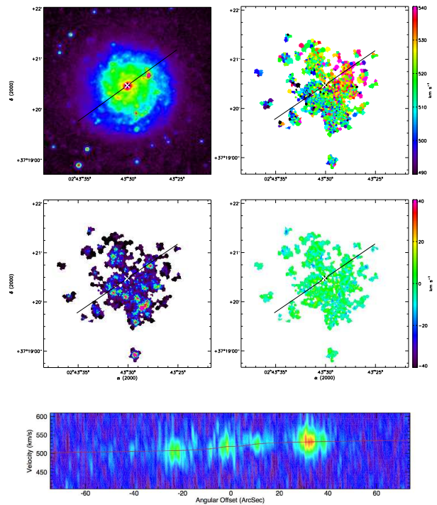
(26) UGC 02193
