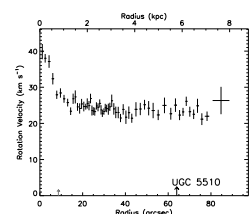
(86) UGC 05510
