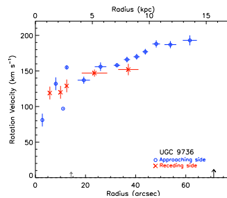
(125) UGC 09736
