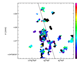
(92) UGC 05829
