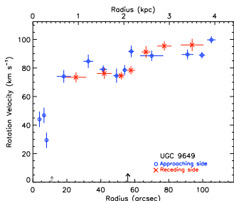
(124) UGC 09649
