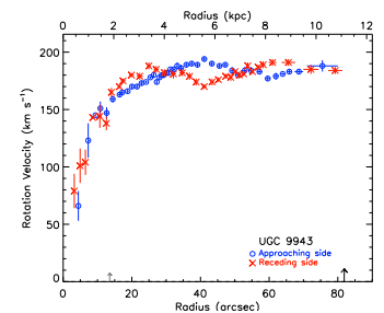
(129) UGC 09943
