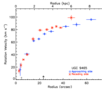
(122) UGC 09465
