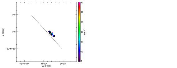
(21) UGC 02053
