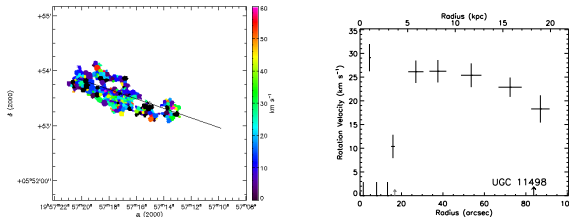
(181) UGC 11498
