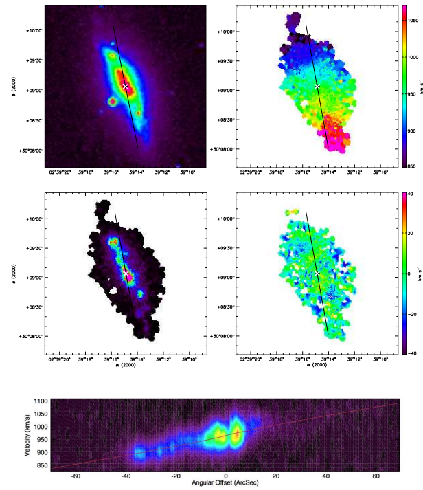
(24) UGC 02141
