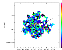
(94) UGC 05842
