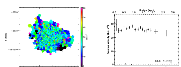
(162) UGC 10652
