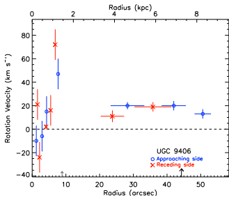
(121) UGC 09406
