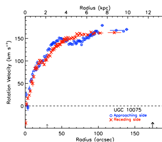
(131) UGC 10075
