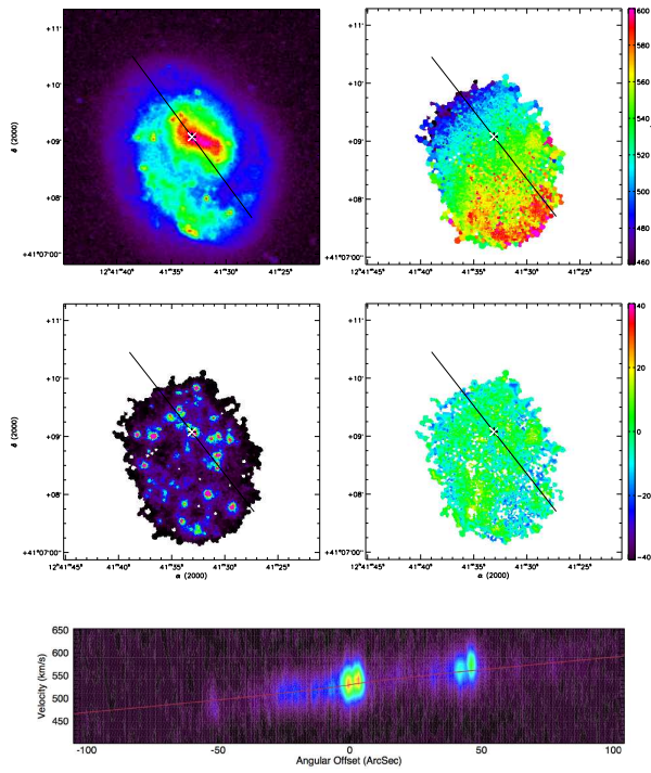
(119) UGC 07853
