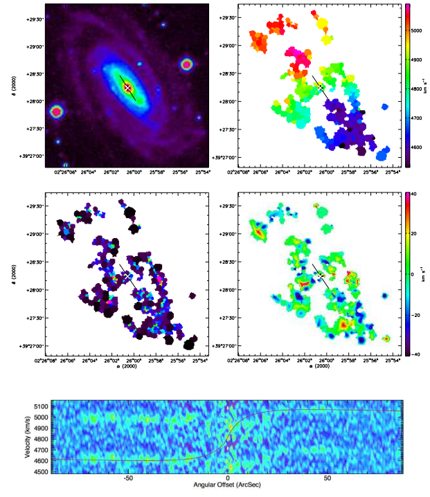
(16) UGC 01886
