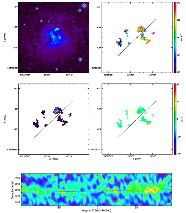
(18) UGC 02023
