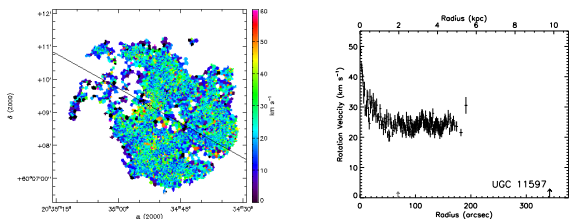
(183) UGC 11597
