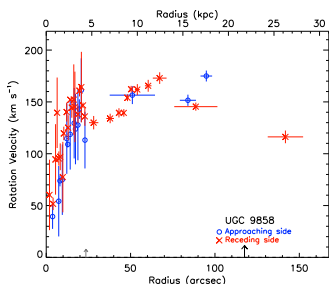
(127) UGC 09858
