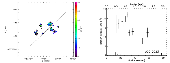
(18) UGC 02023
