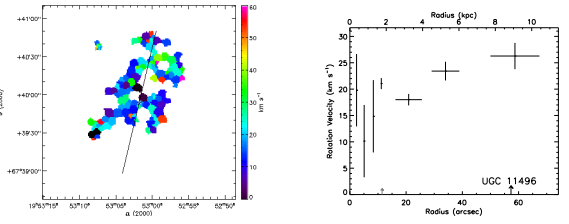
(180) UGC 11496
