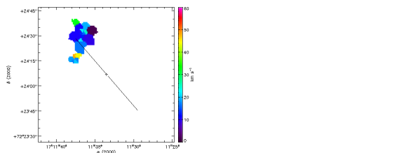
(165) UGC 10769
