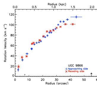
(128) UGC 09866
