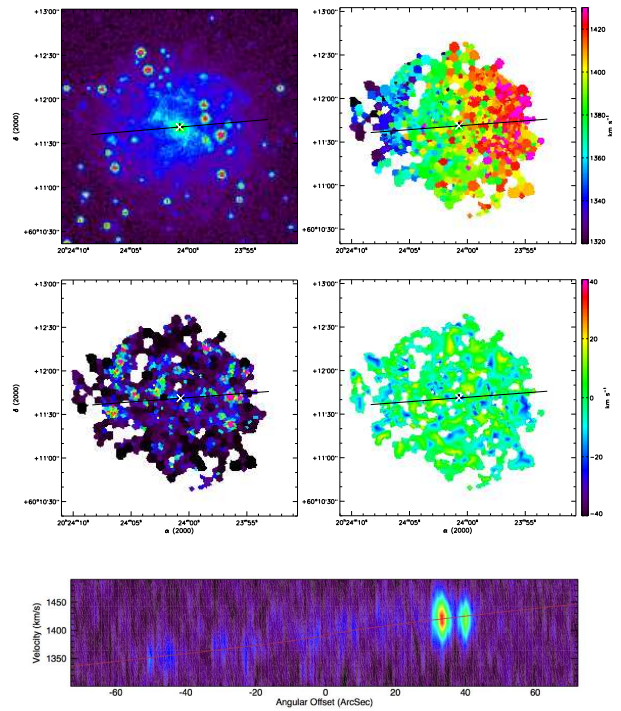
(182) UGC 11557
