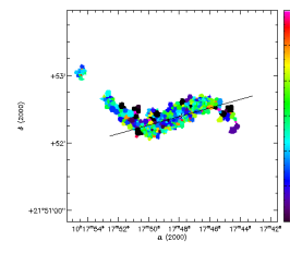
(88) UGC 05556
