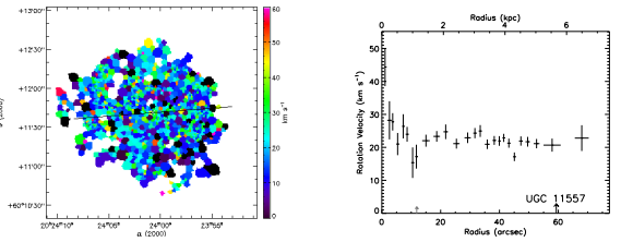
(182) UGC 11557
