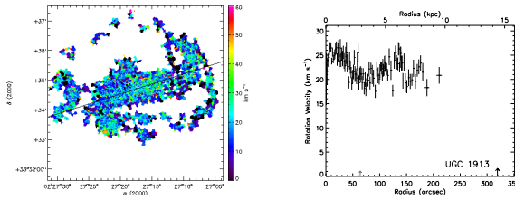
(17) UGC 01913
