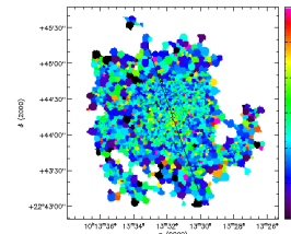
(86) UGC 05510
