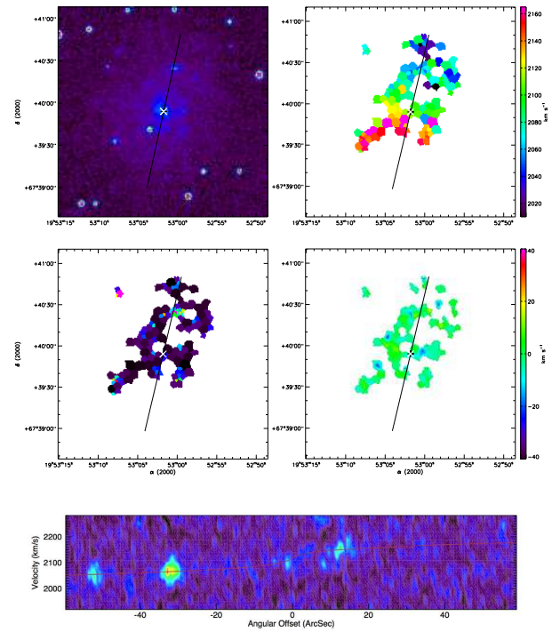
(180) UGC 11496
