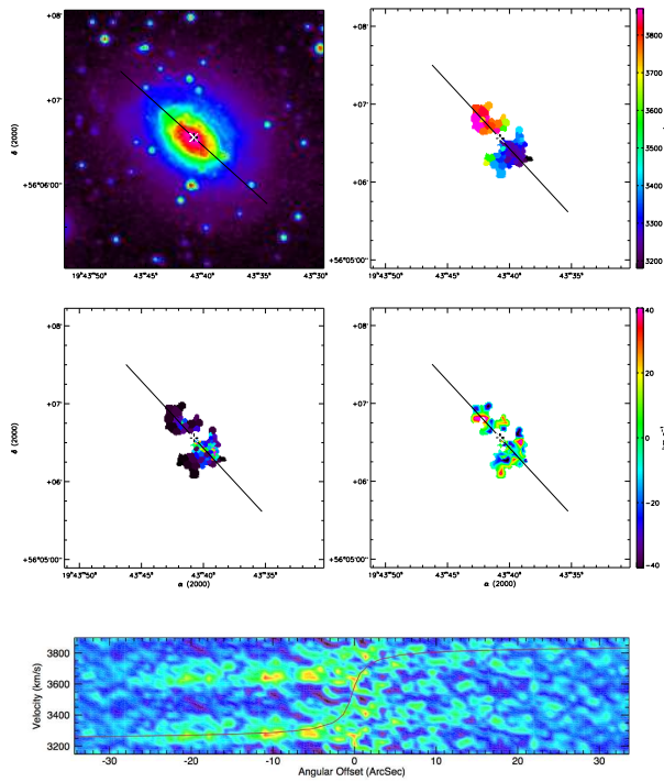
(179) UGC 11470
