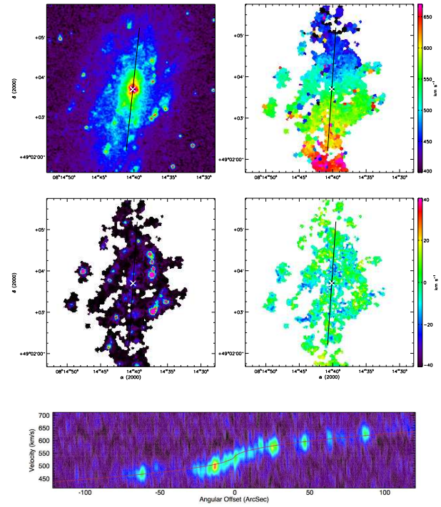
(60) UGC 04284
