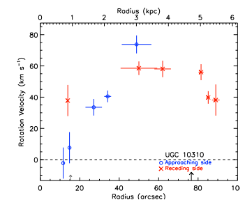
(132) UGC 10310
