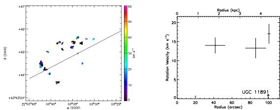
(189) UGC 11891
