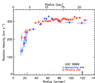
(130) UGC 09969
