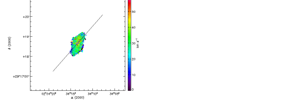
(20) UGC 02045
