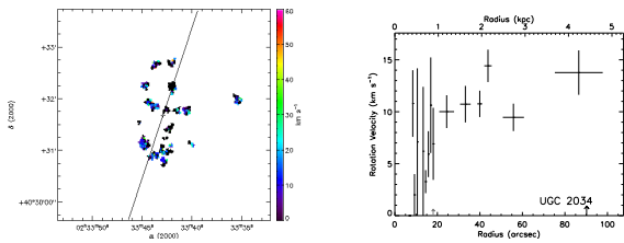
(19) UGC 02034
