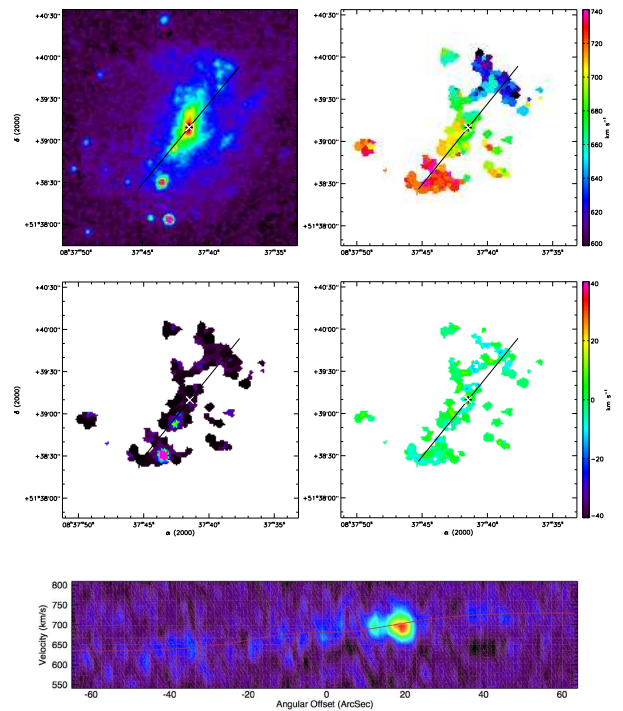
(66) UGC 04499
