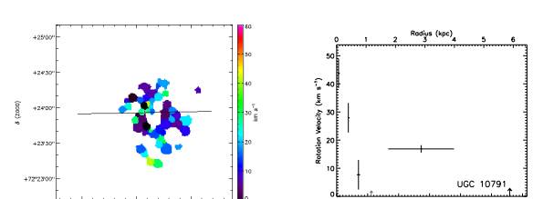
(166) UGC 10791
