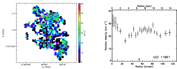
(187) UGC 11861
