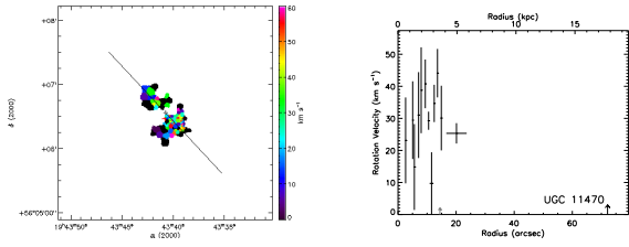
(179) UGC 11470
