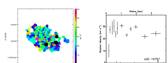
(164) UGC 10757
