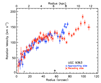
(120) UGC 09363
