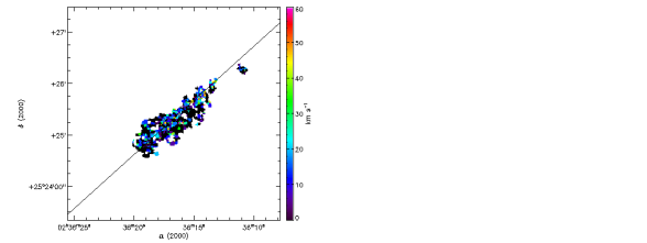
(22) UGC 02082
