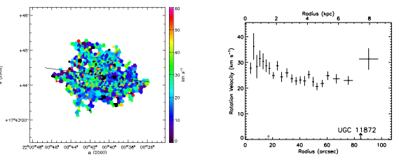
(188) UGC 11872
