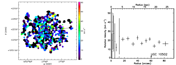
(158) UGC 10502
