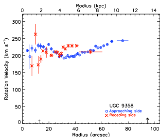
(118) UGC 09358
