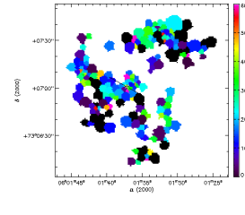
(36) UGC 03384
