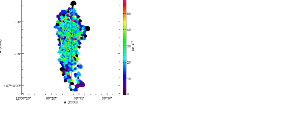
(190) UGC 11909
