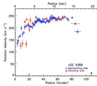
(119) UGC 09366
