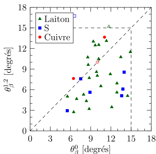
Fig. V.28 : Stabilité des orientations initialement dans la fibre \beta : désorientations par rapport à la composante à \varepsilon = 0 et \varepsilon = 1.2 . Les symboles ouverts représentent les grains ayant changé de composante.
