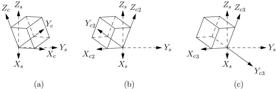
Fig. III.6 : Symétrie par rapport à un plan du SdC de référence. (a) Position originelle, (b) symétrie par rapport au plan de normale Y_s , (c) changement de Y_s en son opposé.
