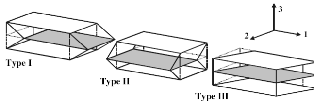
Fig. I.1 : Modèle Lamel : les deux grains considérés ont une face de normale DN commune. Les trois schémas illustrent les relâchements des cisaillements autorisés. D'après [7].
