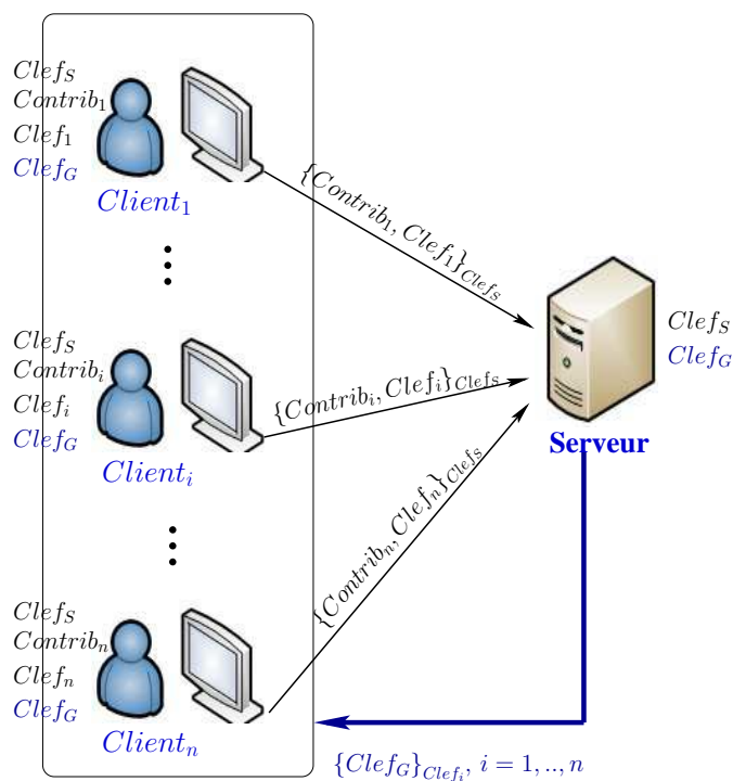
FIG. 1.2 – Exemple de génération d’une clef de groupe
