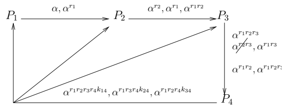
FIG. 3.5 – Attaque de secret futur individuel sur A-GDH.2 à quatre participants
