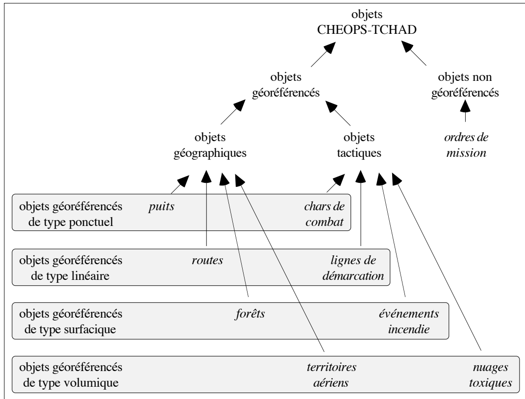
figure 6 : taxinomie des classes d'objets dans CHEOPS-TCHAD et prototypes associés
