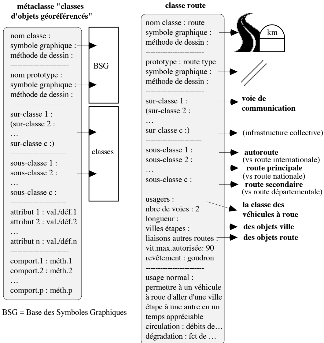
figure 3 : schéma d'organisation de la metaclass des classes d'objets géoréférencés et de la classe route
