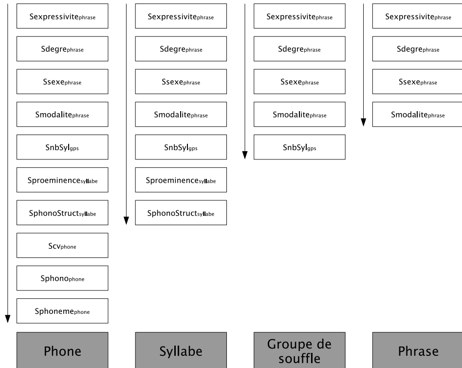
FIG. 4.6: Hiérarchie des variables contextuelles pour les unités de type : phone, syllabe, groupe de souffle et phrase.
