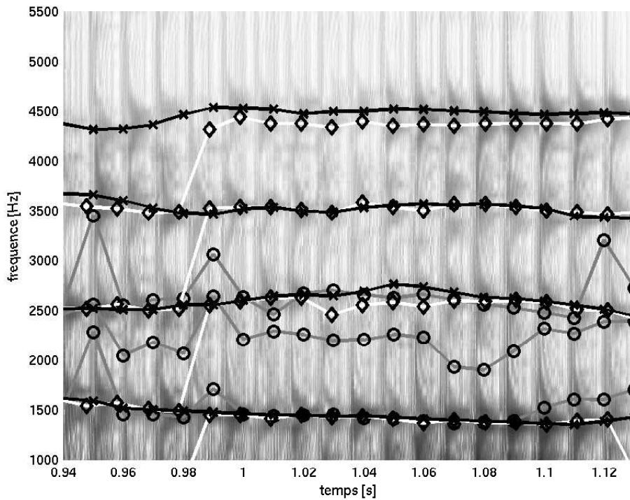
FIG. 3.8: Trajectoires de formants estimées par Praat (gris-cercle), par Wavesurfer (blanc-losange) et par la méthode formant-Viterbi proposée (noir-croix), tracées sur le spectrogramme d'une voyelle [A].
