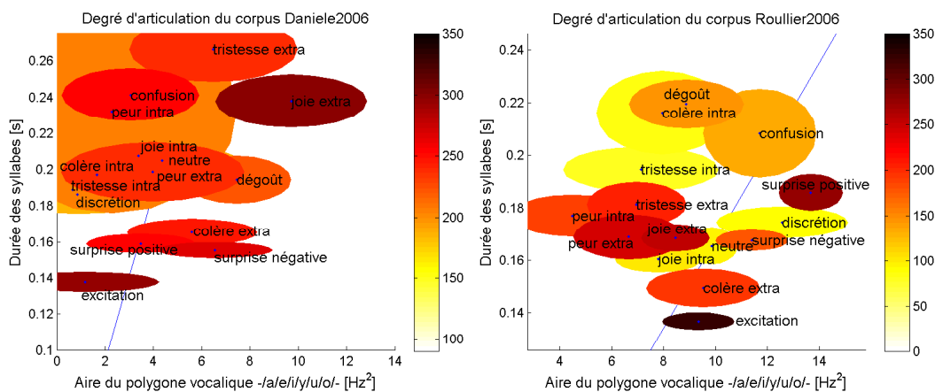
FIG. 3.26: Représentation des expressions dans un espace dont l'abscisse est l'aire couverte par le triangle vocalique [\times 10^4 \text{Hz}^2] , l'ordonnée est la durée des syllabes [s], et la couleur est la fréquence fondamentale [Hz]. A gauche : Daniele2006 ; A droite : Roullier2006.
