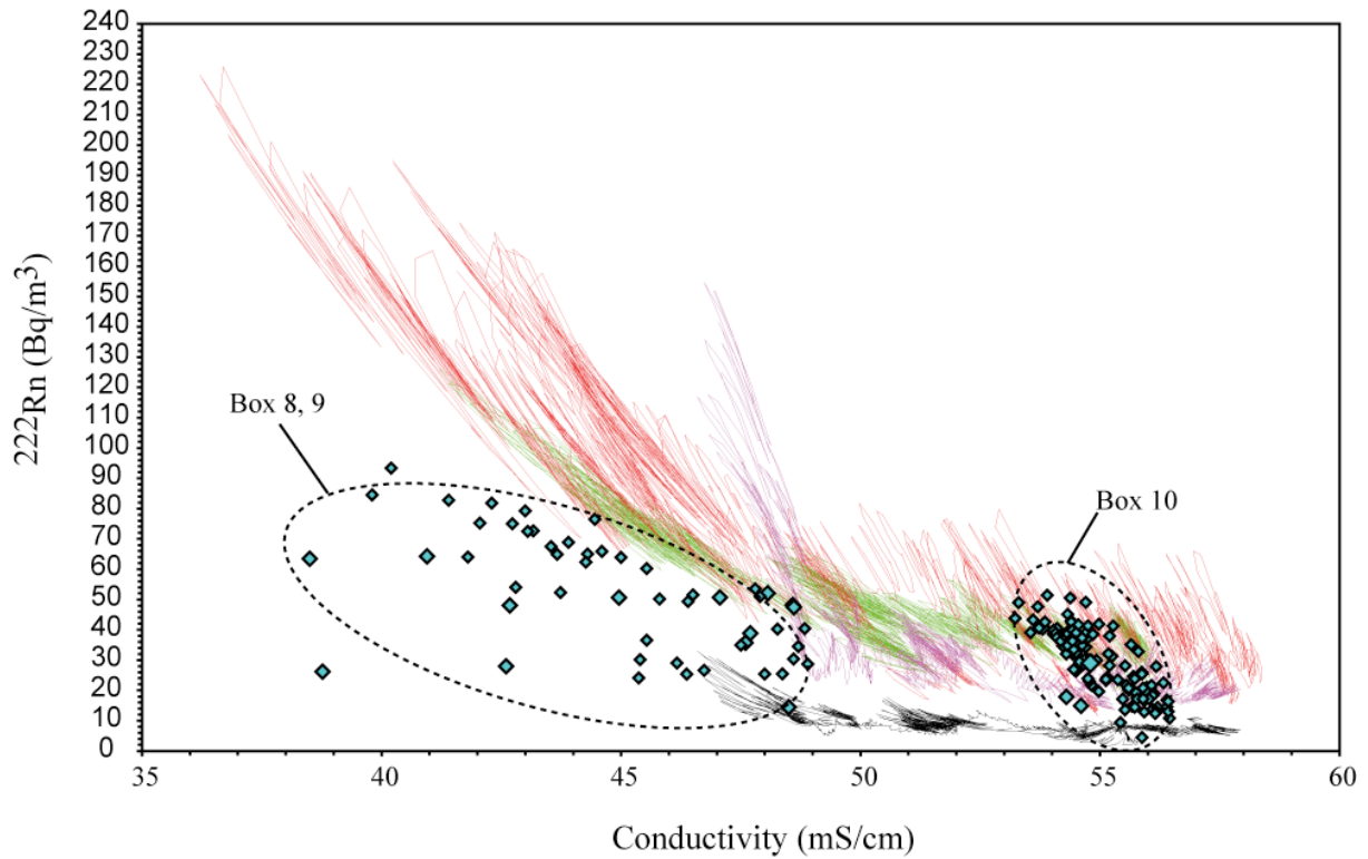
Figure V.5 : Activités de ^{222}\text{Rn} (Bq/m 3 ) en fonction de la conductivité, calculées par simulation pour les boîtes 7, 8, 9, 10 (cf texte). Les activités des échantillons mesurés pendant la thèse sont également reportées avec comme indication la boîte du site d'échantillonnage. Les symboles et couleurs sont identiques à ceux de la figure V.4.
