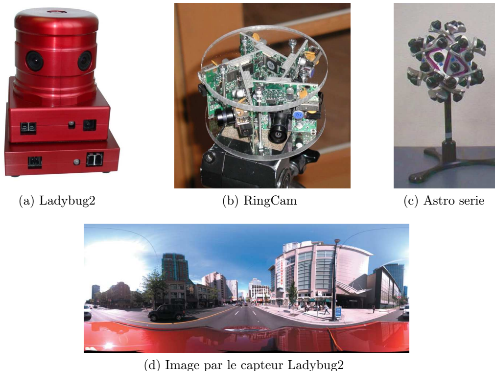
FIG. 1.7 – Quelques exemples de capteurs à réseau de caméras.
