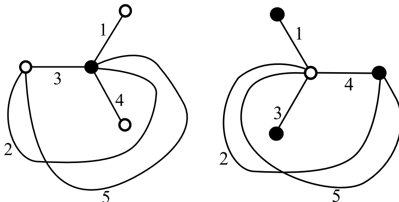
FIG. 2.8 – Cartes correspondant au minimum et au maximum de l'intervalle
