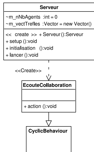
Figure 3.6: La classe Serveur et ses comportements.
