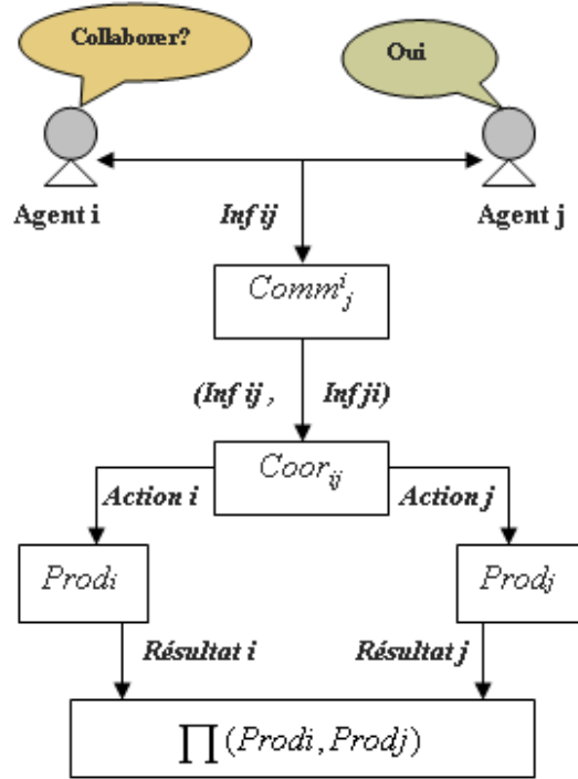
Figure 2.3: Le protocole de collaboration entre deux agents
