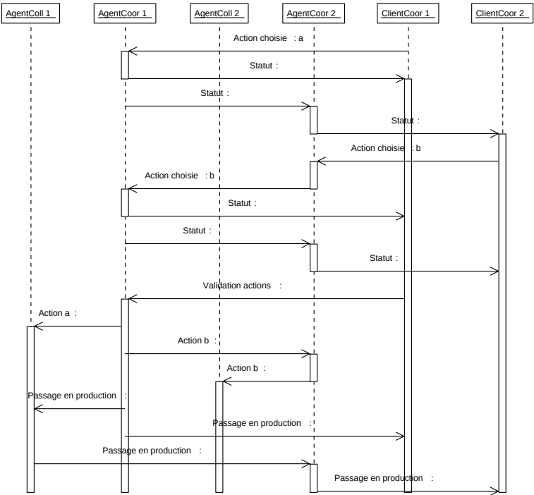
Figure 4.22: Diagramme de séquence de la validation des actions.
