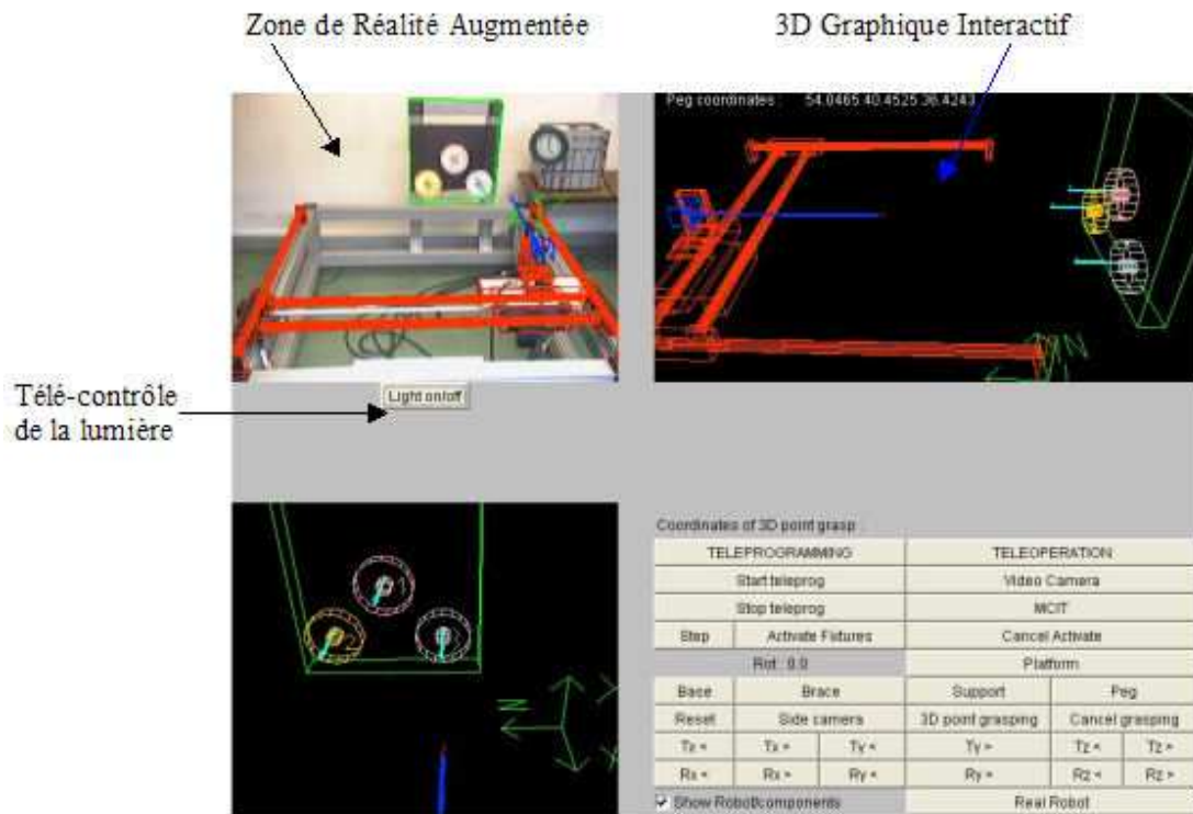
Figure 4.4: L'interface du système ARITI
