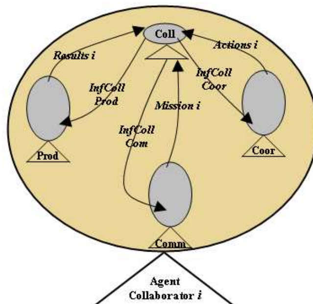
Figure 2.8: Interactions internes entre deux agents durant un processus de collaboration
