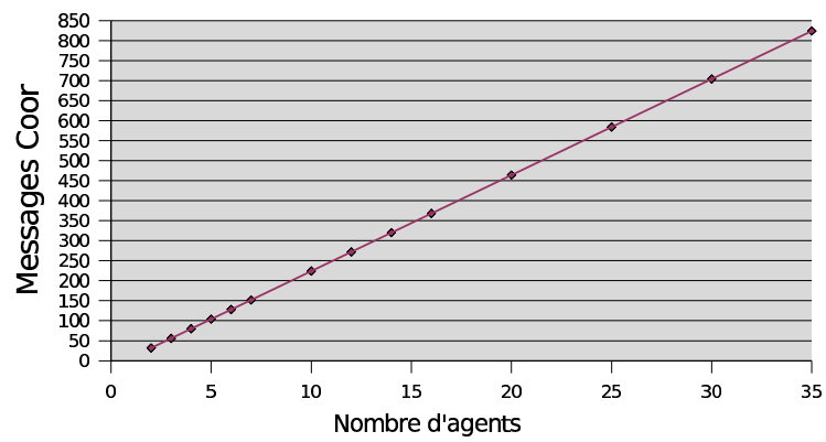
Figure 3.20: Nombre de messages émis par les agents coordination
