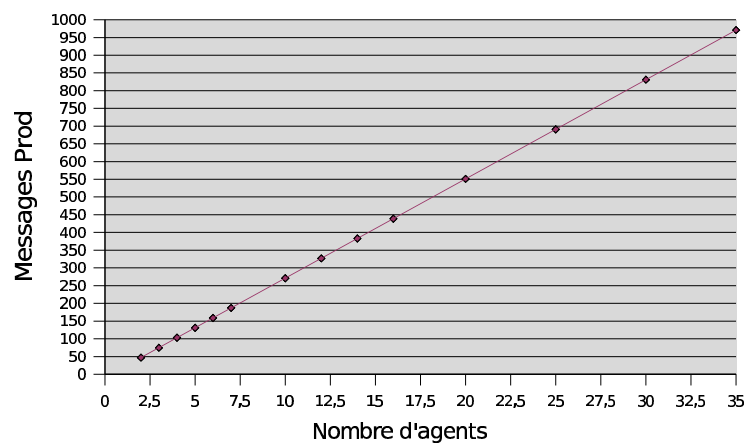
Figure 3.22: Nombre de messages émis par les agents production
