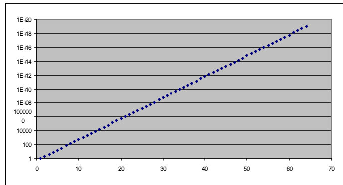
Figure 17. u_{n+1} = 2 \times u_n L'axe Y en échelle logarithmique
