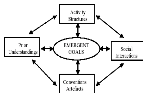
Figure 1. Modèle de Saxe à quatre paramètres (Monaghan, 2004)
