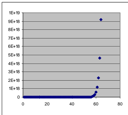
Figure 18. u_{n+1} = 2 \times u_n en échelle linéaire
