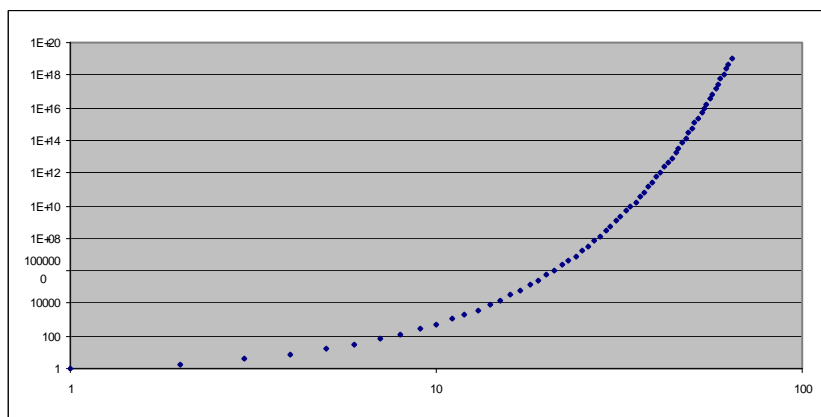
Figure 19. u_{n+1} = 2 \times u_n , Les deux axes en échelle logarithmique
