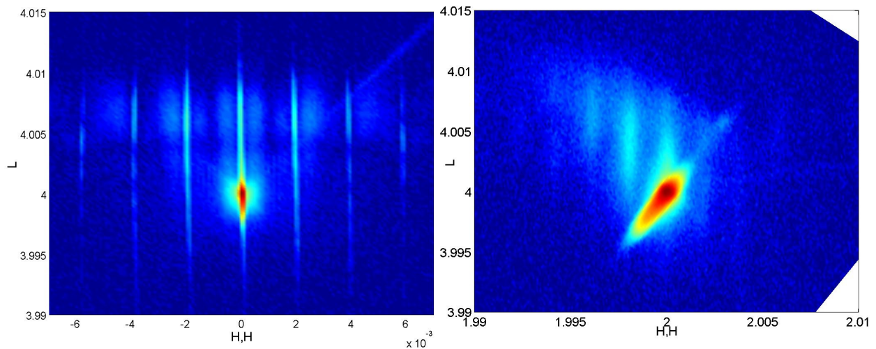
Figure IV- 16: Cartographie 004 (gauche) et 224 (droite) du Silicium. Remplissage des tranchées avec du SiO 2 déposé à l'aide de TEOS-ozone. Mesure avec optique hybride. p= 200 nm.
