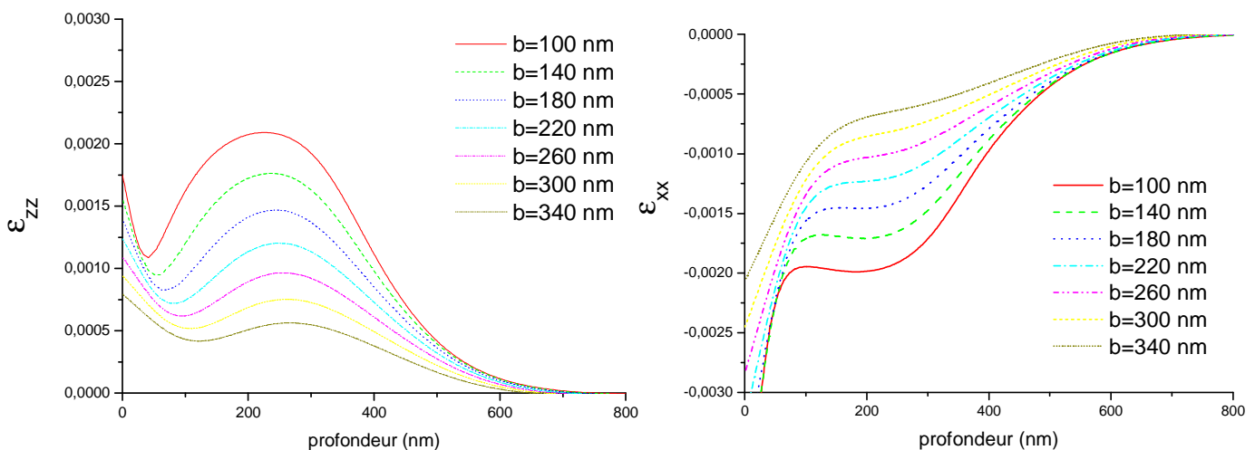
Figure I- 21: Variation de \epsilon_{zz} (gauche) et de \epsilon_{xx} (droite) au milieu de la ligne de silicium en fonction de la profondeur pour différentes valeurs de b . h=410 nm, p=580 nm.
