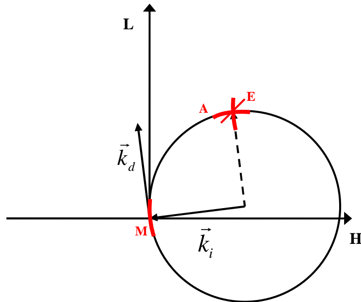
Figure III- 20: Schéma montrant l'origine des signatures du monochromateur (M), de l'analyseur (A) et de la dispersion énergétique (E).
