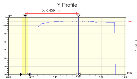
Figure II.17 : Exemple de déflexion du microcommutateur résistif à configuration série
