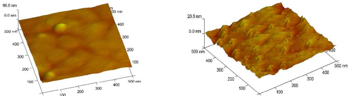
Figure IV.42 : Rugosité de la ligne ( R_a=3.24\text{nm} et R_{\text{max}}=54.6\text{nm} ) et du pont ( R_a=1.14\text{nm} et R_{\text{max}}=10.5\text{nm} )
