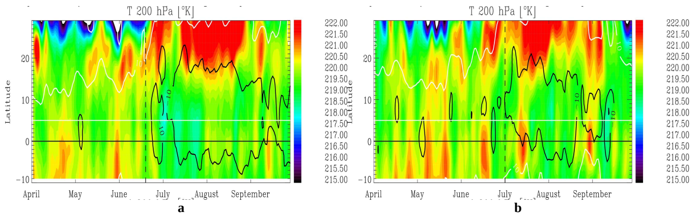
Figure II-13 : Diagrammes Hovmöller temps/ latitude de la température à 200 hPa (a) de la saison 1999 (b) de la saison 2000. En pointillé l'Onset de la saison. Superposé en contour blanc, le STJ ( 10 \text{ m.s}^{-1} ), en contour noir le TEJ ( 10 \text{ m.s}^{-1} ).
