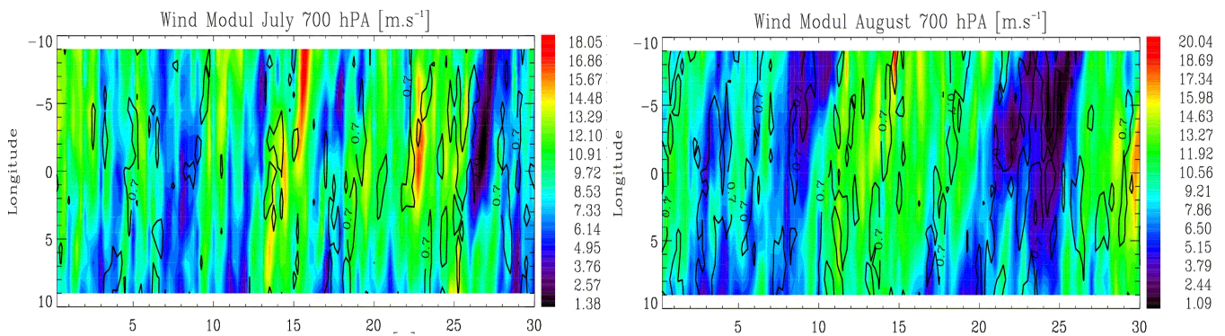
Figure III-8 : Diagrammes Hovmöller temps/longitude du module du vent à 700 hPa (fond de couleur) et de la couverture nuageuse totale du modèle (isoligne noir) (a) pour le mois de Juillet (b) pour le mois d'Août.
