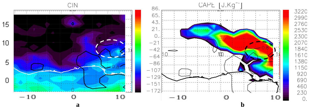
Figure III-11 : Coupes horizontales le 27 Juillet à 1800 UTC : (a) du CIN et (b) du CAPE. La couverture nuageuse du modèle est en isocontour noir. Le cercle en tiré (a) blanc ou (b) noir, localise la convection étudiée.
