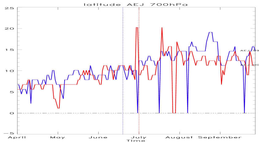
Figure II-18 : Diagramme Hovmöller temps/latitude de la position du maximum de vorticité de l'AEJ en 1999 (courbe bleu) et en 2000 (courbe rouge). En pointillé les Onset des saisons (bleu : 1999 et rouge : 2000).
