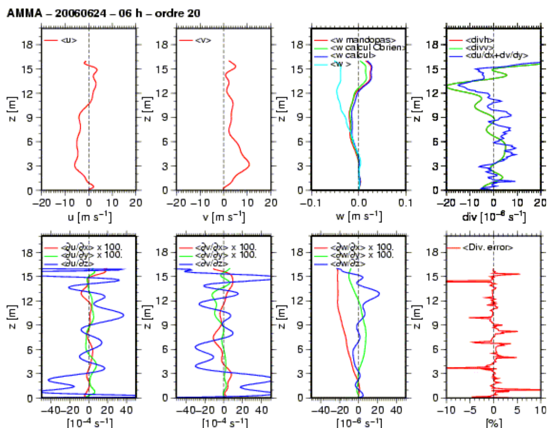
Figure IV-15 : Restitution du champ vent mesuré le 24 Juin 2006 à 06h. Sur la première ligne, chaque figure présente de gauche à droite les données analytiques simulées (bleu ciel) et restituée (rouge) pour la composante zonale, la composante méridienne, la composante verticale du vent, et la divergence. La seconde ligne présente les dérivées en x (rouge), y (vert), z (bleu) des différentes composantes du vent, et l'erreur entre les divergences horizontale et verticale restituées.
