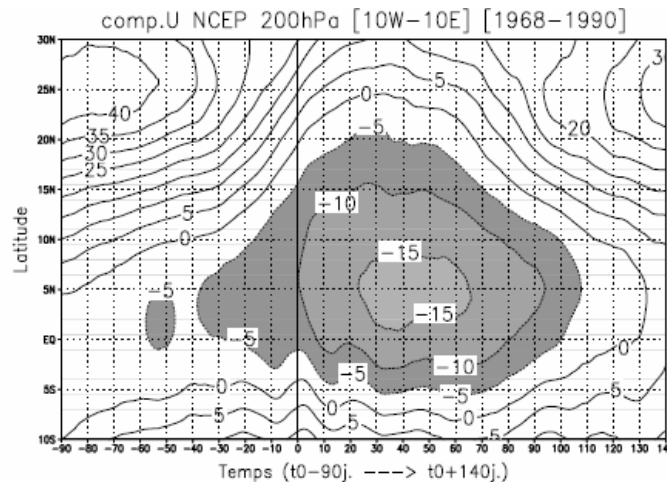
Figure I-11 : Diagramme Hovmüller Temps – Latitude de la composante zonale du vent ( \text{m.s}^{-1} ), entre 1968 et 1990 moyennée sur les longitude 10°E-10°O à 200 hPa, provenant des réanalyses NCEP/NCAR (Sultan, 2002).
