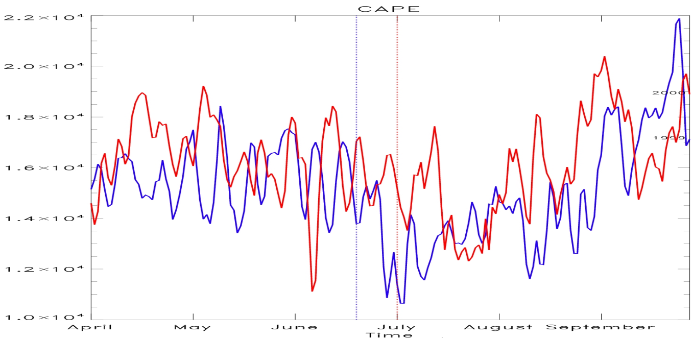
Figure II-22 : Evolution temporelle du maximum de CAPE ( J.Kg^{-1} ), lors de la mousson 1999 (courbe bleue) et lors de la mousson 2000 (courbe rouge). En pointillé les Onset des saisons (bleu : 1999 et rouge : 2000).
