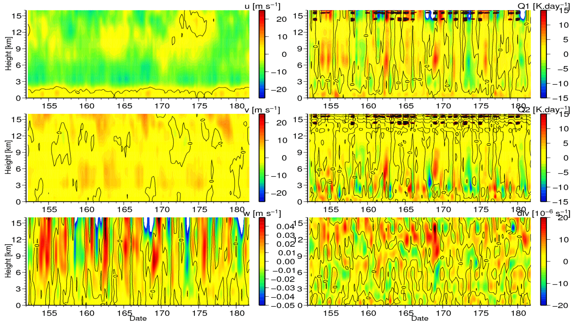
Figure IV-30 : Série temporelle du mois de Juin (jour julien), des profils verticaux de u , v , w , Q1 , Q2 , et de la divergence verticale de w . Ces profils sont calculés par MANDOPAS sur le quadrilatère de l'expérience AMMA.
