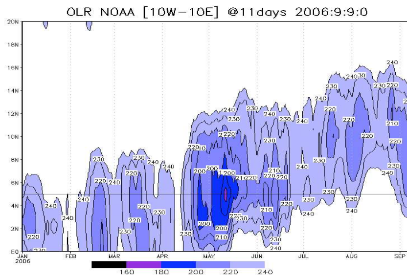
Figure II-31 : Image OLR NOAA ( W.m^{-2} ) mettant en évidence le déplacement des nuages vers le nord, (Janicot et al., 2008).
