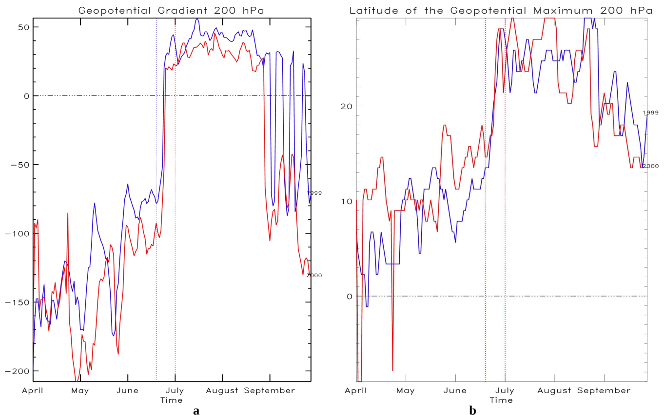
Figure II-15 : Evolution temporelle (a) gradient maximum de géopotential ( m^2s^{-2} ), et (b) de sa latitude (°) pour les années 1999 (bleu) et 2000 (rouge). En pointillé les Onset des saisons (bleu : 1999 et rouge : 2000).
