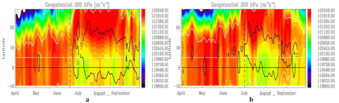
Figure II-11 : Diagrammes Hovmöller temps/ latitude du géopotential à 200 hPa (a) de la saison 1999 (b) de la saison 2000. Superposé en contour blanc, le STJ (10 m.s -1 ), en contour noir le TEJ (10 m.s -1 ), en pointillé l'Onset de la saison.
