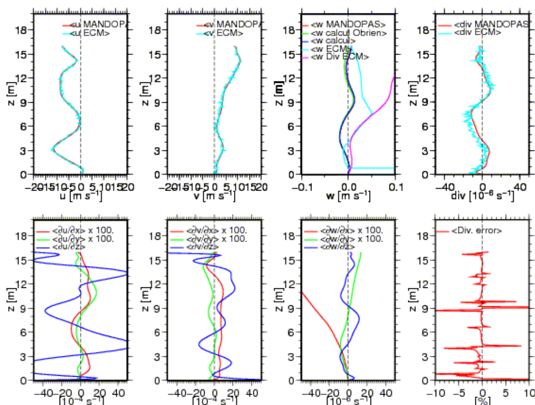
Figure IV-11 : Restitution d'un champ de vent issu du Centre Européen (ECMWF) du 28 Juillet 2006 à 12h par MANDOPAS bilinéaire avec 5 Radiosondages en entrée. Sur la première ligne, chaque figure présente de gauche à droite les données du Centre Européen (bleu ciel) et restituée (rouge) pour la composante zonale, la composante méridienne, la composante verticale du vent, et la divergence. La seconde ligne présente les dérivées en x (rouge), y (vert), z (bleu) des différentes composantes du vent, et l'erreur entre les divergences horizontale et verticale restituées.
