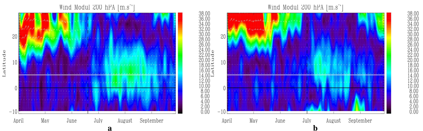
Figure II-14 : Diagrammes Hovmöller temps/ latitude du module du vent à 200 hPa (a) de la saison 1999 (b) de la saison 2000. En pointillé l'Onset de la saison.
