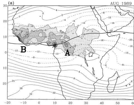
Figure I-12 : Coupe horizontale de la Composante U du vent à 200 hPa ( m.s^{-1} ) sur l'Afrique de l'Ouest. Les zones grises représentent les précipitations au sol (Nicholson et Grist, 2003).
