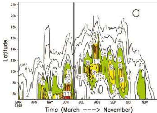
Figure I-14 : Diagramme temps – latitude du 1 mars au 30 novembre 1978 des précipitations journalières ( \text{mm}\cdot\text{jour}^{-1} ) moyennées entre 10°O – 10°E (Sultan et Janicot, 2003).
