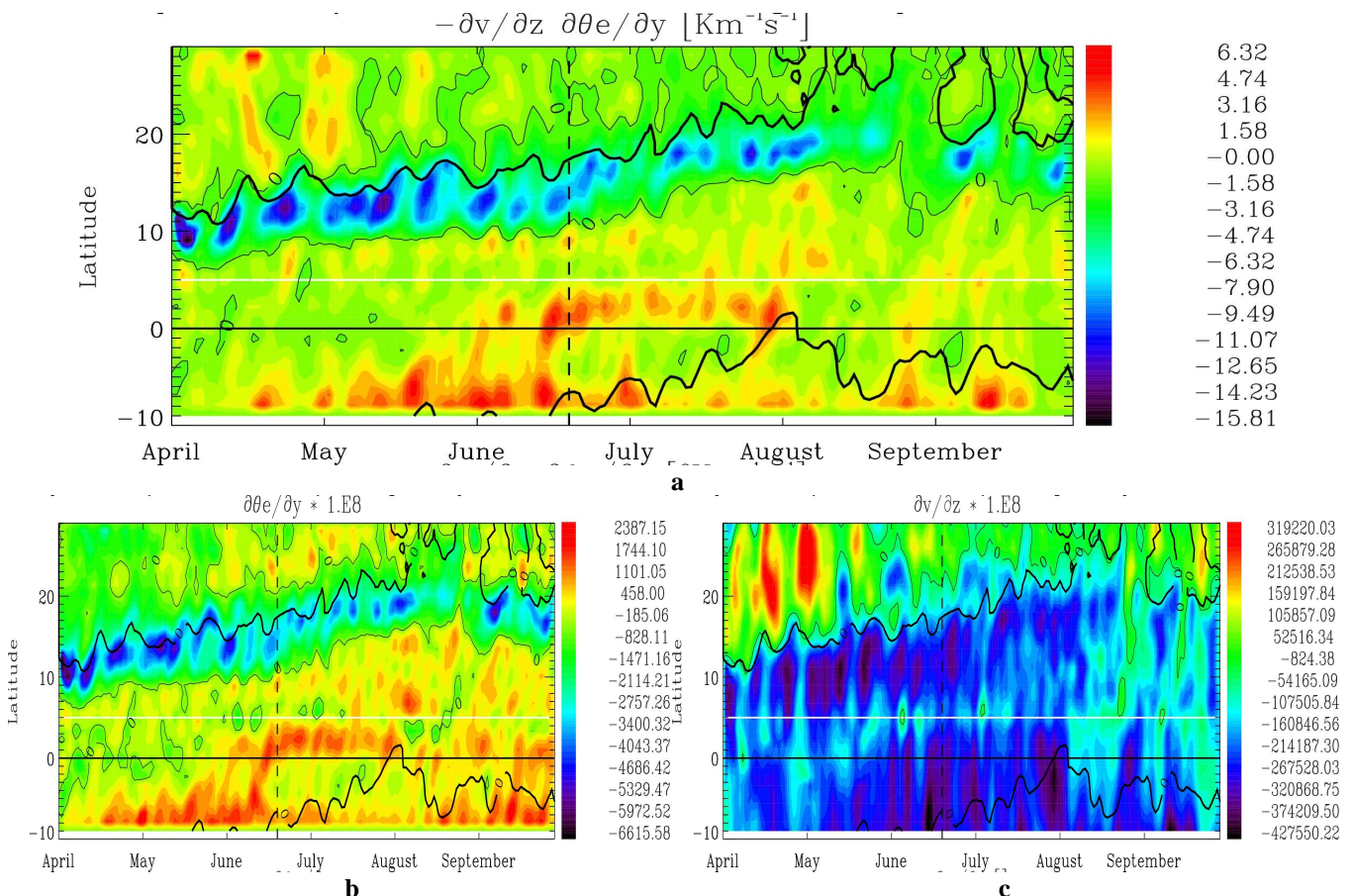
Figure II-29 : Diagrammes temps/latitude pour l'année 1999, (a) de -\frac{\partial v}{\partial z} \frac{\partial \theta_e}{\partial y} , (b) de \frac{\partial \theta_e}{\partial y} et (c) de \frac{\partial v}{\partial z} .
