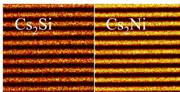
Figure III.44 – Images ioniques ( 19,5 \times 19,5 \mu m^2 ) obtenues par ToF-SIMS pour des lignes de silicium et de STI de 1 \mu m de largeur. Les espèces Cs_2Si et Cs_2Ni sont acquises.
