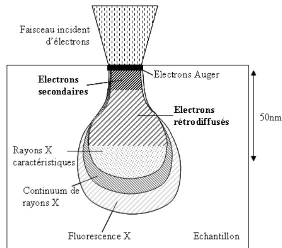
Figure II.19 - Représentation schématique d'une poire de diffusion d'un faisceau d'électron incident.
