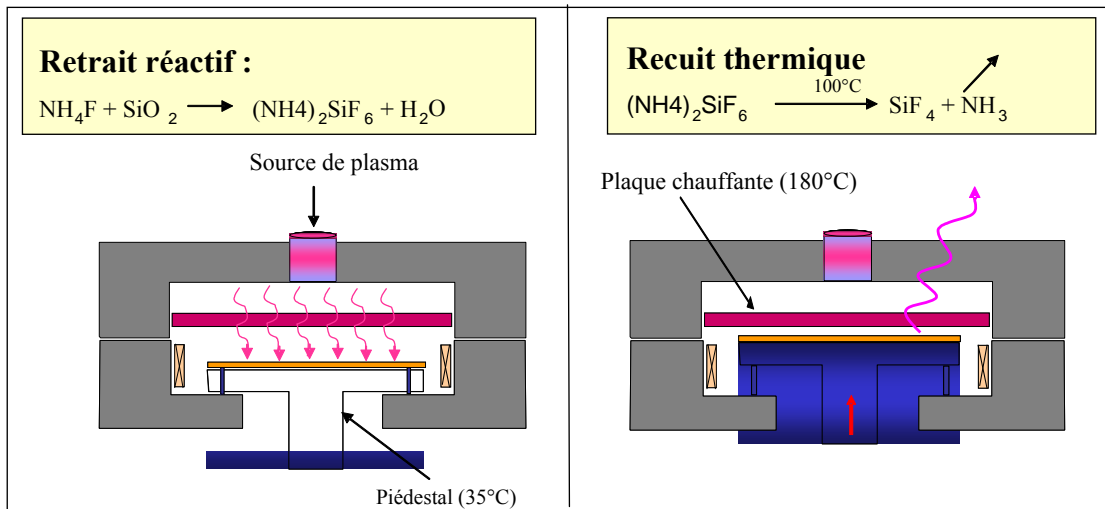
Figure III.2 – Représentation schématique des deux étapes de retrait réactif et de recuit thermique (100°C) de la préparation de surface par plasma réactif in-situ \text{NH}_4\text{F}/\text{NH}_3 .
