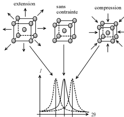
Figure II.7 – Variation des spectres \theta - 2\theta en fonction des contraintes internes de l'échantillon.
