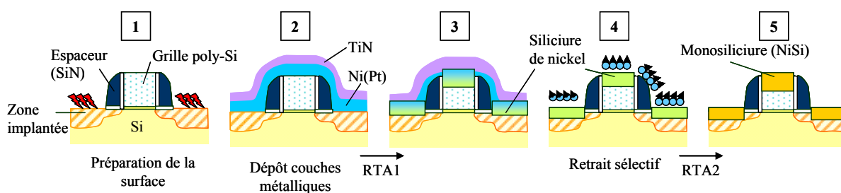
Figure III.1 – Représentation schématique des étapes du procédé SALICIDE appliquées aux transistors CMOS.
