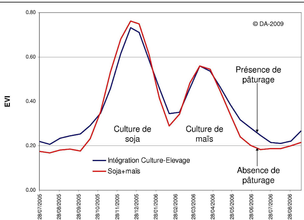
Figure 2.22 : Comparaison du profil moyen de EVI des classes « Intégration Culture-Elevage » et « Soja+maïs ».
