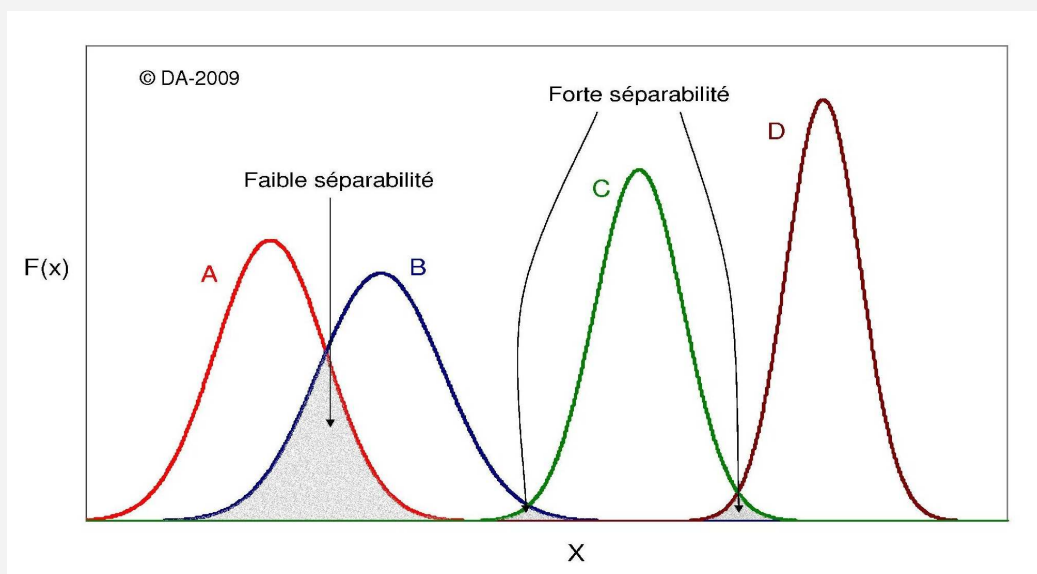
Figure 2.8 : Présentation du principe des tests de séparabilité entre 4 classes A, B, C et D. Les classes A et B sont faiblement séparables. La classe C est fortement séparée des classes B et D. Il n'y a pas de confusion possible entre les paires de classes A-C, A-D et B-D.
