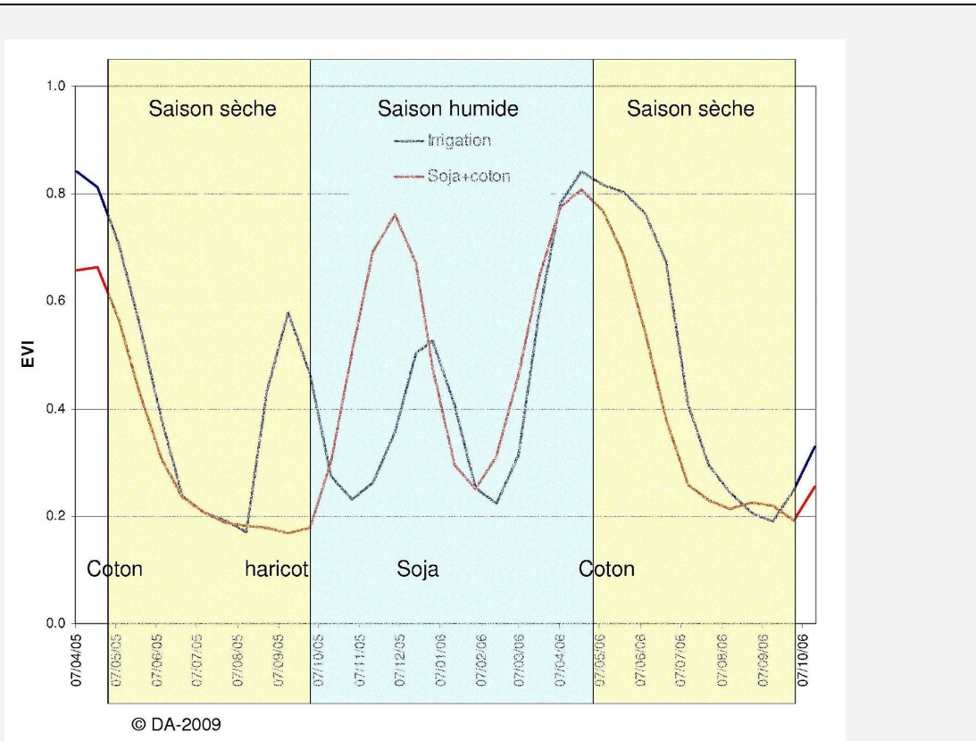
Figure 2.24 : Comparaison d'un profil temporel de EVI d'un pixel avec un pivot en saison sèche et du profil moyen de la classe « soja+coton » (sans pivot).
