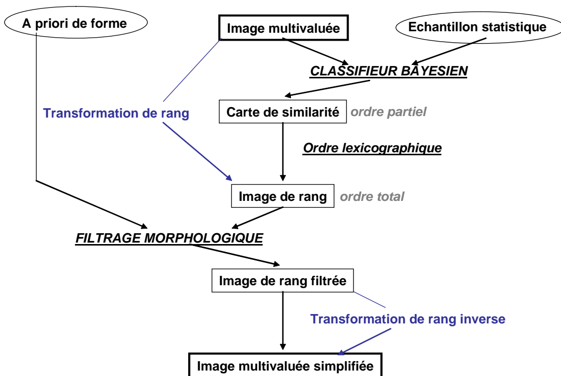
FIG. 2.1: Prise en compte d'informations statistiques et géométriques pour l'analyse des images multivaluées.
