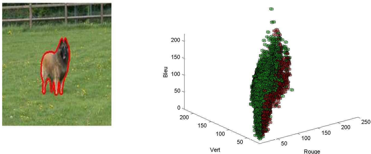
FIG. 2.16: Afin de comprendre la complexité du problème, il faut transposer l'image dans l'espace des caractéristiques. Dans cet exemple, deux classes sont représentées dans l'espace RGB. Les deux classes sont correctement séparées et peuvent être incluses dans des hyperellipses. Par conséquent, la carte des distances constituera un support favorable à une segmentation.
