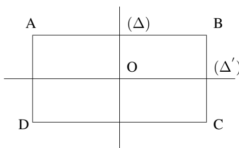
FIG. 1.7: Table d'addition du groupe de Klein, \mathbb{Z}/2\mathbb{Z} \times \mathbb{Z}/2\mathbb{Z} en haut à gauche. Si nous définissons par i l'identité, s_1 la réflexion d'axe \Delta , s_2 la réflexion de \Delta' et enfin s la symétrie de centre O , nous pouvons dresser une table équivalente pour le groupe des isométries laissant A, B, C, D invariants. Les deux groupes sont isomorphes mettant en avant la similitude de leurs structures internes bien que leurs éléments soient différents. En effet, le groupe de Klein est composé des éléments \{(0, 0), (0, 1), (1, 0), (1, 1)\} , alors que le groupe des isométries contient \{i, s_1, s_2, s\} .
