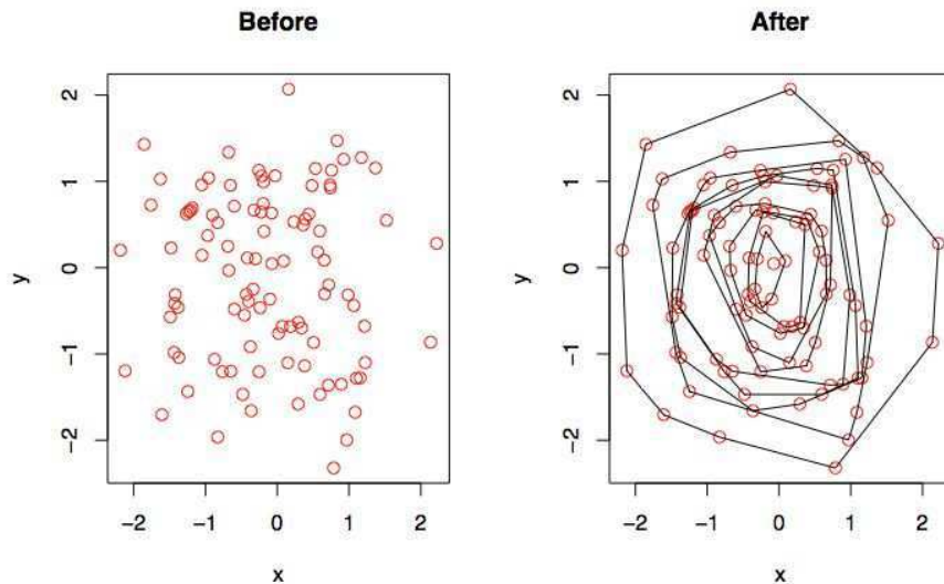
FIG. 1.13: Illustration du principe du « convex hull peeling », les vecteurs sont regroupés en enveloppes convexes incluses les unes dans les autres (image extraite de la présentation sur le sujet par [72]).
