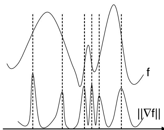
FIG. 2.13: Fonction à variations lentes et partition en bassins versants.
