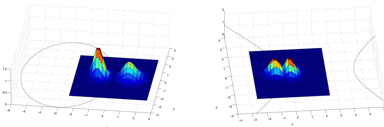
FIG. 2.5: Illustration des courbes de décision lorsque les matrices de covariance changent. Dans les deux cas, les moyennes sont identiques ( \mu_1 = [0; 0] et \mu_2 = [-1; 0] ), à gauche les matrices de covariance sont \Sigma_1 = [0.1, 0.0; 0.0, 0.15] et \Sigma_2 = [0.2, 0; 0, 0.25] , la courbe est alors une ellipse d'équation -\frac{5}{2}x^2 - \frac{4}{3}y^2 - 15x - 1.296 = 0 . À droite, \Sigma_1 = [0.1, 0; 0, 0.15] et \Sigma_2 = [0.15, 0; 0, 0.1] l'équation devient une hyperbole ( -x^2 + y^2 + 4x + 2 = 0 ).
