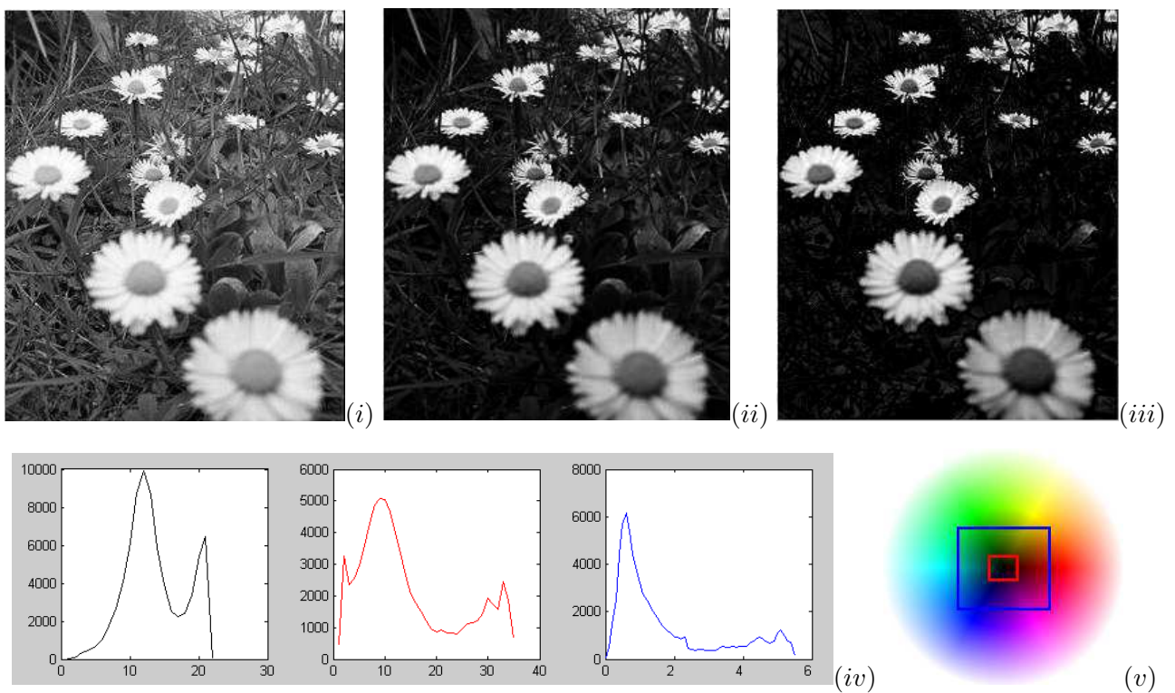
FIG. 2.8: Comparaison des distances d'Euclide (i) et de Mahalanobis ((ii) et (iii)) pour des échantillon de référence de variance croissante. L'origine pour le calcul de la distance euclidienne est le point 0. Les échantillons de référence pour le calcul de la distance de Mahalanobis sont indiqués en rouge (cas (ii)), bleu (cas (iii)) sur la figure (v).
