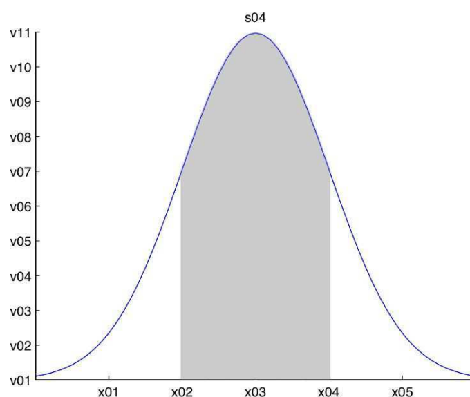
FIG. 2.2: Représentation de la loi normale ( \mu = 0, \sigma^2 = 4 ). La probabilité d'appartenance est représentée par la surface sous la courbe. Ainsi, la partie hachurée \int_{-\sigma}^{+\sigma} f(x) \approx 0.68 , représente la grande majorité des possibilités, c'est-à-dire 68%. Par exemple, si les caractéristiques de la forme suivent une loi normale de moyenne \mu et de variance \sigma^2 , alors environ 68% des points auront une valeur entre \mu \pm \sigma .
