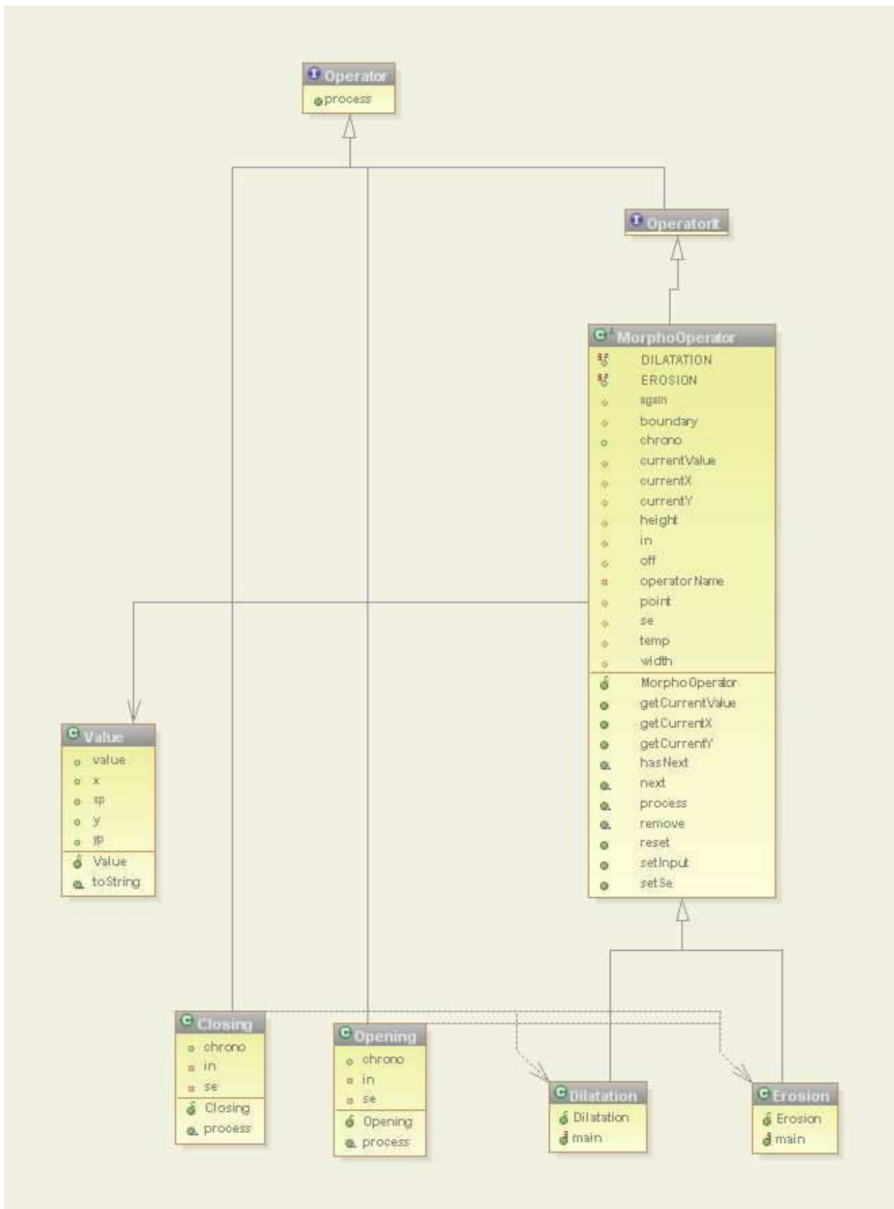
FIG. 3.33: Package contenant la construction des opérateurs morphologiques pour les scalaires. Érosion et dilataion dérivent tous les deux d'une classe abstraite contenant toute la logique métier. La classe de base toute MorphoOperator implémente également la classe Iterator afin d'offrir un moyen simple et efficace pour rendre la main à chaque traitement.
