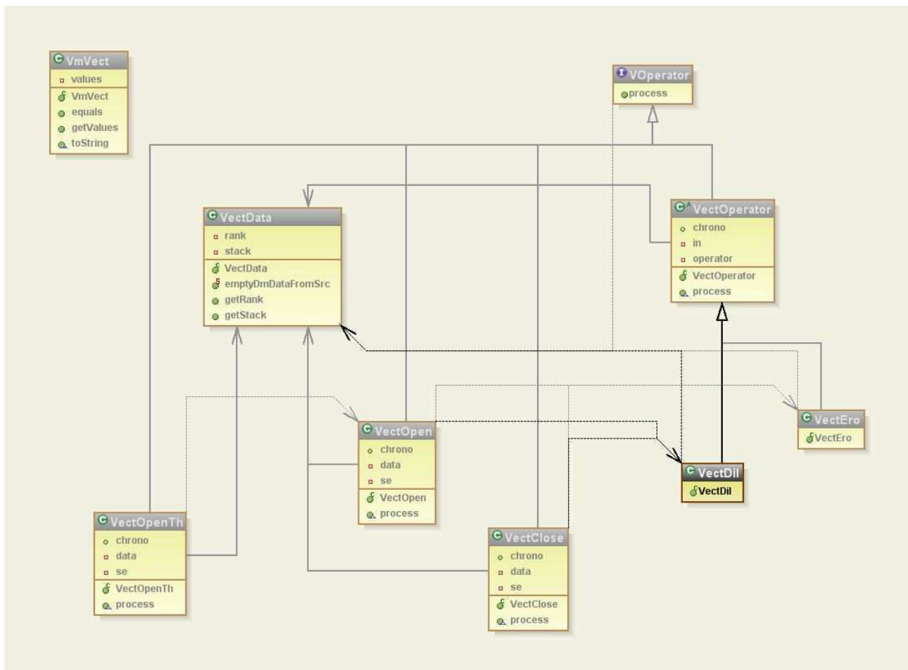
FIG. 3.34: Package contenant la construction des opérateurs vectoriels. Érosion et dilation dérivent également d'une classe abstraite. Cette classe utilise la logique métier de MorphoOperator que nous utilisons pour le traitement des scalaires.
