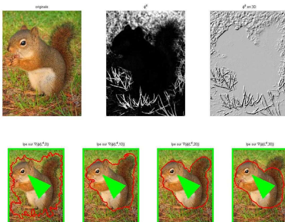
FIG. 2.15: Segmentation par calcul de la ligne de partage des eaux sur la carte des distances. En haut, l'image originale, la carte des distances et sa représentation 3D. L'échantillon de référence est l'écureuil (zone triangulaire verte représentée en superposition sur l'image). Cette zone sert également de source d'inondation lors du calcul de la ligne de partage des eaux. En bas, trois résultats de la segmentation par LPE sur le gradient de la carte des distances. En fonction des différentes fermetures (disque de taille 0, 10, 20, 30), le résultat est plus ou moins grossier. Une fermeture avec un disque de taille 20 (troisième image) permet d'approcher au mieux la forme recherchée.
