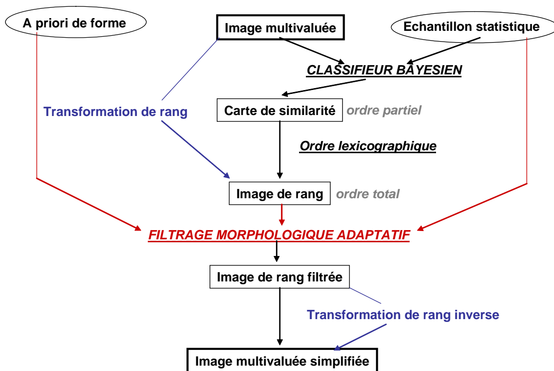
FIG. 2.41: Comment tenir compte de la référence statistique dans l'analyse morphologique d'une image multivaluée.
