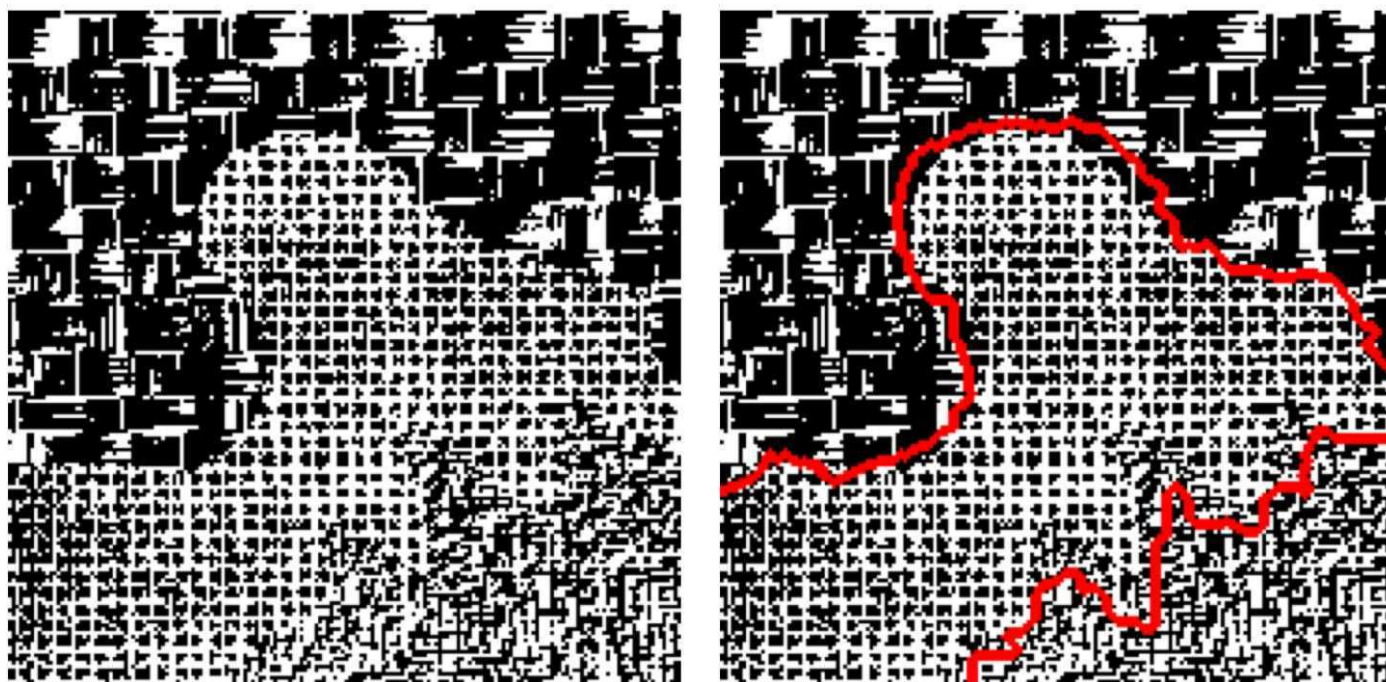
FIG. 2.25: Segmentation d'une texture après décomposition en plusieurs résolutions selon la méthodologie proposée par [42]. L'image segmentée est constituée de vecteurs de dimension 15. Trois marqueurs locaux (quelques pixels) sont positionnés dans les 3 zones d'intérêt.
