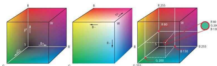
FIG. 1.10: Illustration de la représentation géométrique dans l'espace 3D d'une couleur à partir des composantes RGB. (origine de l'image : wikipedia)
