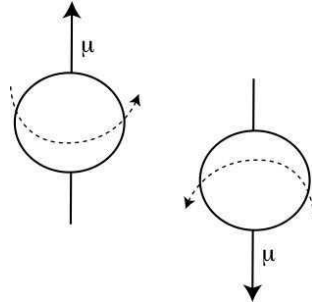
FIG. 3.14: Plongés dans un champ magnétique les protons s'alignent dans la direction du champ magnétique. En fonction de leur spin, les protons ont alors deux configurations possibles : parallèle (Sud Nord) et antiparallèle (Nord Sud).
