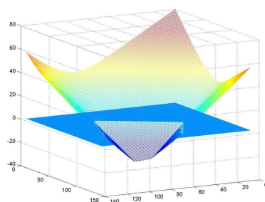
FIG. 3.20: Visualisation de \phi sous un autre angle. Sous cet angle, le contour n'est pas visible, mais nous visualisons correctement la fonction de distance signée. Notons que |\nabla\phi| = 1
