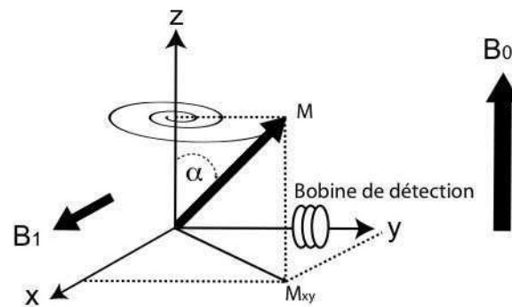
FIG. 3.15: Phase de relaxation : La RF à \omega_0 équivalente à un champ magnétique B_1 augmente l'énergie des protons et déplace l'axe de précession d'un angle \alpha . L'arrêt de la RF permet un retour à l'état initial d'énergie suivant un parcours en spirale. Durant la phase de retour au calme, l'énergie précédemment emmagasinée est libérée ce qui provoque un courant induit récupéré par une bobine de l'IRM.
