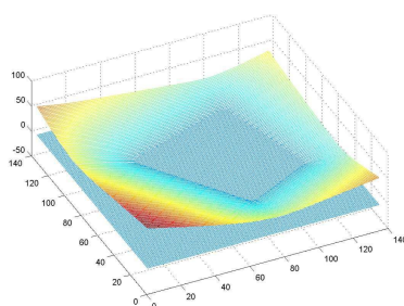
FIG. 3.19: Représentation de la fonction \phi avec son intersection avec le plan de niveau 0. Nous visualisons parfaitement le contour initial C
