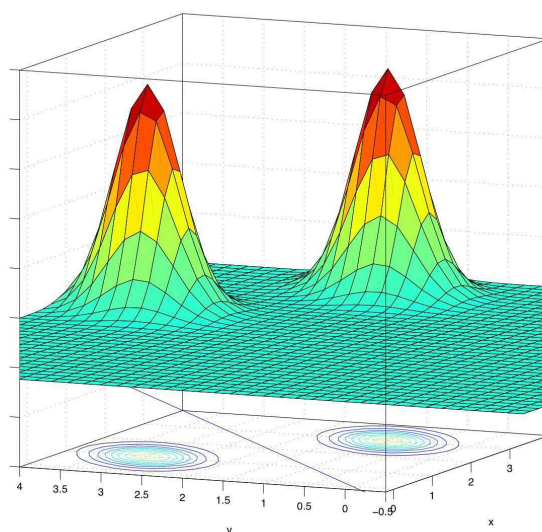
FIG. 2.4: Les paramètres des deux gaussiennes sont \mu_1 = [3; 1] , \mu_2 = [1; 3] et \Sigma_1 = \Sigma_2 = \frac{1}{16}[3, 1; 1, 3] . Le fait que \Sigma ne soit pas diagonale implique que les gaussiennes décrivent au sol non plus des cercles, mais des ellipses. La règle de décision est une droite d'équation : x - y = 0
