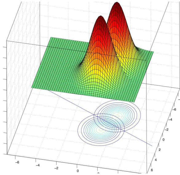
FIG. 2.3: Exemple de deux distributions gaussiennes, dont les moyennes sont \mu_1 = [1; 1] , \mu_2 = [-2, 2] et dont les matrices de covariance sont diagonales \Sigma_1 = \Sigma_2 = [2, 0; 0, 1] . Les gaussiennes décrivent au sol des cercles. La règle de décision est donnée par l'équation de la droite \frac{3}{2}x - y + \frac{9}{4} = 0 qui est perpendiculaire à l'axe reliant les moyennes.
