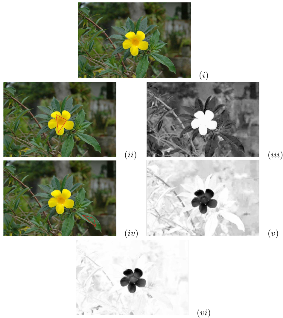
FIG. 2.6: Cartes de similarité associées à une image couleur calculée à partir de la distance de Mahalanobis en utilisant différents échantillons statistiques de référence. Sur les images de similarité, les points de forte luminance localisent les formes statistiquement similaires à l'échantillon de référence tandis que les points de faible luminance sont des points peu ou pas similaires à l'échantillon. (i) est l'image originale. (iii) est l'image des distances associée à la référence (ii) (l'échantillon est la région délimitée en rouge sur l'image (ii)). (iv) est la carte des distances associée à la référence (v) et (vi) est la carte des distances obtenue en prenant comme référence un blanc le blanc (après ajout d'un bruit gaussien). Sur les cartes des distances, les structures de l'image sont ordonnées selon leur similarité à l'échantillon de référence.
