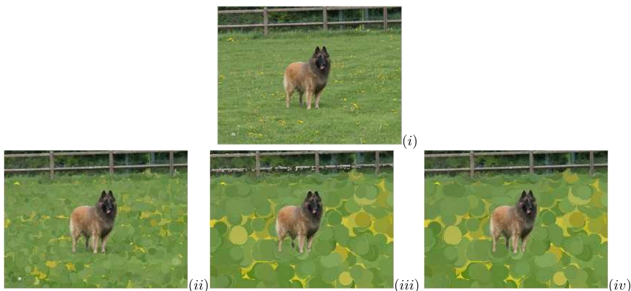
FIG. 2.52: (i) est l'image originale. L'échantillon de référence est pris dans le chien (voir figure 2.40). (ii) et (iii) sont les résultats d'ouvertures visqueuses de taille 5 et 10, l'activité r(h) est une fonction linéaire de h : r(h) = R \left[ 1 - \frac{h}{N-1} \right] . (iv) est le résultat obtenu par ouverture visqueuse de taille 10, l'activité étant cette fois une fonction à variations plus lentes pour les très fortes et très faibles similarités : r(h) = R \left[ 1 - \frac{h}{N-1} \right]^{\frac{5}{2}} \left[ 1 + \frac{h}{N-1} \right]^{\frac{5}{2}}
