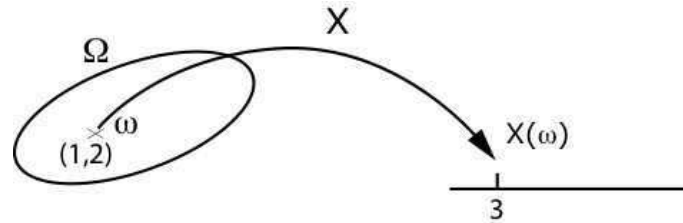
FIG. 1.8: Une variable aléatoire est une application X de \Omega dans \mathbb{R} . Dans l'exemple ci-dessus d'un lancer de deux dés, nous nous intéressons à la somme. La variable aléatoire associe à chaque événement \omega une valeur dans [2; 12] .
