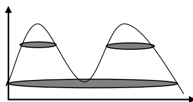
FIG. 2.43: Décomposition d'une fonction à valeurs scalaires en ensembles de niveau.
