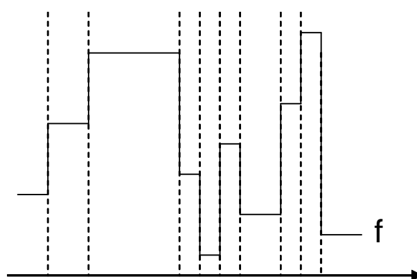
FIG. 2.10: Une fonction constante par morceaux et sa partition en zones plates.
