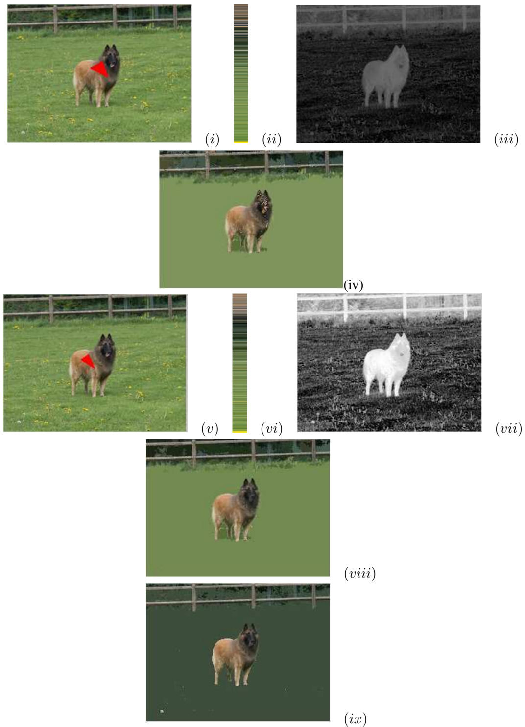
FIG. 2.54: Tests avec FAS visqueux par reconstruction : (iv) et (viii). L'élément structurant est un disque euclidien de taille (maximale) 20. L'activité suit une loi de type sigmoïde. Les résultats ont été obtenus pour deux échantillons de référence différents (voir (i) et (v)). (ix) a été obtenue par simple seuillage de l'image de rang.
