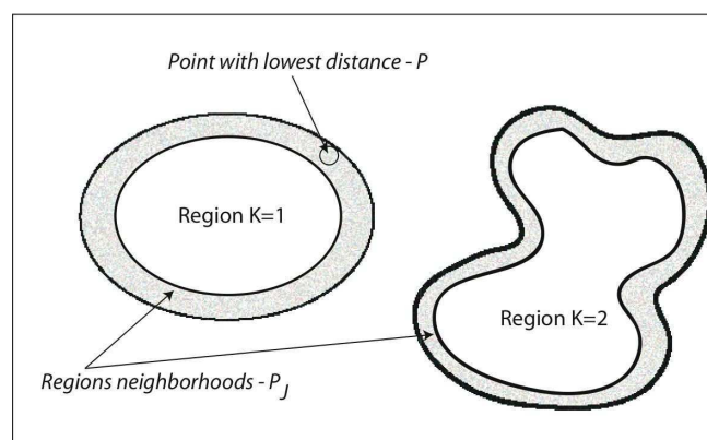
FIG. 2.20: Modification du protocole de croissance de région dans le cas où chaque source définit une référence statistique. Chaque région grossit à un rythme fixé par la distance statistique des points libre à la source.
