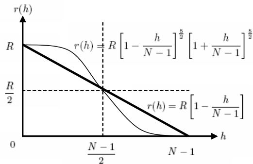
FIG. 2.47: Deux exemples de relation de dépendance entre l'activité du filtre r(h) et le rang (ou similarité) h .
