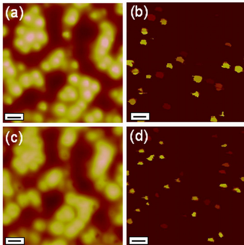
FIG. 3.10 – Images topographiques et électriques d'une zone de 5 \times 5 \mu\text{m}^2 en appliquant une force de (a, b) 120 nN et (c, d) 2,8 \mu\text{N} . Les corrections apportées sur la planéité des images (a) et (c) après acquisition sont les mêmes. Échelles 500 nm.
