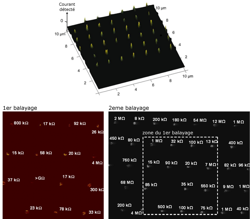
FIG. 3.25 – (Haut) cartographie en vue 3D montrant la détection du courant, localisée au niveau des vias. (Bas) Images électriques donnant les valeurs de résistances associées à chaque via lors du premier balayage et deuxième balayage (la zone couverte lors du second balayage est plus large, le carré en pointillés représente celle balayée la première fois).
