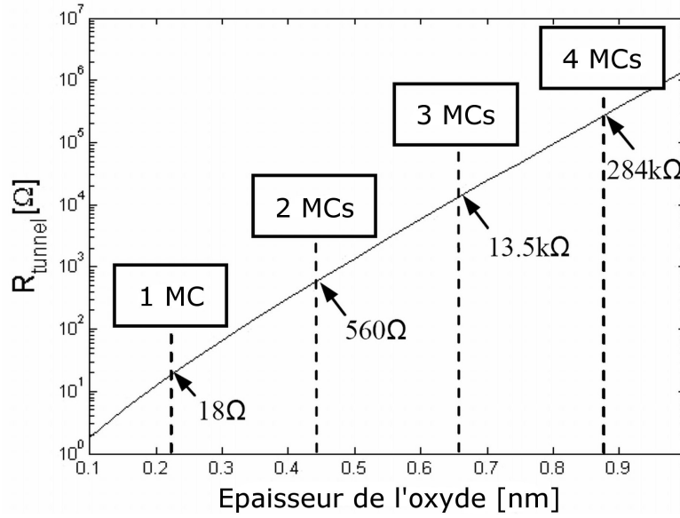
FIG. 3.19 – Tracé de la résistance tunnel en fonction de l'épaisseur d'oxyde pour un rayon de contact de 40 nm, calculée à partir de la formule de Simmons. Les résistances sont données par nombre de monocouches (MCs).
