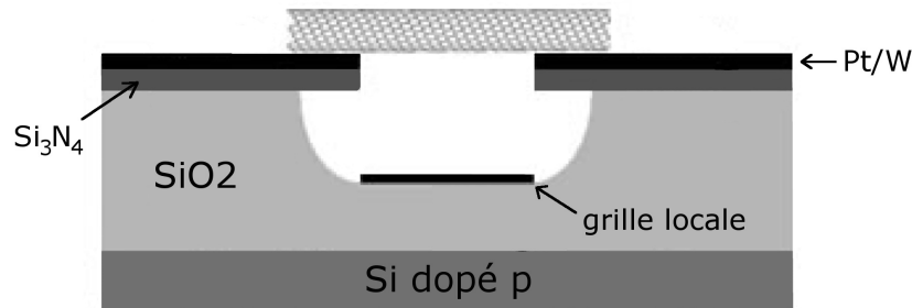
FIG. 5.4 – Schéma représentant la structure. Le catalyseur n'est pas représenté sur les électrodes. Adapté de [67].
