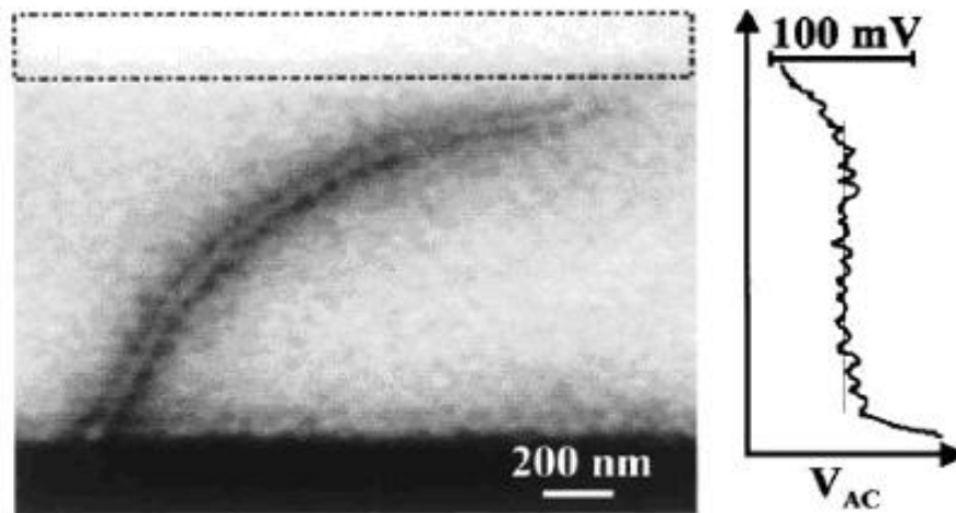
FIG. 1.29 – Image de microscope à force électrostatique et profil de potentiel d'un fagot de nanotubes métalliques de résistance totale 40\text{ k}\Omega et de résistance intrinsèque 3\text{ k}\Omega .
