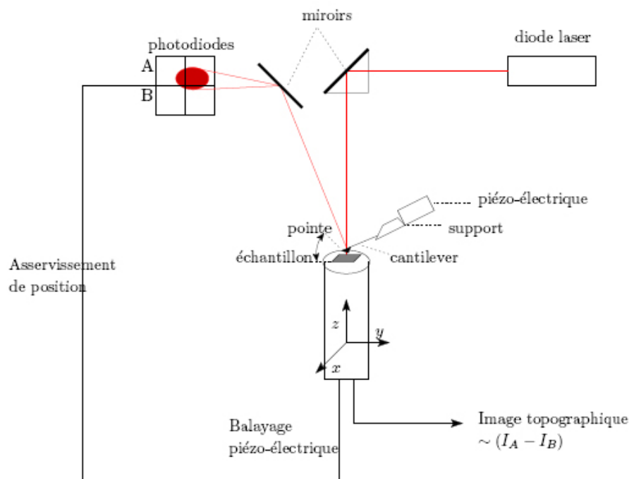
FIG. 3.1 – Principe de fonctionnement d'un microscope à force atomique
