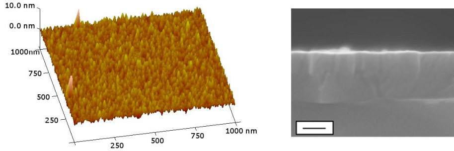
FIG. 3.13 – (Gauche) Représentation 3D d'une surface de 1 \mu\text{m} de côté balayée à l'AFM – acquisition faite en mode tapping. (Droite) Image MEB en coupe d'un échantillon Si / Ti (40 nm) / TiN (60 nm). Échelle 50 nm.
