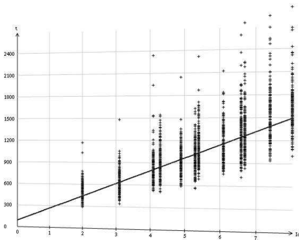
Figure 28 : Régression linéaire (empruntée à [Raynal et Serrurier, 2007]).
