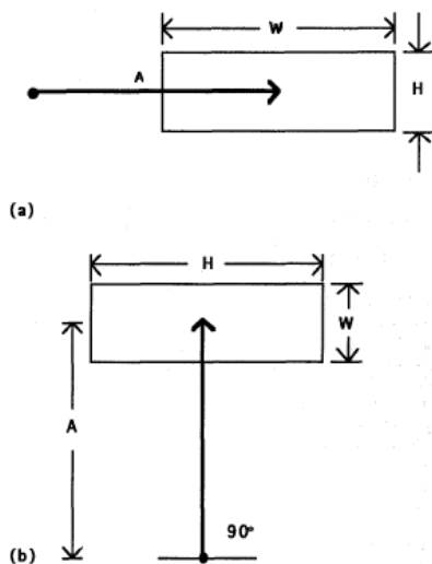
Figure 22: Atteinte de cible selon la direction verticale et horizontale méréule, empruntée à [MacKenzie, 1992]
