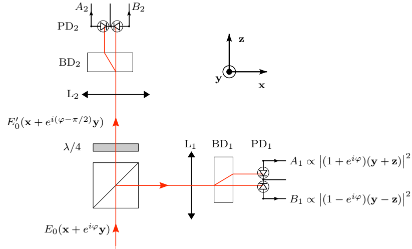
FIGURE 2.5 – Le faisceau lumineux provenant de la région de mesure est séparé en deux par un cube séparateur non polarisant. Dans chaque bras d'analyse une lame de calcite de 5 mm d'épaisseur ( BD_1 et BD_2 ) projette les composantes de la polarisation à 45^\circ afin d'obtenir les interférences. Chaque composante est focalisée (lentilles L_1 et L_2 ) sur une photodiode ( PD_1 et PD_2 ) pour en enregistrer l'intensité ( A_1 , A_2 , B_1 et B_2 ). Dans le deuxième bras d'analyse une lame au quart d'onde ( \lambda/4 ) ajoute une phase \psi_2 = -\pi/2 à la phase initiale \varphi .
