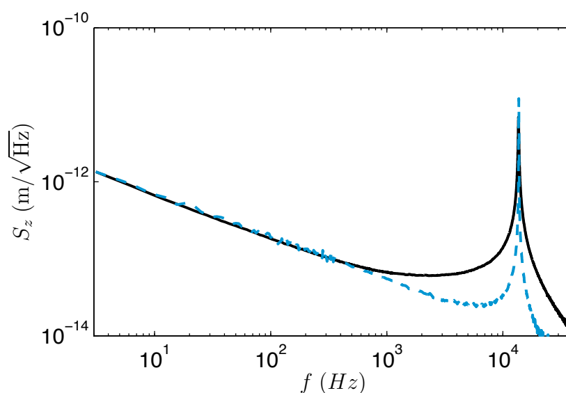
FIGURE 5.7 – Levier avec revêtement en or DSP mesurée à pression atmosphérique (ligne continue) et à 3 \times 10^{-5} mbar de pression (ligne en pointillé long).
