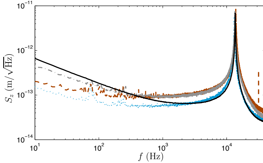
FIGURE 5.5 – DSP des fluctuations thermiques pour différents leviers : levier en silicium ( \cdots ), avec revêtement en platine ( - ), avec revêtement en aluminium ( \cdot- ) et avec revêtement en or (trait continu).
