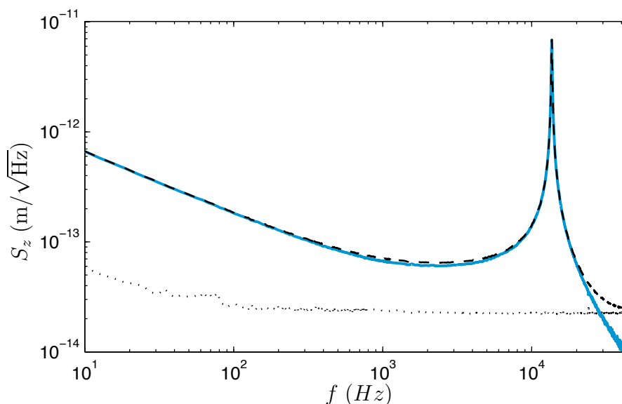
FIGURE 5.3 – En soustrayant à la mesure de la DSP des fluctuations thermiques d'un levier en silicium avec revêtement en or (—) le bruit de fond de l'appareil ( \cdots ), on obtient le spectre du signal thermique sur tout l'intervalle de fréquence représenté (—). On remarque que la partie basse fréquence du spectre n'est pas affectée par le bruit de fond.
