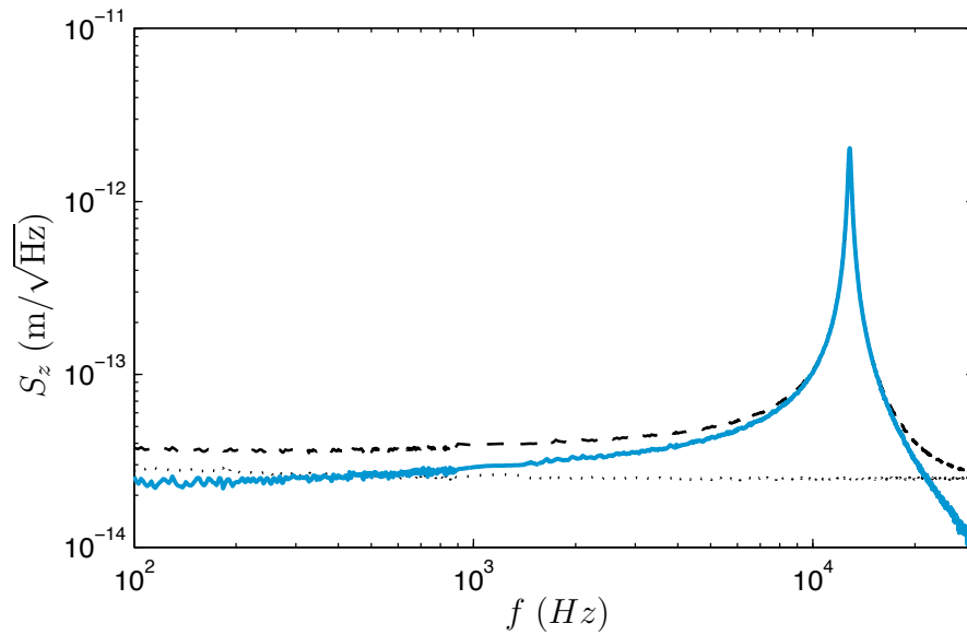
FIGURE 5.1 – En soustrayant à la mesure de la DSP des fluctuations thermiques d'un levier en silicium (--) le bruit de fond de l'appareil (· · ·), on obtient le spectre du signal thermique sur tout l'intervalle de fréquence représenté (—).
