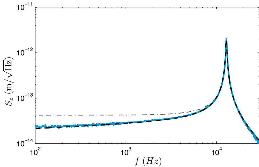
FIGURE 5.1 – En soustrayant à la mesure de la DSP des fluctuations thermiques d'un levier en silicium (--) le bruit de fond de l'appareil (· · ·), on obtient le spectre du signal thermique sur tout l'intervalle de fréquence représenté (—).
