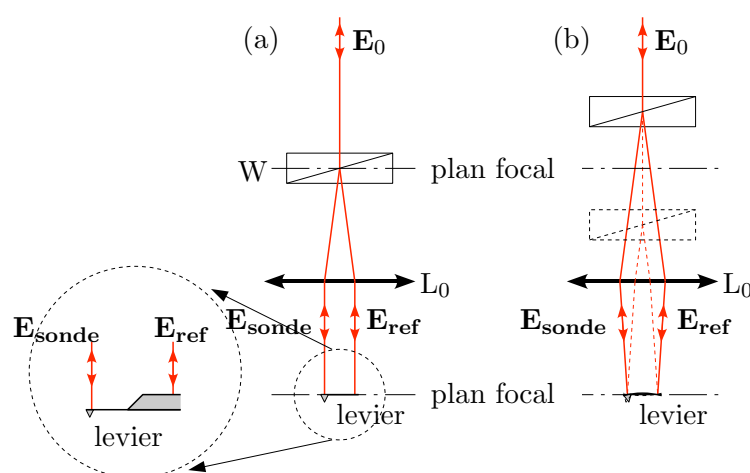
FIGURE 2.4 – (a) Le prisme de Wollaston W sépare le rayon incident \mathbf{E}_0 en deux faisceaux de polarisation orthogonales ( \mathbf{E}_{\text{ref}} et \mathbf{E}_{\text{sonde}} ). Suite au passage dans la lentille de focalisation L_0 et au positionnement du prisme de Wollaston à la distance focale de la lentille, on obtient \mathbf{E}_{\text{ref}} et \mathbf{E}_{\text{sonde}} parallèles, avec une distance relative de 1 mm (lentille L_0 de focale 30 mm et prisme de Wollaston W de divergence 2^\circ ). (b) Le réglage de la distance entre le Wollaston et la lentille permet de compenser une faible courbure du levier.
