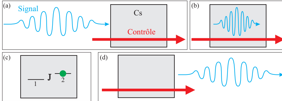
FIG. 6.9 – Représentation schématique du fonctionnement d'une séquence mémoire. (a) Après avoir pompé les atomes dans le niveau 2, le champ de contrôle et l'impulsion signal sont envoyés dans les atomes. (b) Le signal est ralenti dans la vapeur de césium par le phénomène d'EIT engendré par le champ de contrôle, et les fluctuations du signal sont transférées au spin collectif transverse des atomes. (c) Le champ de contrôle est alors éteint et les informations quantiques sont stockées dans les fluctuations du spin collectif. (d) Après un certain temps, le champ de contrôle est rallumé, ce qui crée de nouveau une fenêtre d'EIT. Les fluctuations du spin sont transmises à la lumière qui ressort sous forme d'un signal ayant les mêmes propriétés quantiques que le signal d'entrée.
