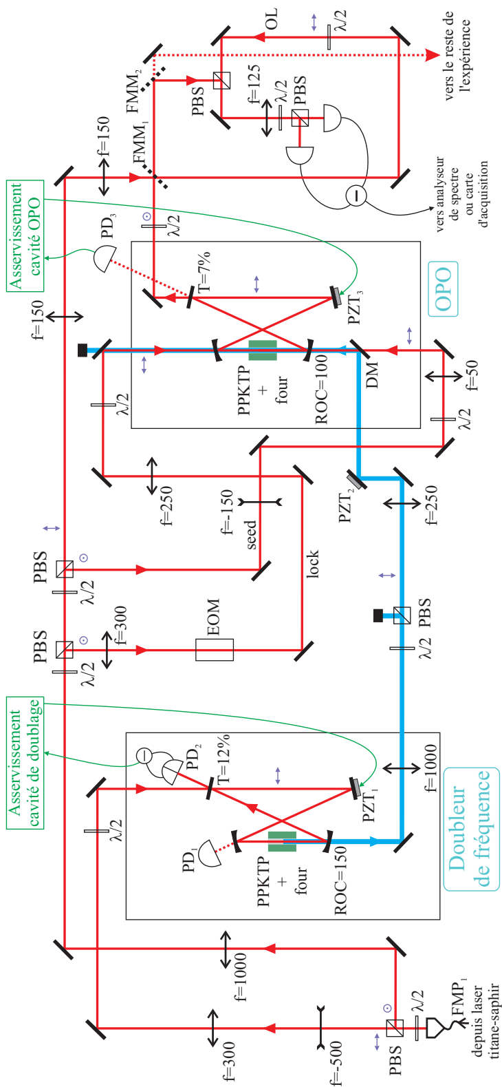
FIG. 4.1 – Schéma du dispositif expérimental composé d'un doubleur de fréquence et d'un oscillateur paramétrique optique permettant de produire des états comprimés (FMP : fibre monomode à maintien de polarisation, DM : miroir dichroïque, FMM : miroir escamotable, seed : faisceau signal source pour l'OPO, lock : faisceau servant à l'asservissement de l'OPO, OL : oscillateur local).
