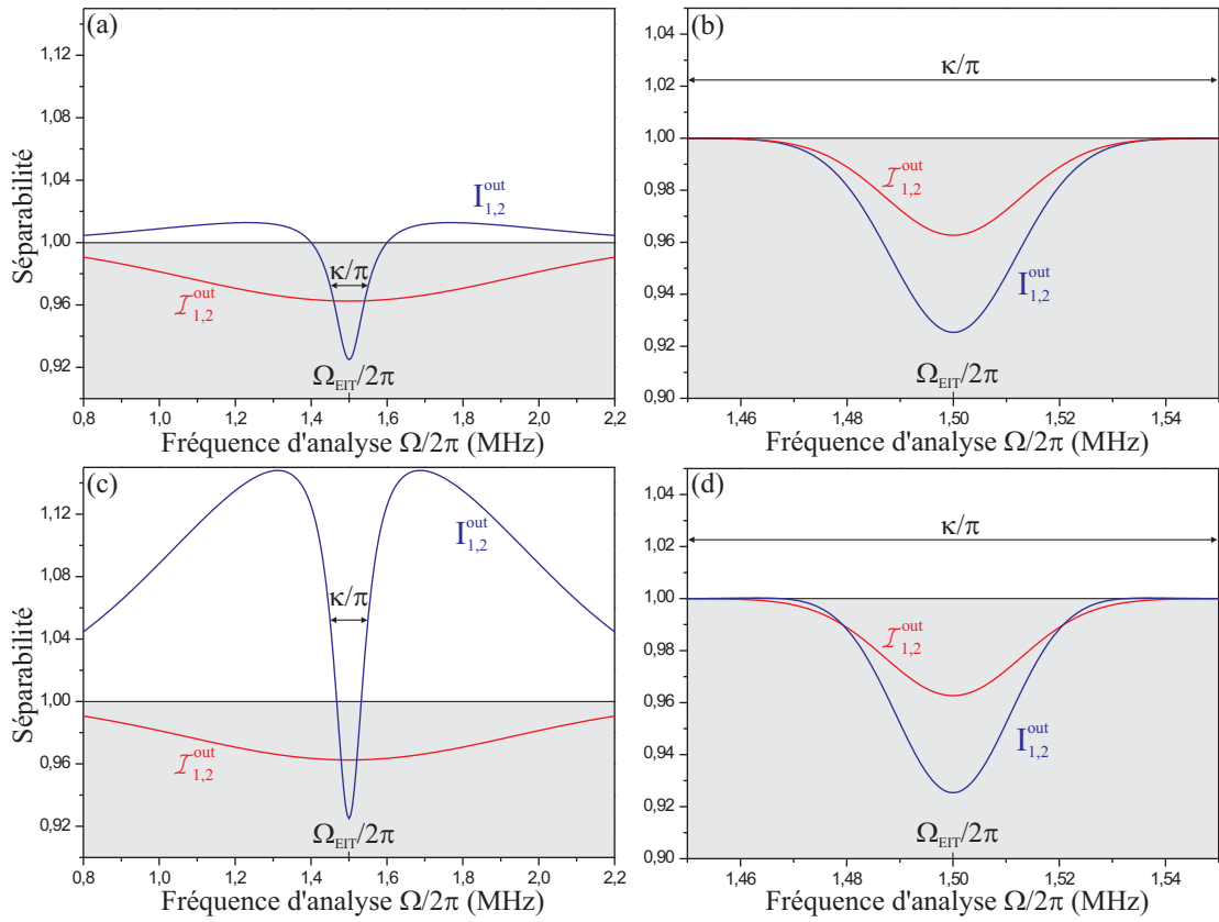
FIG. 5.8 – Comparaison de la séparabilité des faisceaux à la sortie des atomes dans le cas où le dispositif de séparation spatiale est la lame semi-réfléchissante ( \mathcal{I}_{1,2}^{out} ) ou la cavité ( I_{1,2}^{out} ), pour un état incident comprimé selon la quadrature X . La région grisée indique la zone où les faisceaux sont intriqués (séparabilité inférieure à 1). Taux de compression : 3 dB ( s = 0,5 ), (a) et (b) état comprimé minimal, (c) et (d) état comprimé avec 8 dB d'excès de bruit sur la quadrature Y . Paramètres communs aux 4 figures : désaccord cavité - porteuse du signal : \Delta/2\pi = 1,5 MHz, bande passante de la cavité : \kappa/\pi = 100 kHz, \kappa_L = 0 , fenêtre d'EIT de l'ensemble atomique 1 centrée à \Omega_{EIT,1}/2\pi = -1,5 MHz et fenêtre d'EIT de l'ensemble atomique 2 centrée à \Omega_{EIT,2}/2\pi = 1,5 MHz, transparence des fenêtres d'EIT : 30 % en intensité. Paramètres des figures (a) et (c) ((b) et (d)) : fenêtre d'EIT de largeur totale à mi-hauteur de 1 MHz (respectivement 30 kHz).
