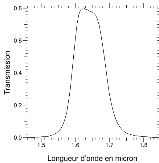
FIG. 3.4 – Transmission du filtre étroit en bande H utilisé pour les données de Bételgeuse.
