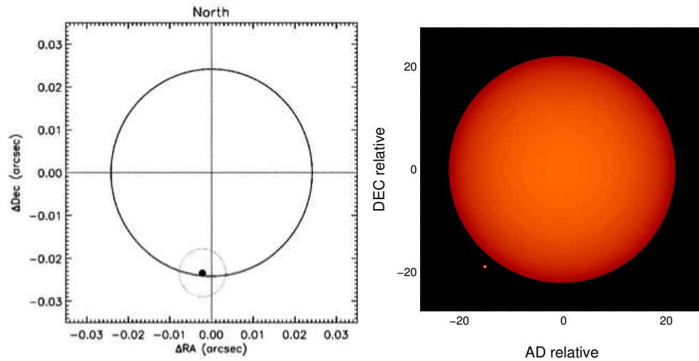
FIG. 4.12 – Gauche : Modèle de disque uniforme de 48,4 milli-secondes d’angle ajusté aux données de Bételgeuse à 11,15 \mu\text{m} fin 2006. Un point situé sur le bord Sud du disque et représentant 5,3% du flux total rend compte des clôtures de phase observées. Extrait de Tatebe et al. (2007). Droite : Imagerie paramétrique de Bételgeuse d’après l’exploitation de données interférométriques obtenues à 1,65 micron au mois d’Octobre 2005. Bételgeuse est représentée par un disque assombri d’une taille angulaire de 44,3 milli-secondes d’angle entourée d’un environnement. Les clôtures de phase indiquent la présence d’une structure localisée d’1 milli-seconde d’angle de diamètre et proche du bord Sud-Est de la photosphère. Elle contribue à 1% du flux total observé.
