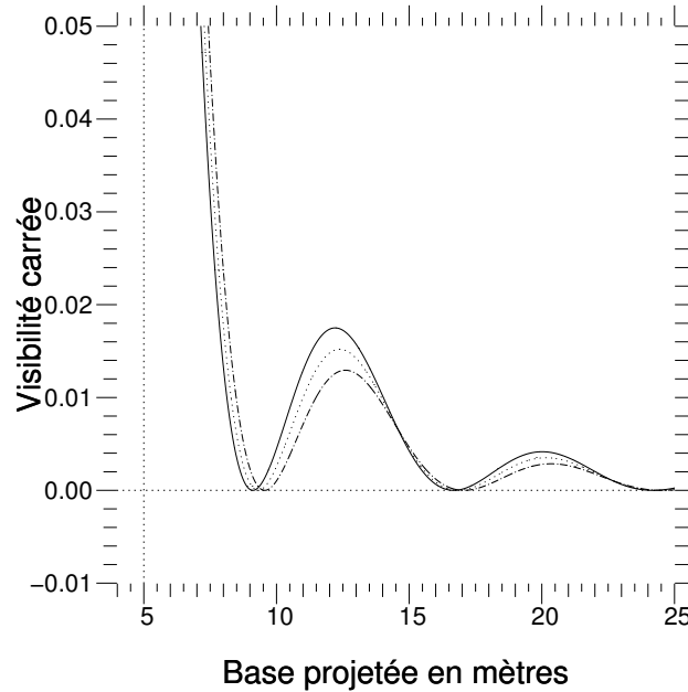
FIG. 4.6 – Visibilités carrées pour un disque uniforme (en continu) et des disques linéairement assombrissants ( A = 0,2 en pointillés et A = 0,4 en trait-point). Voir le texte pour la signification de A .
