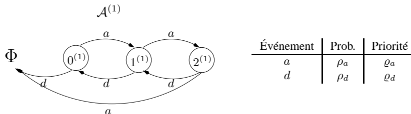
FIG. 6.5 – File d'attente avec arrivée et départ pour n = 0
