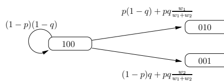
FIG. 6.3 – Graphe de marquage du modèle de FIG. 6.1 selon Ciardo
