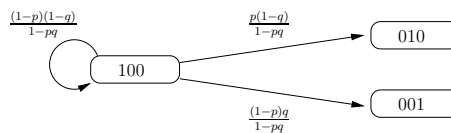
FIG. 6.2 – Graphe de marquage du modèle de FIG. 6.1 selon Molloy
