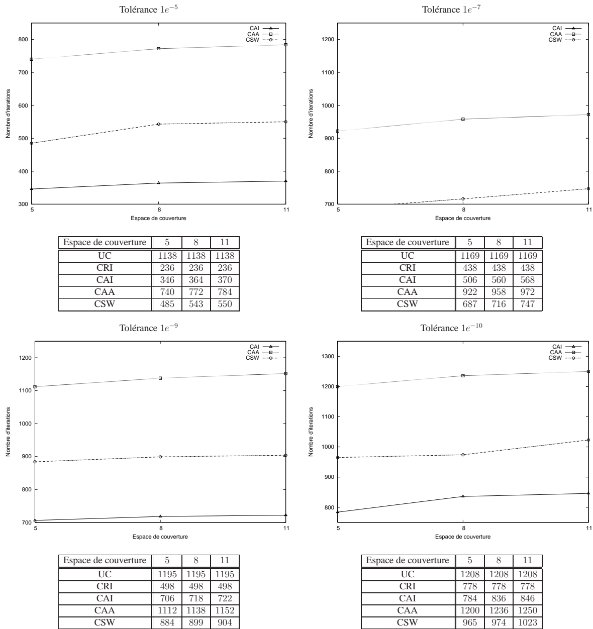
FIG. A.15 – RWP - Nombre d'itérations pour différentes aires de couverture
