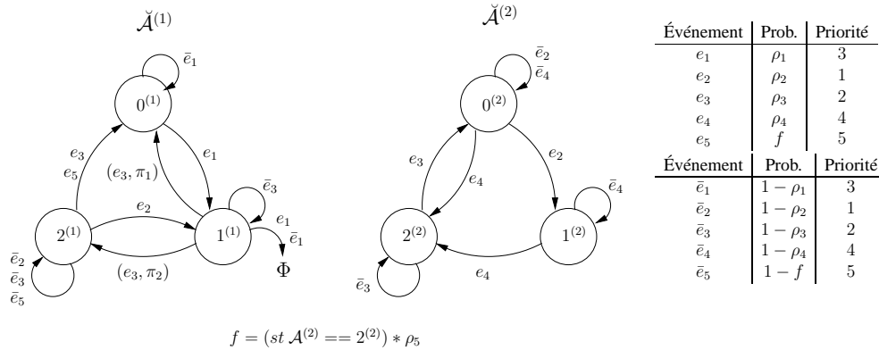
FIG. 6.12 – Représentation graphique d'un réseau d'automates complétés du modèle SAN de FIG. 6.11
