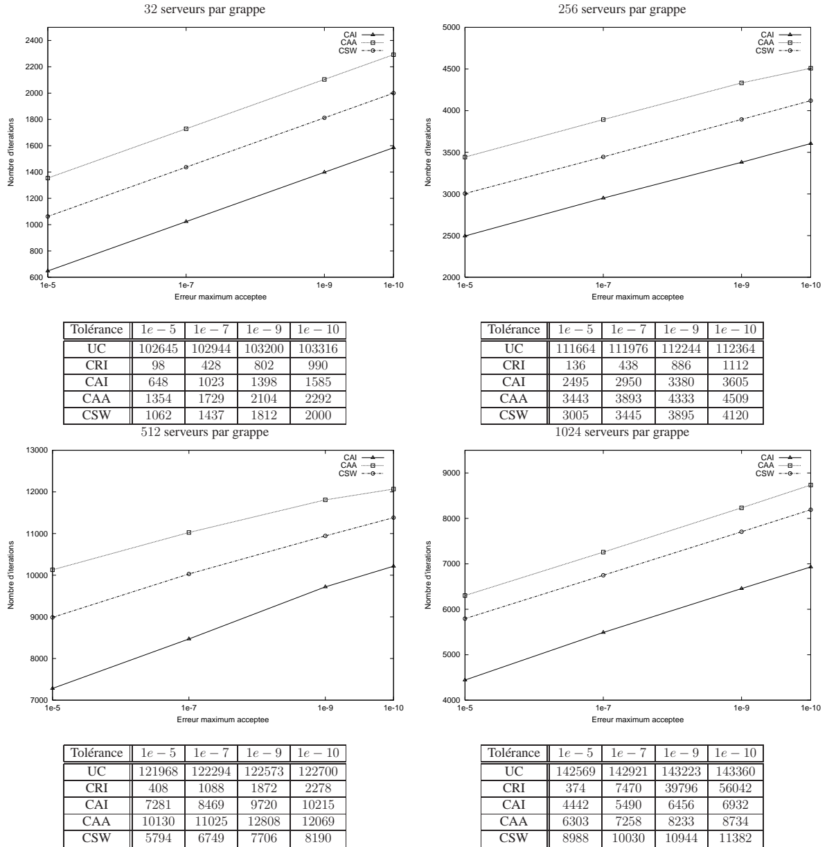
FIG. A.36 – WORKSTATION (90% des serveurs disponibles) - Nombre d'itérations pour différentes erreurs maximum acceptées
