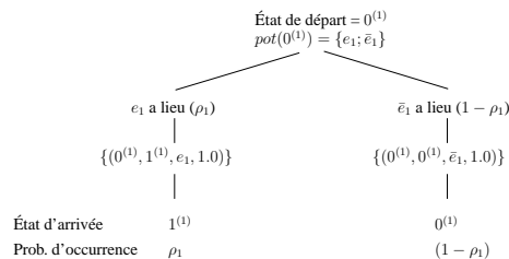
FIG. 6.7 – Construction des chaînes de transitions globales pour l'état 0^{(1)} de l'automate \check{\mathcal{A}}^{(1)}
