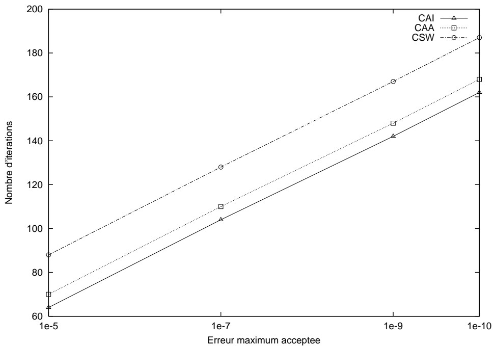
FIG. 5.3 – MSA- 256 serveurs
