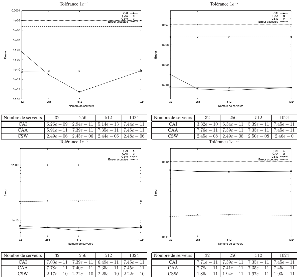
FIG. A.21 – WORKSTATION (10% des serveurs disponibles) - Précision des résultats pour différents nombres de serveurs
