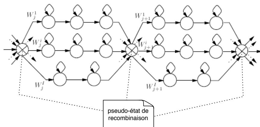
FIG. 3.3: HMM comportant des pseudo-états de recombinaison.
