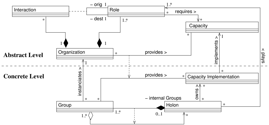
FIG. 5.2 – Méta-modèle CRIO
