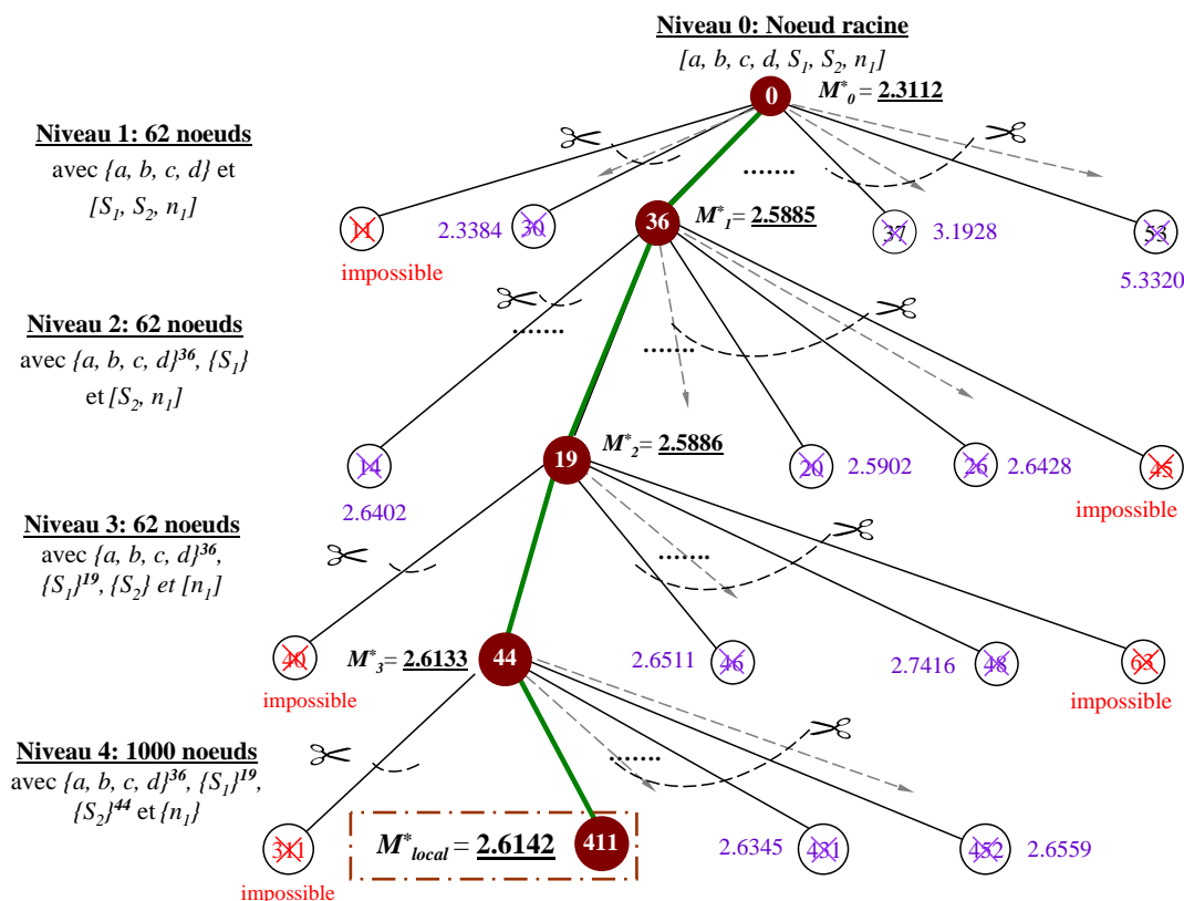
FIG. 4.19 – Arborescence de la première descente de l'algorithme BB. [ ] et \{ \} indiquent respectivement les variables continues et discrètes. Le successeur de chaque niveau est désigné par M_m^n ( |^n est le nombre de branches; |_m est le niveau de l'arbre).
