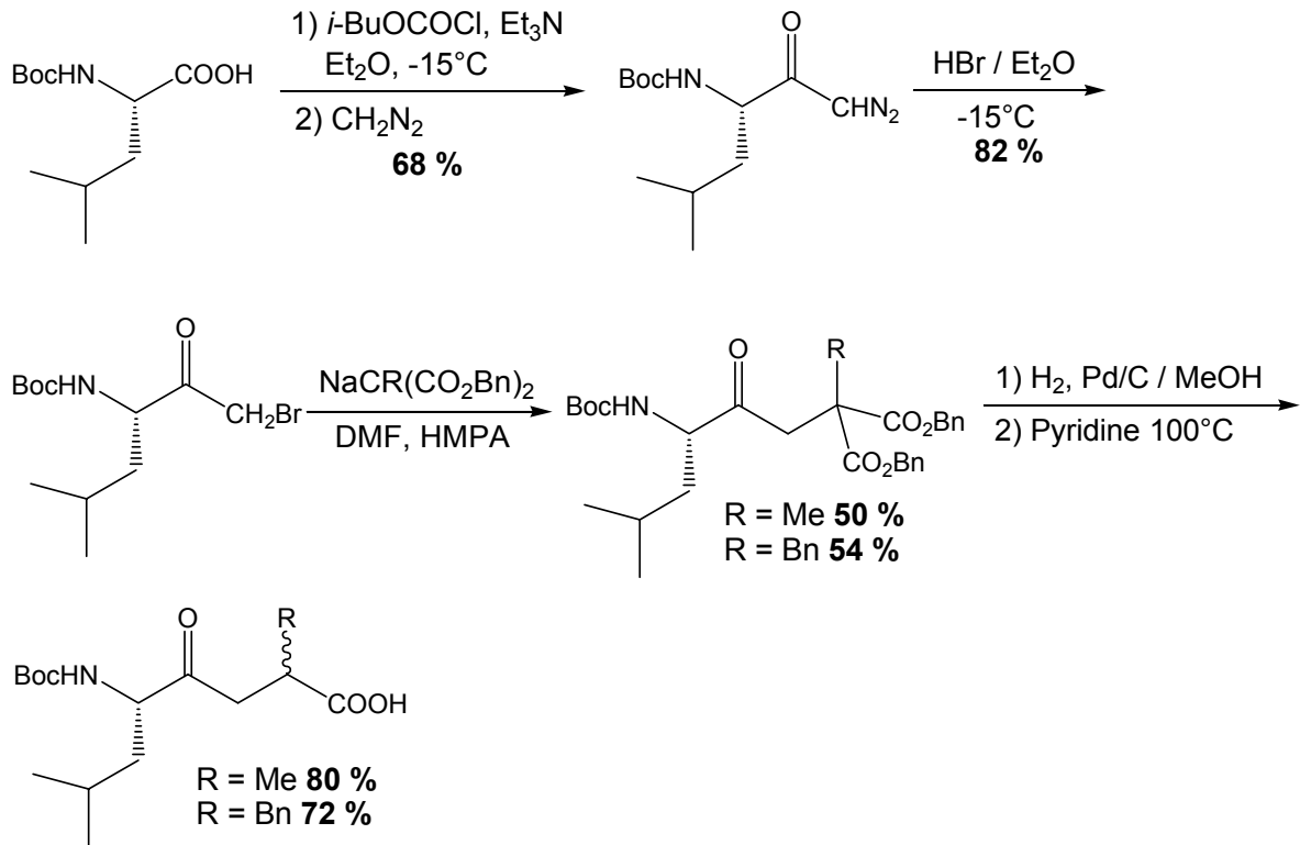
Schéma 37 : synthèse via un malonate
