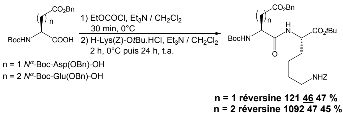
Schéma 82 : synthèse des réversines 121 et 1092
