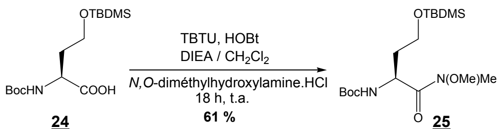
Schéma 60 : préparation de l'amide de Weinreb
