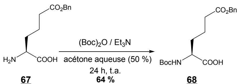
Schéma 100 : synthèse du N^\alpha -Boc-Aad(OBn)-OH
