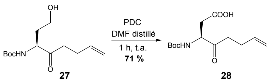
Schéma 63 : oxydation de l'alcool par le PDC
