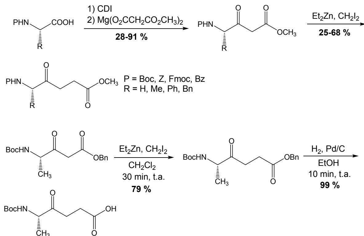
Schéma 36 : synthèse par réaction d'un carbénoïde sur un β-cétoester
