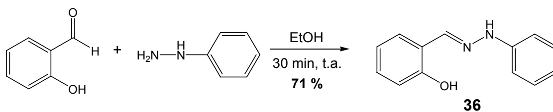
Schéma 70 : synthèse de la phénylhydrazone dérivée de l'aldéhyde salicylique
