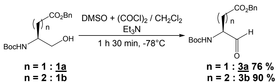
Schéma 19 : préparation de l'aldéhyde par la méthode de Swern
