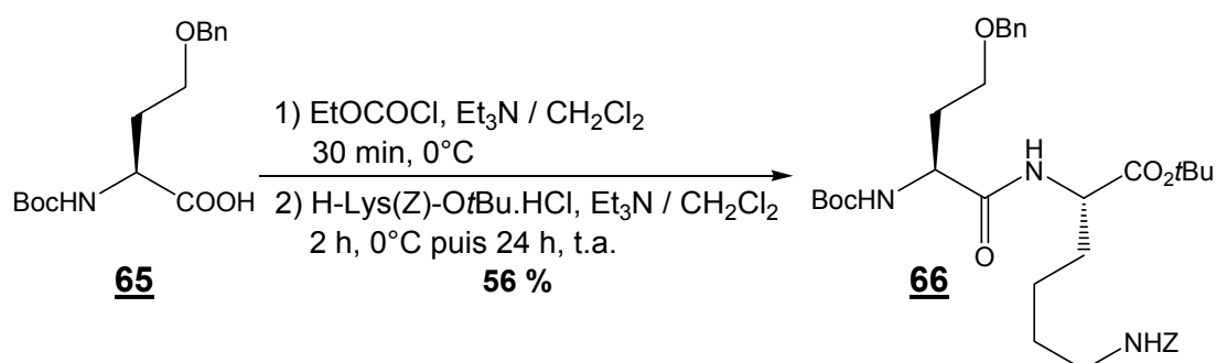
Schéma 98 : synthèse du N^\alpha -Boc-Hse(Bn)-Lys(Z)-OtBu
