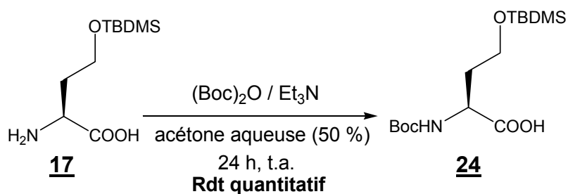
Schéma 59 : protection de l'amine
