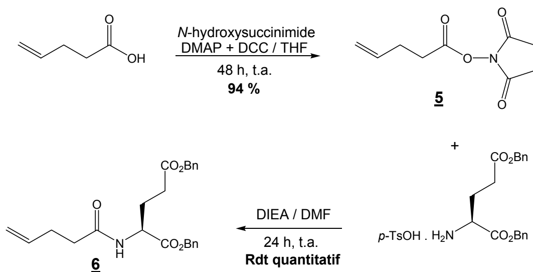
Schéma 21 : couplage de l'acide pent-4-énoïque avec le H-Glu(OBn)-(OBn). p -TsOH
