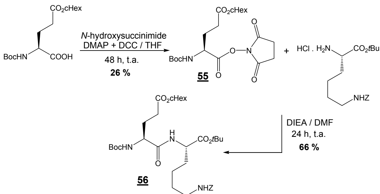
Schéma 87 : synthèse du N^\alpha -Boc-Glu(OcHex)-Lys(Z)-OtBu
