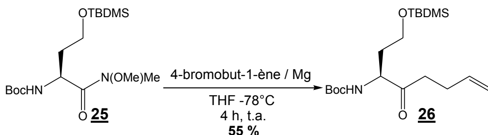
Schéma 61 : obtention du cétoéthylène par la réaction de Grignard
