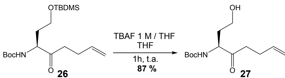
Schéma 62 : déprotection de l'alcool par le TBAF
