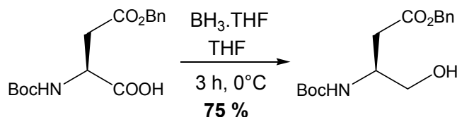
Schéma 5 : préparation de l'α-aminoalcool en une étape
