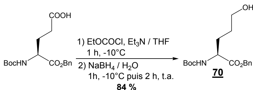
Schéma 102 : synthèse de la N^\alpha -Boc-Nva( \delta -OH)-OBn
