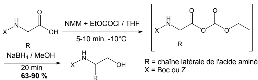
Schéma 6 : préparation de l'alcool en deux étapes « one-pot »
