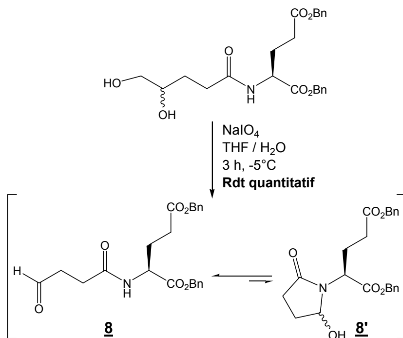
Schéma 23 : formation de l'aldéhyde
