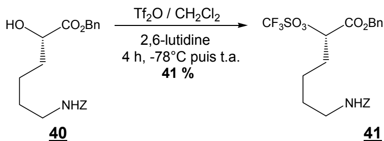
Schéma 79 : synthèse du triflate selon Thierry et coll.
