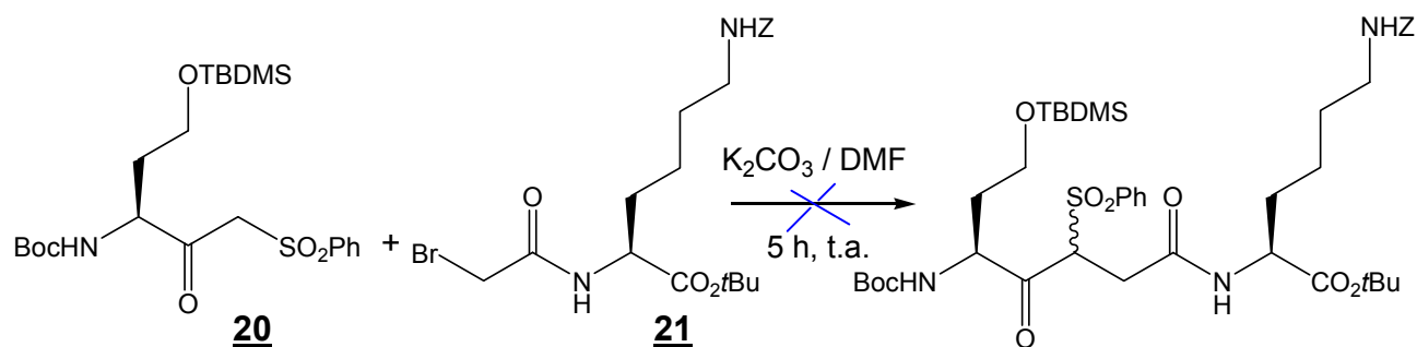
Schéma 54 : couplage de la β-cétosulfone avec le dérivé bromé de la lysine
