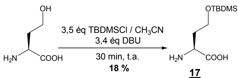
Schéma 47 : protection de l'alcool de la L-homosérine
