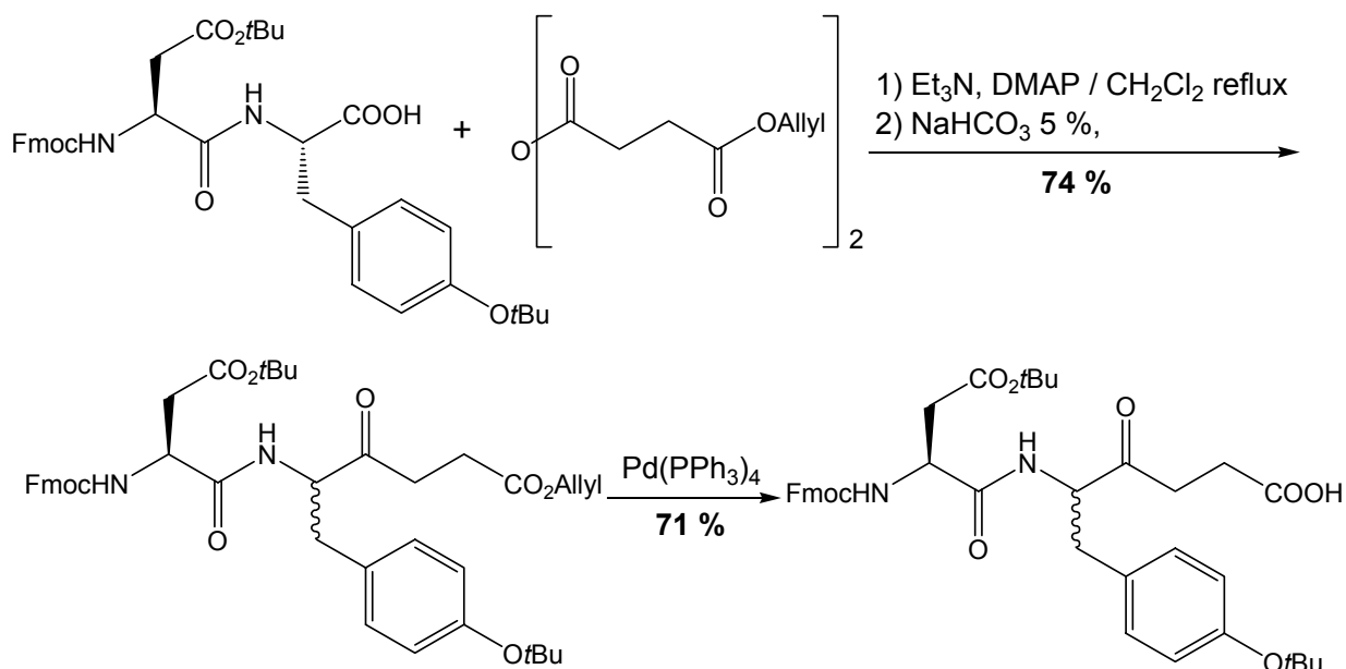
Schéma 34 : synthèse par réaction de Dakin-West
