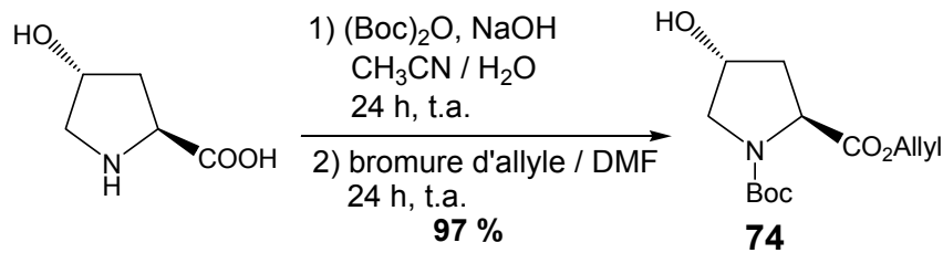
Schéma 106 : synthèse de la N^\alpha -Boc- trans -4-Hyp-OAllyl
