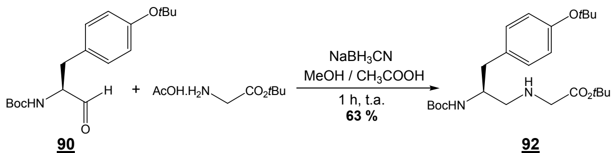
Schéma 123 : synthèse du N^\alpha -Boc-Tyr( t Bu)- \psi (CH 2 -NH)-Gly- Ot Bu
