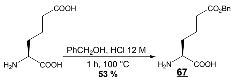
Schéma 99 : synthèse du H-Aad(OBn)-OH
