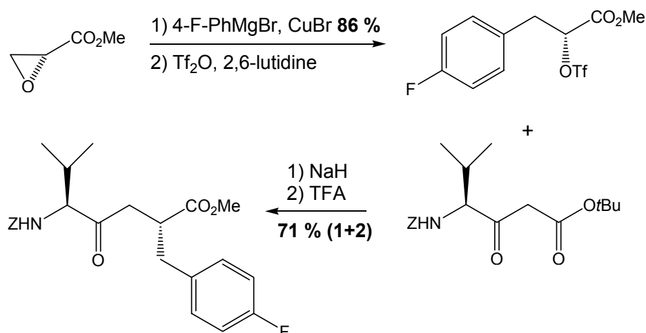
Schéma 42 : SN2 entre un triflate et un β-cétoester tert -butylique
