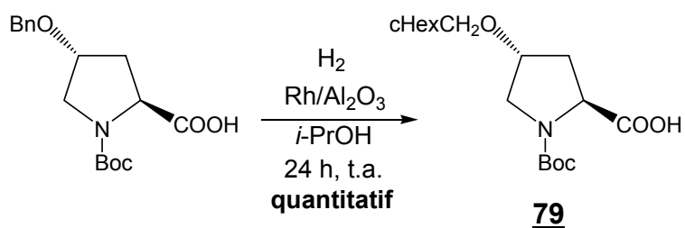
Schéma 111 : synthèse de la N^\alpha -Boc- trans -4-Hyp(CH 2 cHex)-OH
