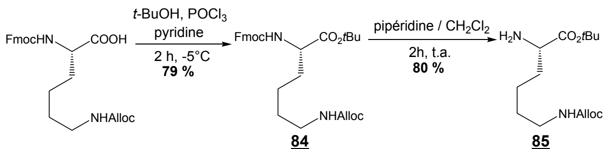
Schéma 116 : synthèse de la H-Lys(Alloc)-OtBu
