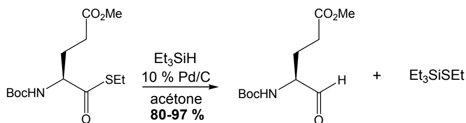
Schéma 4 : réduction du thioester
