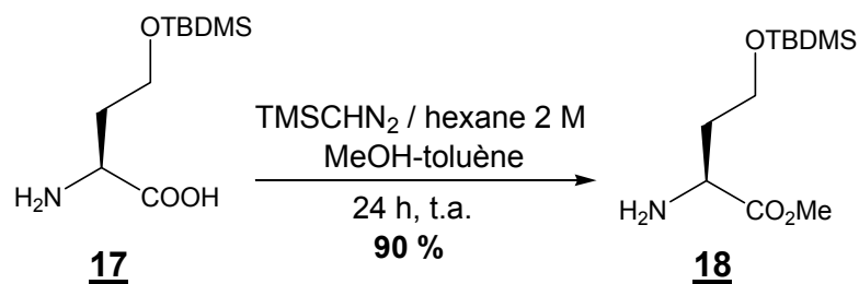
Schéma 50 : estérification avec le TMSCHN 2
