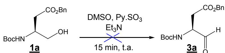
Schéma 18 : préparation de l'aldéhyde par la méthode de Doering
