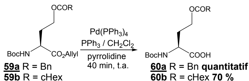
Schéma 92 : préparation de la N^\alpha -Boc-Hse(COBn)-OH
