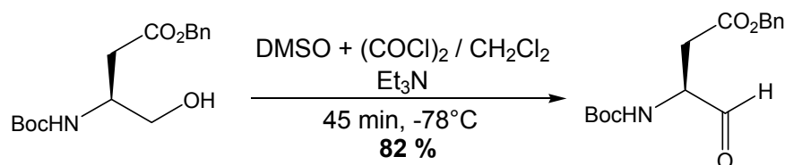
Schéma 9 : préparation de l'aldéhyde par la méthode de Swern
