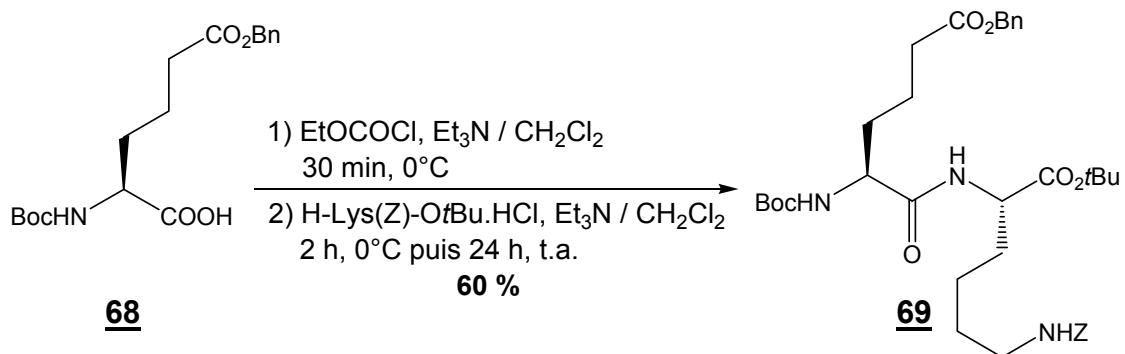
Schéma 101 : synthèse du N^\alpha -Boc-Aad(OBn)-Lys(Z)-OtBu
