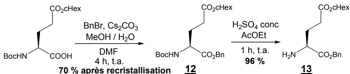
Schéma 27 : synthèse du H-Glu(OcHex)-OBn
