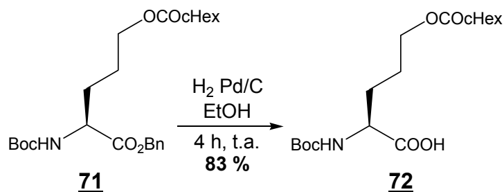
Schéma 104 : synthèse de la N^\alpha -Boc-Nva( \delta -OCOCHex)-OH
