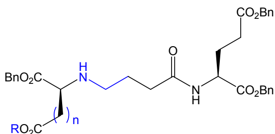
Analogues « monoréduits » de la réversine 213 n = 1 R = Bn n = 2 R = Dmp, cHex
