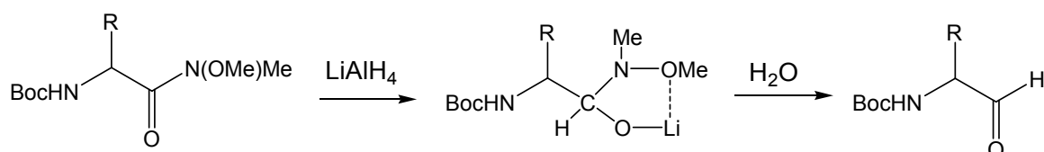
Schéma 3 : réduction de l'amide de Weinreb
