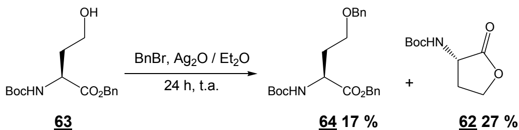
Schéma 96 : synthèse de la N α -Boc-Hse(Bn)-OBn
