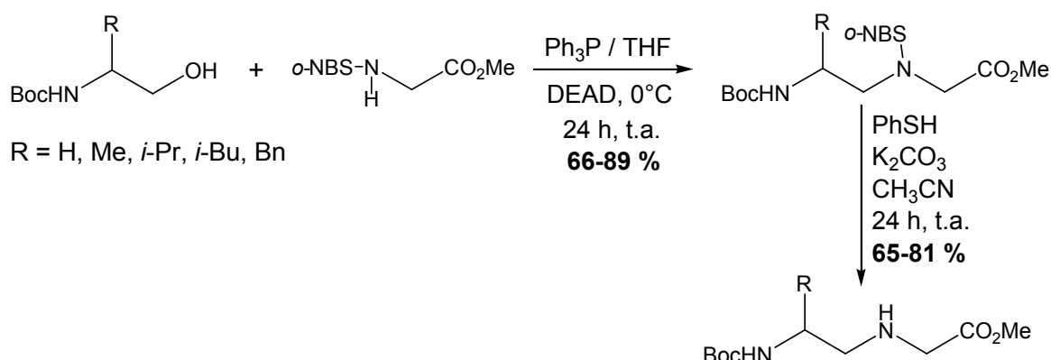
Schéma 14 : réaction de Mitsunobu
