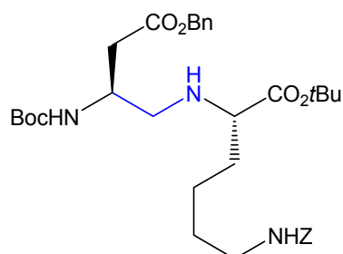
Analogue « réduit » de la réversine 121 N^{\alpha} -Boc-Asp(OBn)- \psi (CH 2 -NH)-Lys(Z)-OtBu
