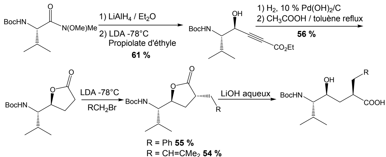
Schéma 44 : synthèse via une lactone
