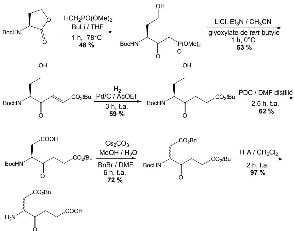
Schéma 35 : synthèse via un cétophosphonate
