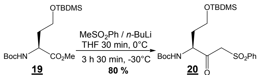
Schéma 52 : préparation de la β-cétosulfone
