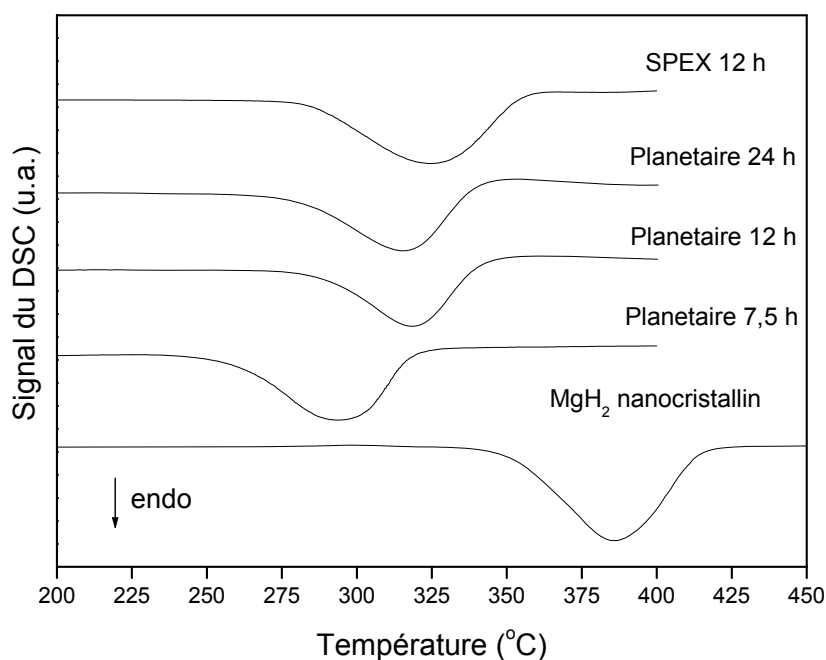
Figure 6 Courbes de DSC d'échantillons sélectionnés, préparés par broyage réactif de mélanges 2Mg-Fe (40:1, 3 MPa de H_2 ). Le type de broyeur et le temps de broyage sont indiqués. Le courbe pour le MgH_2 nanocristallin est montré pour comparaison.
