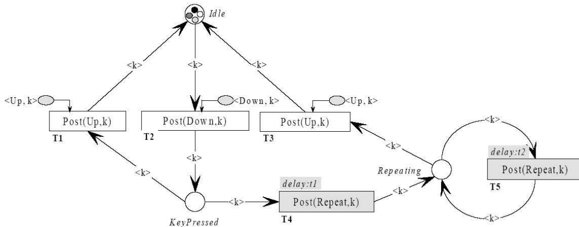
FIG. 2.11 – Un comportement bas-niveau du clavier (répétition de touches) décrit avec une variante élaborée de réseau de Petri [Accor et al. 97].
