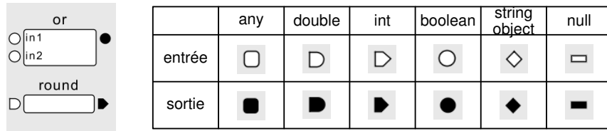
FIG. 3.11 – À gauche, un ou logique comportant deux booléens en entrée et un booléen en sortie, et un dispositif d'arrondi qui transforme un réel (double) en un entier. À droite, les différents types de slots.
