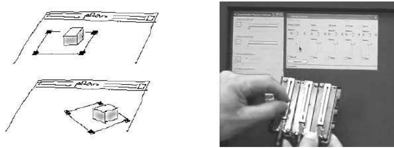
FIG. 1.26 – À gauche : interface « saisissable » , où des briques physiques sont utilisées pour manipuler des objets virtuels [FITZMAURICE et al. 95]. À droite : un assemblage de phidgets est assigné à des widgets de contrôle sonore [GREENBERG & BOYLE 02].
