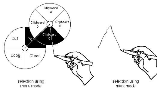
FIG. 1.17 – Sélection d'une commande dans un Marking Menu , par un novice (à gauche) et par un expert (à droite).
