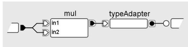
FIG. 3.16 – Deux dispositifs mutables reliés en série. Le premier opère sur des réels ou sur des entiers en fonction de ses connexions en entrée. Le second adapte son type à la fois en entrée et en sortie.
