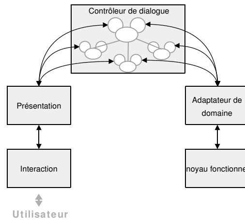
FIG. 2.9 – Le modèle PAC/Amodeus
