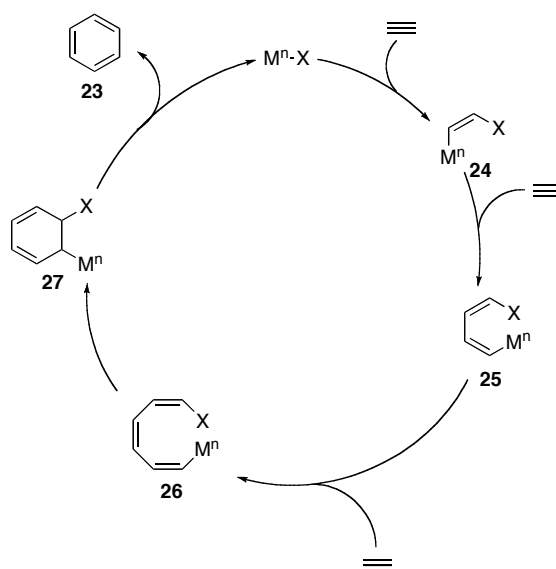
Figure 1-28. Mécanisme proposé pour la cyclotrimérisation d'alcynes via une série d'insertions séquentielles ou carbométallations.
