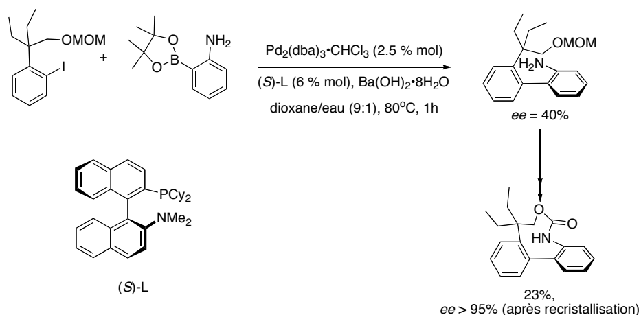
Figure 3-9. Synthèse asymétrique d'un analogue du Rhazinilam.
