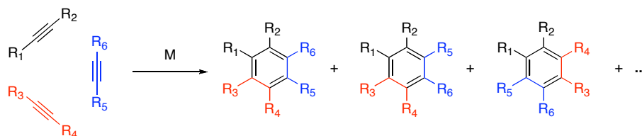
Figure 1-30. Le problème de régiosélectivité de la cyclotrimérisation.
