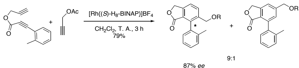
Figure 3-5. Cyclotrimérisation asymétrique des alcynes catalysée par un complexe de Rh(I)/H 8 -BINAP. 9c
