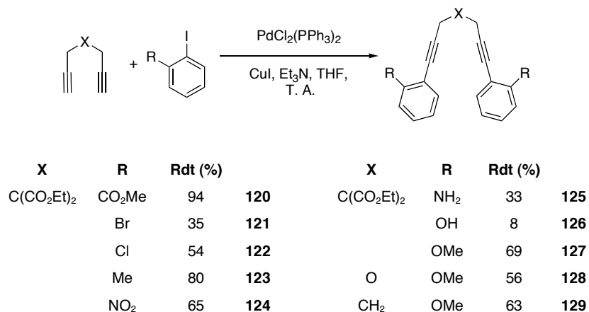
Figure 3-19. Structure des 1,7-diaryl-1,6-diynes ortho -substitués, préparés pour être évalués dans la cyclotrimérisation avec le maléimide.
