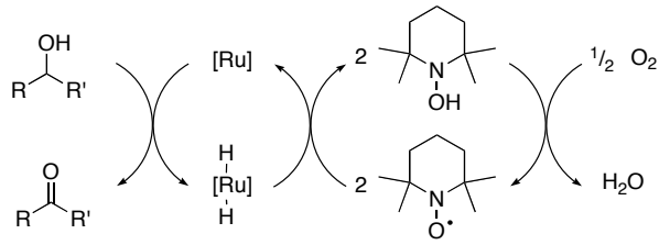
Figure 1-3. Système catalytique Ru/TEMPO pour l'oxydation aérobie des alcools. 11
