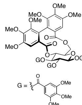
(+)-O-perméthyltellimagrandin II
