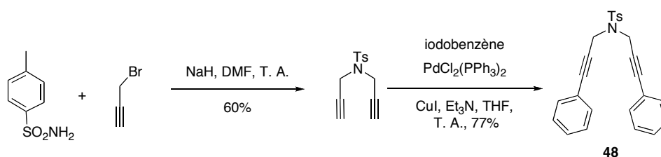
Figure 2-26. Préparation de la sulfonamide 48 .
