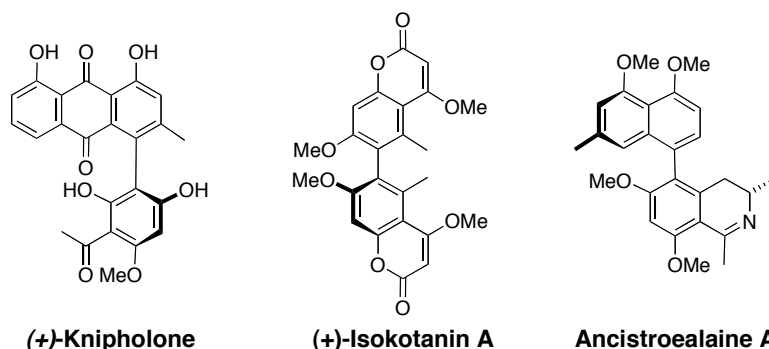
Figure 3-3. Produits naturels d'intérêt pharmaceutique qui présentent de l'atropoisomérisie.
