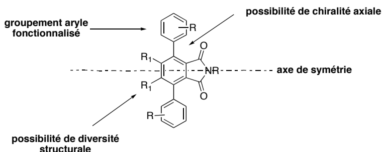
Figure 1-25. Structure générale des catalyseurs à préparer.
