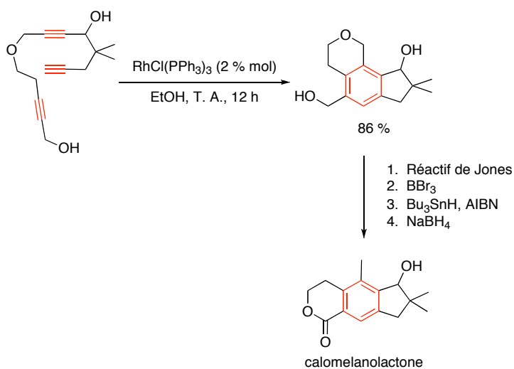
Figure 2-3. Synthèse de la calomelanolactone rapportée par Stevenson et al. 9
