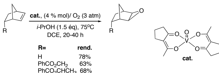
Figure 1-2. Époxydation de dérivés du norbornène catalysée par un complexe de vanadium (IV). 9
