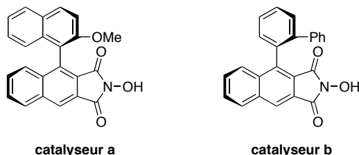
Figure 1-20. Oxydation aérobie asymétrique du 2-méthylindane catalysé par deux analogues chiraux du NHPI.
