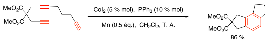
Figure 2-6. Cyclotrimérisation des diyynes catalysée au \text{Co}_2
