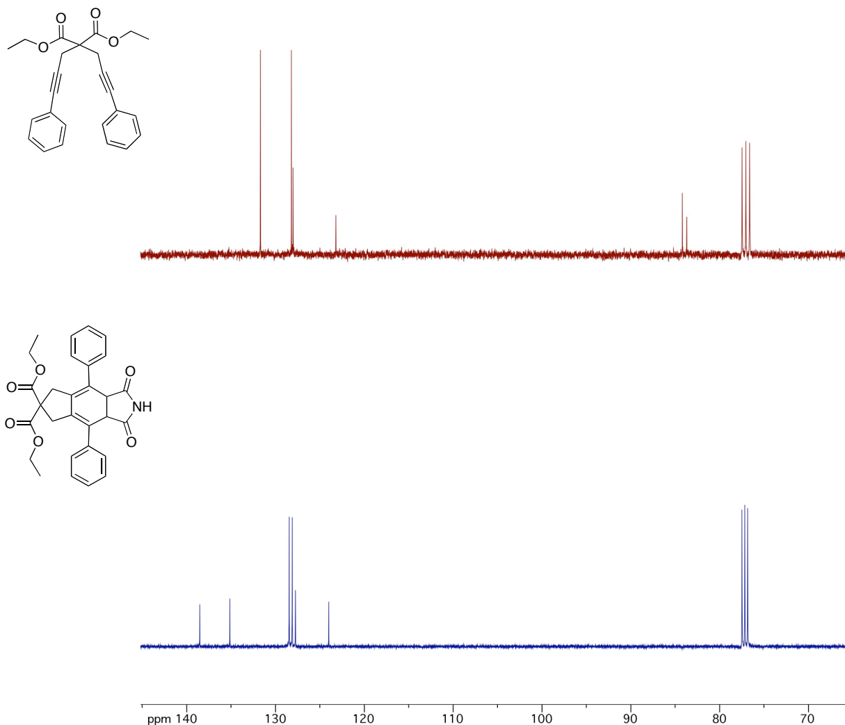
Figure 2-22. En haut: Spectre RMN- ^{13}\text{C} (133 MHz, \text{CDCl}_3 ) du 37 . En bas: Spectre RMN- ^{13}\text{C} (133 MHz, \text{CDCl}_3 ) du produit 45 issu de la cyclotrimérisation du diyne 37 et le maléimide.
