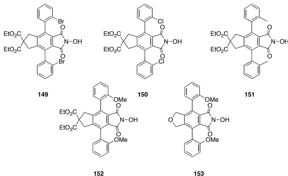
Figure 3-29. Structure des N -hydroxyphthalimides préparés comme mélanges d'atropoisomères.
