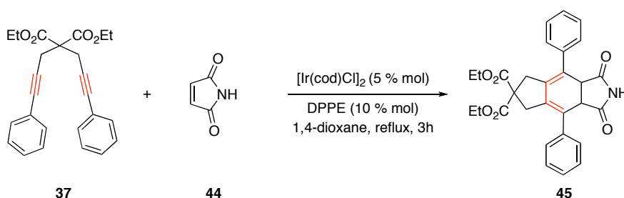
Figure 2-21. Cyclotrimérisation entre le diyne 37 et 44 catalysée à l'iridium.
