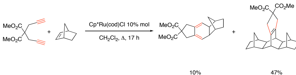
Figure 2-19. Cyclotrimérisation de 1,6-diyne avec le norbornene catalysée par \text{cp}^*\text{Ru}(\text{cod})\text{Cl} .
