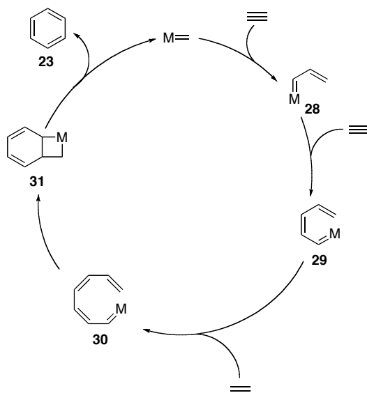
Figure 1-29. Mécanisme proposé pour la cyclotrimérisation d'alcynes via une métathèse en cascade.
