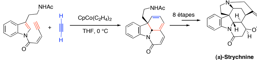
Figure 2-18. Synthèse de la ( \pm )-Strychnine par la cyclotrimérisation catalysée par \text{CoCp}(\text{C}_2\text{H}_4)_2 entre l'acétylène et un dérivé de la tryptamine.
