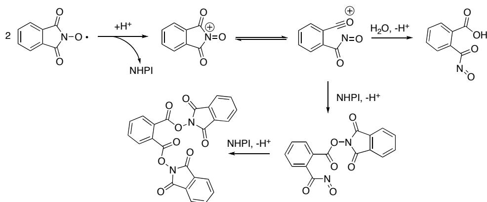
Figure 1-11. Dégradation du radical PINO via la formation d'oligomères rapporté par Masui. 42a
