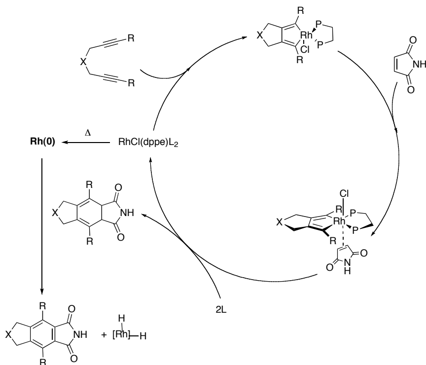
Figure 3-22. Mécanisme de formation du produit aromatisé 141 pendant la cyclotrimérisation [2+2+2] du diyne 121 et le maléimide.
