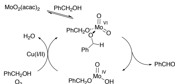
Figure 1-5. Oxydation aérobie d'alcools benzyles catalysé par un système bimétallique molybdène/cuivre. 13
