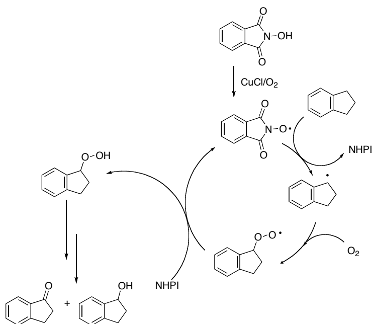
Figure 4-1. Mécanisme de l'oxydation aérobie de l'indane en indanone catalysé par des N -hydroxyphthalimides.
