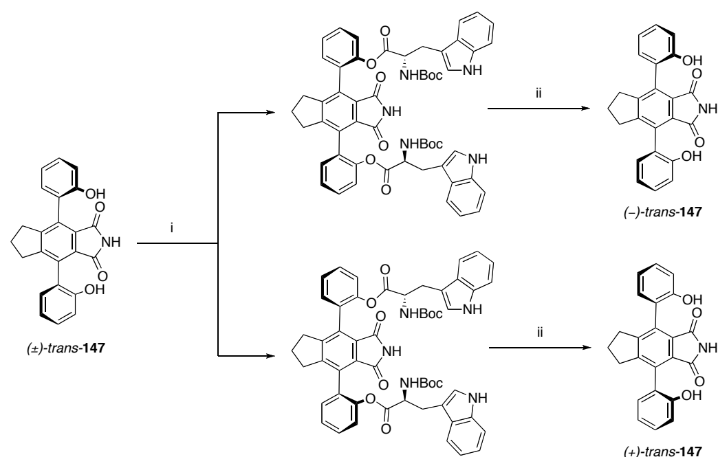
Figure 3-28. Dédoublage du (±)- trans -147 par le biais d'une dérivatisation avec le N -(α)-Boc-L-tryptophane. Conditions de réaction et réactifs: (i) (a) DCC, DMAP, N -(α)-Boc-L-tryptophane, CH 2 Cl 2 , T. A. (b) chromatographie sur gel de silice. (ii) (a) LiOH, MeOH, T. A. (b) TFA.
