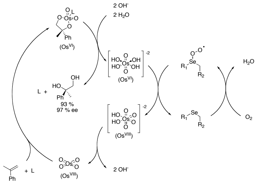
Figure 1-4. Dihydroxylation asymétrique aérobie catalysée par l'osmium. 12
