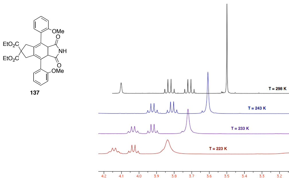
Figure 3-24. Etude RMN- 1 H (CDCl 3 , 400 MHz) à basse température du cyclohexadiène 137 .
