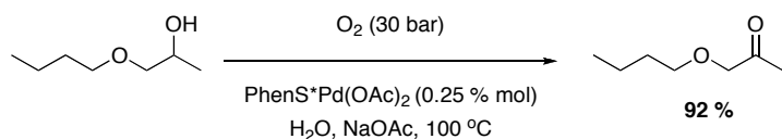
Figure 1-1. Oxydation aérobie d'alcools catalysée par un complexe hydrosoluble de palladium (II) rapportée par Sheldon et al. 8
