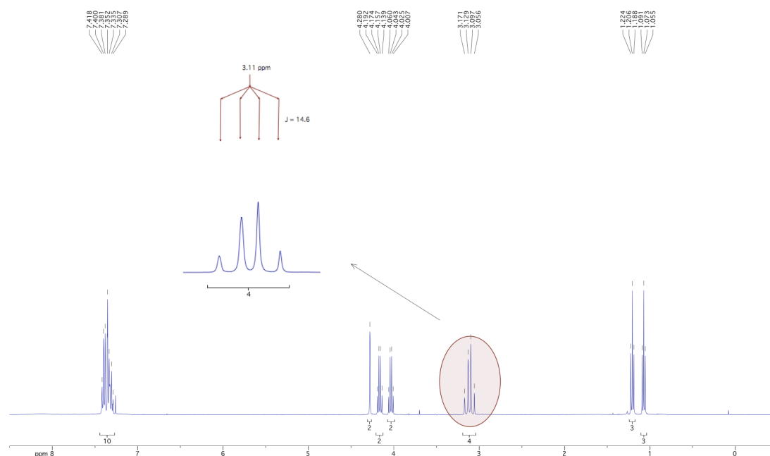
Figure 2-23. Spectre RMN- 1 H (CDCl 3 , 400 MHz) du produit 45 issu de la cyclotrimérisation du diyne 37 et le maléimide 44 .
