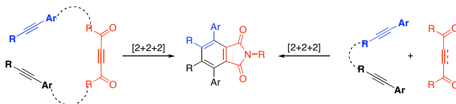
Figure 1-32. Stratégie envisagée pour la préparation de précurseurs de N -hydroxyphthalimides.
