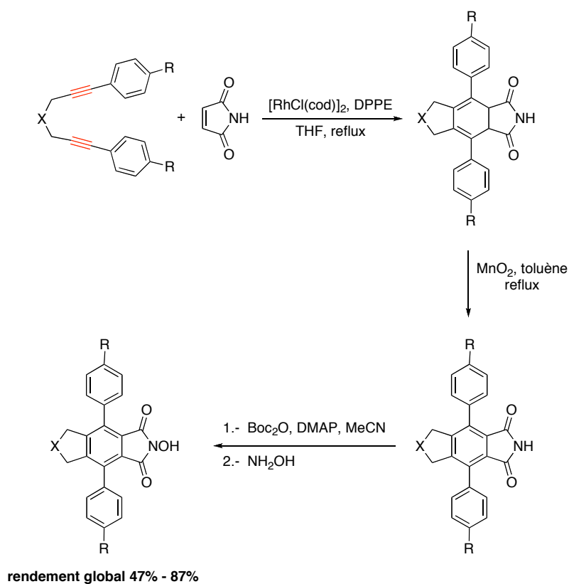
Figure 5-1. Synthèse des N -hydroxyphthalimides hautement fonctionnalisés.
