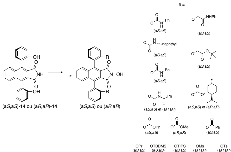
Figure 1-23. Analogues chiraux du NHPI préparés par Nechab.
