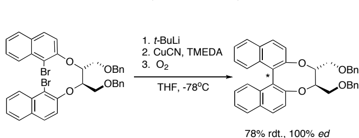
Figure 3-8. Préparation de biaryles via l'utilisation d'un pont présentant deux centres asymétriques.
