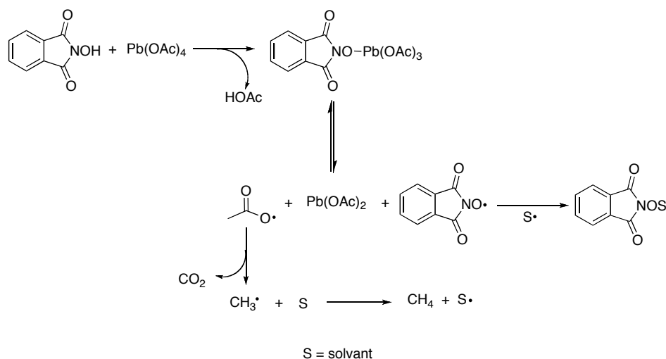
Figure 1-9. Préparation in-situ du PINO avec \text{Pb}(\text{OAc})_4 et dérivatisation avec le solvant.
