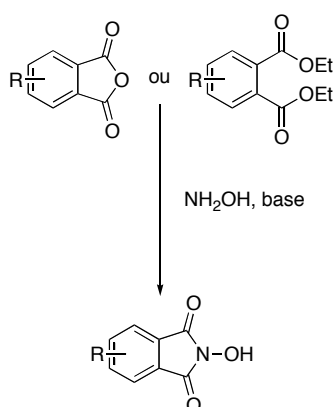
Figure 1-18. Méthodologie générale pour la préparation des analogues achiraux du NHPI.
