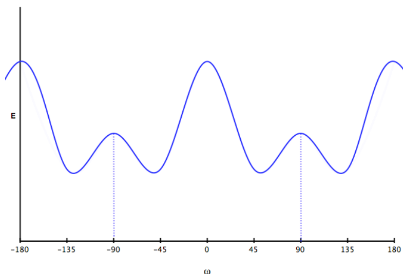
Figure 3-2. Profil énergétique de l'interconversion conformationnelle du diphenyle.
