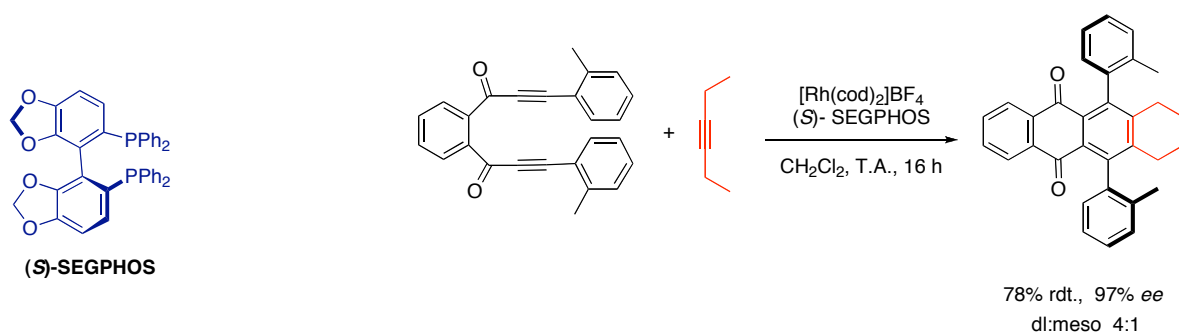
Figure 3-16. Synthèse énantiosélective des systèmes triaryliques via une cyclotrimérisation catalysée au rhodium. 20
