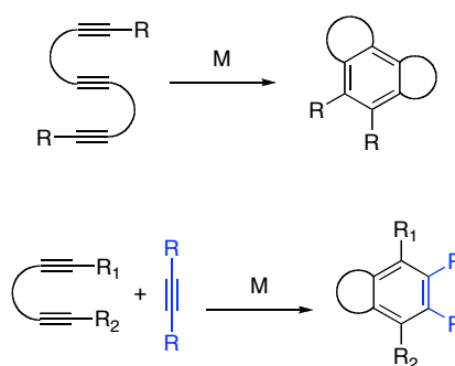
Figure 1-31. En haut: version intramoléculaire de la cyclotrimérisation. En bas: version partiellement intramoléculaire.
