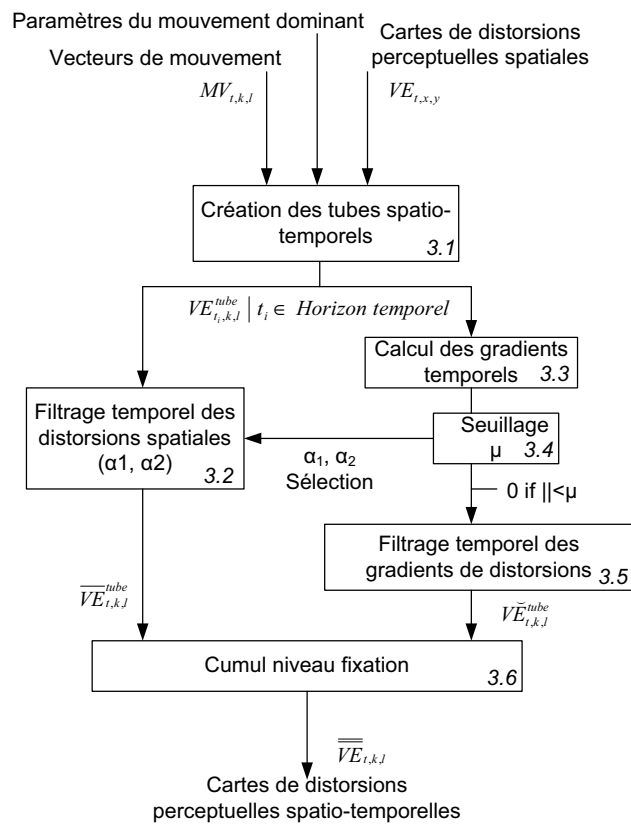
FIGURE 3.3 – Structure du cumul temporel court terme, ou autrement dit de l'étape d'évaluation des distorsions perceptuelles spatio-temporelles.
