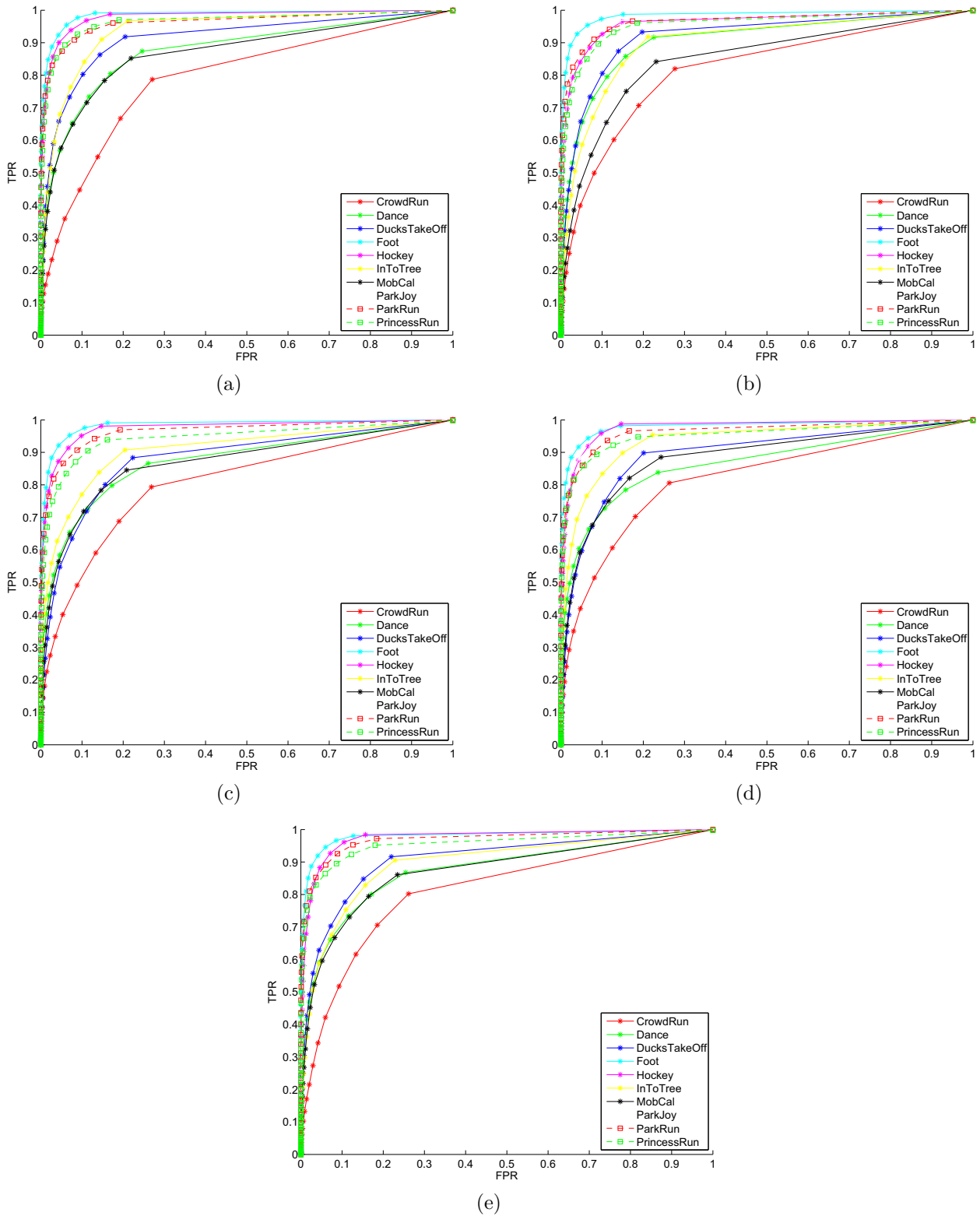
FIGURE 9.7 – Courbes ROC associées à la comparaison A. Les figures (a), (b), (c), (d) et (e) représentent respectivement les graphes correspondant à la présentation de la vidéo de référence en tâche de qualité précédant la présentation des versions dégradées pour les cinq niveaux de dégradations (du niveau de dégradations le plus faible au niveau le plus élevé). Ces courbes sont utilisées pour calculer les valeurs d’AUC correspondantes.
