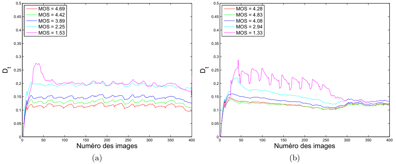
FIGURE 6.2 – Évolution temporelle des notes intermédiaires D_t , pour deux séquences de la base de test (cf. section 6.3.1) et cinq niveaux de dégradation : (a) ParkRun , (b) MobCal . L'axe horizontal représente le numéro d'images, et axe vertical représente l'échelle de distorsions (de 0 pour la meilleure qualité à 0.5 pour la pire qualité). Pour chaque niveau de dégradations les MOS sont donnés.
