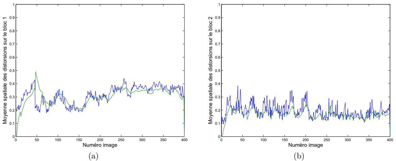
FIGURE 3.9 – Évolution temporelle de la distorsion moyenne des cartes de distorsions purement spatiale VE (en bleu) et spatio-temporelle \overline{VE} (en vert) dans le bloc 1 (a), et le bloc 2 (b) de la séquence CrowdRun (cf. figure 3.8).
