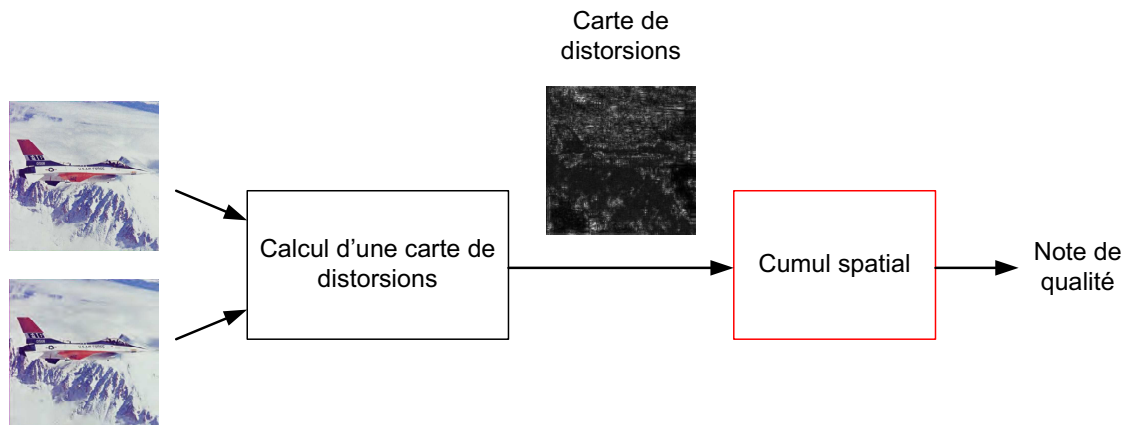
FIGURE 4.6 – Structure générale d'une métrique de qualité d'images reposant sur le calcul de cartes de distorsions.
