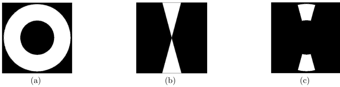
FIGURE B.3 – Construction d’un filtre Cortex : le filtre DoM utilisé en (a), le filtre Fan utilisé en (b), et en (c) le filtre Cortex résultant.
