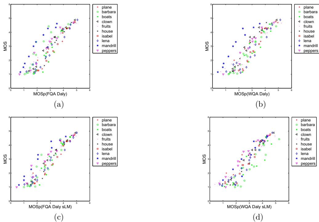
FIGURE 5.4 – Nuage de points des couples (MOS, MOS_p) par image de référence : (a), (c) pour FQA 1 et FQA 2 respectivement ; (b), (d) pour WQA 1 et WQA 2 respectivement.
