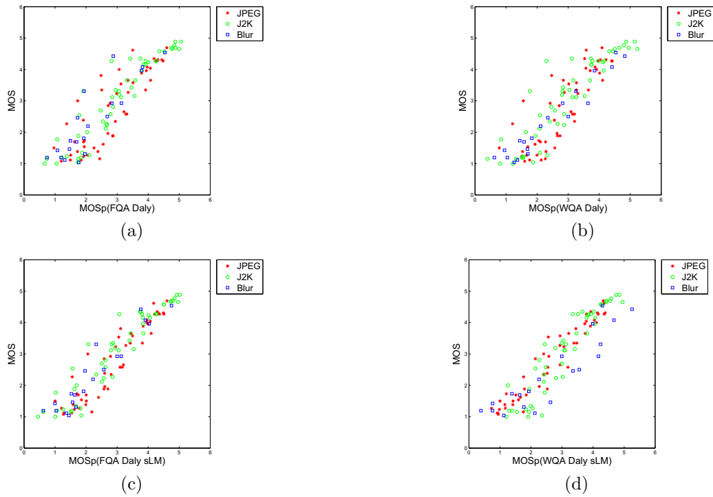
FIGURE 5.3 – Nuage de points des couples (MOS, MOS_p) par type de distortions : (a), (c) pour FQA 1 et FQA 2 respectivement ; (b), (d) pour WQA 1 et WQA 2 respectivement.
