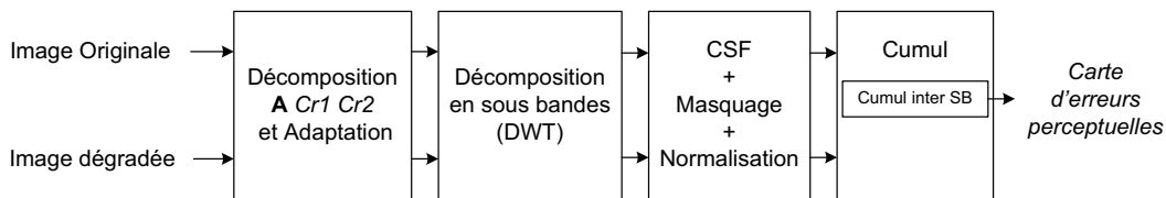
FIGURE 2.5 – Structure du modèle basé ondelettes (WQA).
