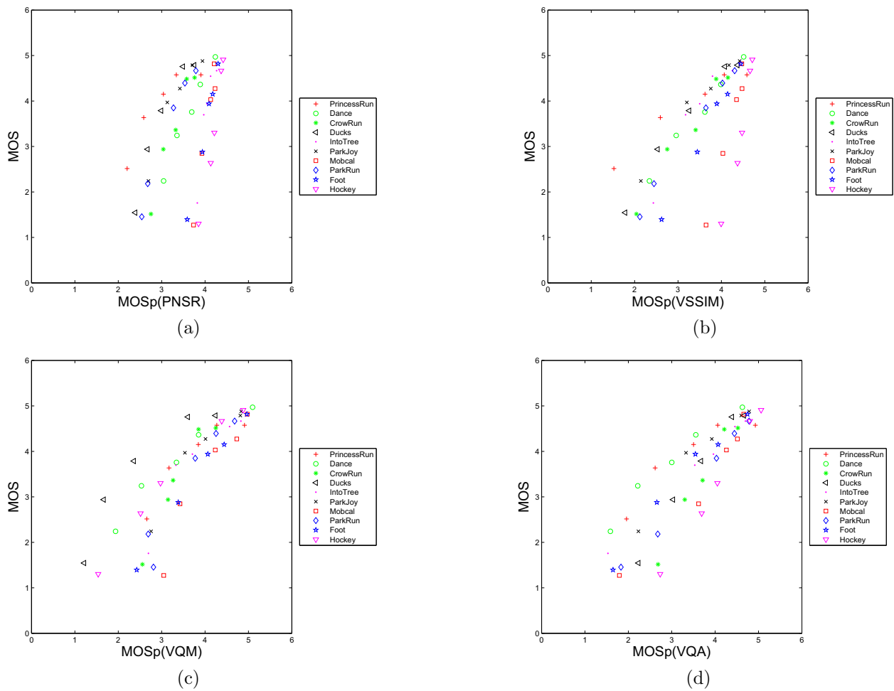
FIGURE 6.6 – Nuage de points des couples (MOS, MOS_p) par vidéo de référence. Chaque point représente une séquence vidéo. Le même symbole est utilisé pour toutes les vidéos dégradées issues de la même vidéo de référence : (a) PSNR, (b) VSSIM, (c) VQM et (d) VQA.
