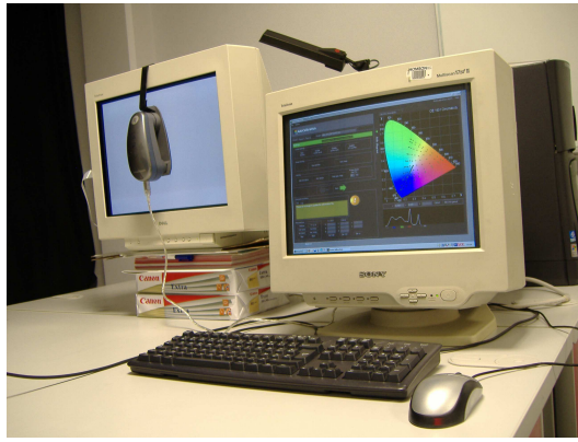
FIGURE 2.6 – Mesures des gammas d'un écran CRT à l'aide d'un colorimètre et d'un logiciel adapté.
