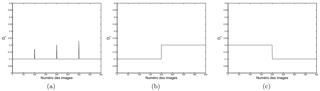
FIGURE 6.4 – Exemples d'évolutions temporelles des notes intermédiaires D_t : (a) illustration de la saturation perceptuelle, (b,c) illustration du comportement asymétrique. L'axe horizontal représente le numéro d'images, et l'axe vertical représente l'échelle de distorsions (de 0 pour la meilleure qualité à 0.5 pour la pire qualité).
