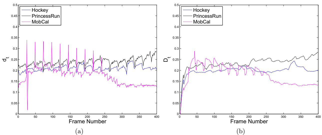
FIGURE 6.8 – Évolution temporelle des notes de distorsions par image d_t (a), et D_t (b), pour trois séquences dégradées de la base de test : Hockey (MOS=1.4), PrincessRun (MOS=2.6) and MobCal (MOS=1.3). L'axe horizontal représente le numéro d'images, et l'axe vertical représente l'échelle de distorsions (de 0 pour la meilleure qualité à 0.5 pour la pire qualité).
