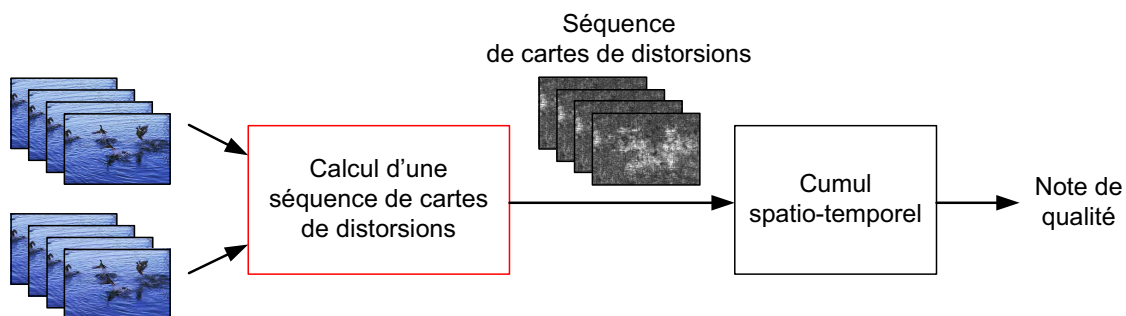
FIGURE 3.1 – Structure générale d’une métrique de qualité de vidéos reposant sur le calcul de séquences de cartes de distorsions.
