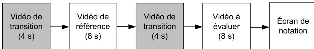
FIGURE 9.3 – Déroulement d’une présentation en tâche d’évaluation de qualité (protocole DSIS).
