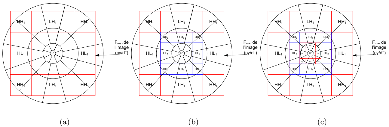
FIGURE 2.11 – Illustration de la correspondance entre la DCP et la DWT en fonction du niveau de décomposition de la DWT : (a) un niveau, (b) deux niveaux et (c) trois niveaux.
