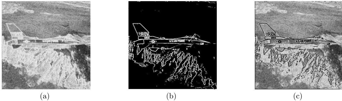
FIGURE 2.25 – (a) est la carte d'entropie de l'image Avion , (b) est la carte de détection des contours de l'image Avion , et (c) la carte d'entropie corrigée de l'image Avion .
