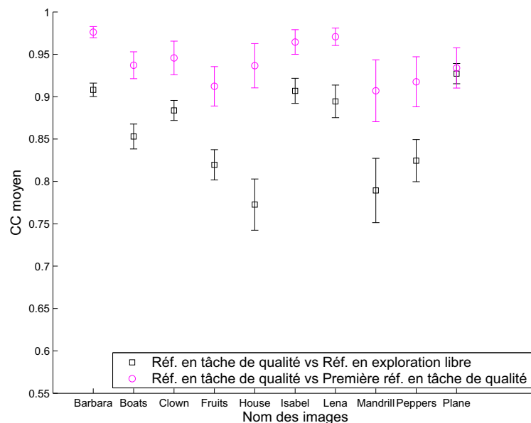
FIGURE 8.11 – Moyennes des Coefficients de Corrélation calculées pour chaque image d'origine. Comme le montre la figure 8.9, les valeurs de CC sont calculées, d'une part entre la carte de saillance de l'image de référence en tâche de qualité et la carte de saillance d'image de référence en exploration libre (test A), d'autre part entre la carte de saillance de l'image de référence en tâche de qualité et la première carte de saillance provenant de la première présentation de l'image de référence en tâche de qualité (test B). Pour chaque valeur l'intervalle de confiance à 95% est donné.
