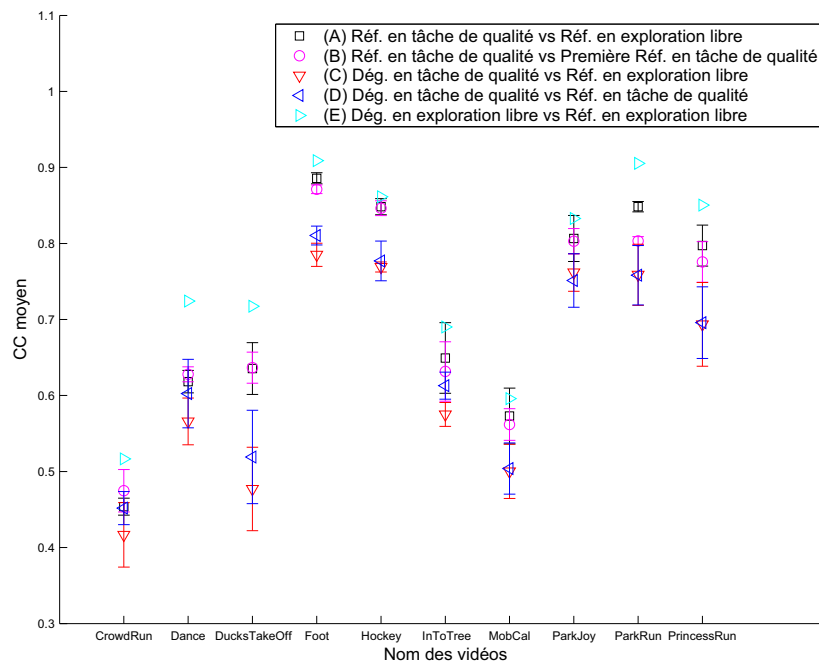
FIGURE 9.9 – Moyennes des Coefficients de Corrélation calculées pour chaque vidéo d'origine. Comme le montre la figure 8.9, les valeurs de CC sont calculées pour les cinq tests (cf. figure 9.6 : A, B, C, D et E). Pour chaque valeur, l'intervalle de confiance à 95% est donné.
