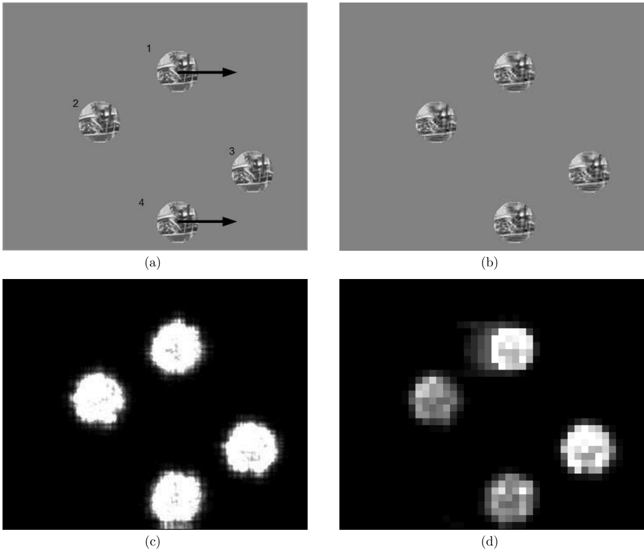
FIGURE 3.7 – Exemple d’une séquence de synthèse : (a) version originale (avec annotations), (b) version dégradée, (c) et (d) cartes de distorsions VE (purement spatiale) et \overline{VE} (spatio-temporelle) respectivement. Dans cette séquence deux « extraits » d’images sont en mouvement de translation vers la droite (notés 1 et 4) et deux sont fixes (notés 2 et 3). Deux « extraits » d’images (1 et 3) sont dégradées à une fréquence temporelle et les deux autres (2 et 4) ne varient pas temporellement.
