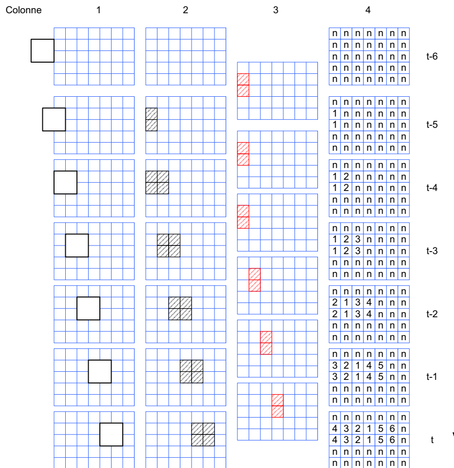
FIGURE 3.5 – Illustration du calcul de l'horizon temporel d'un tube spatio-temporel. Les lignes correspondent à des images successives de t - 6 à t . De gauche à droite, la première colonne présente un objet en déplacement. La seconde colonne présente la carte des blocs outlier en terme de mouvement. La troisième colonne présente la carte des changements de classification ( inlier/outlier ) entre les blocs de deux images successives et en tenant compte du mouvement de ces blocs entre les deux images. La quatrième colonne présente pour chaque image, la taille en nombres d'images de l'horizon temporel des tubes spatio-temporels partant de chaque bloc, la valeur n correspondant à la durée maximale d'un tube soit 400ms exprimée en nombre d'images.
