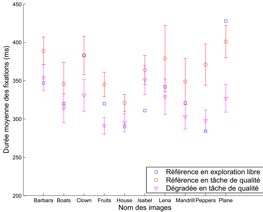
FIGURE 8.8 – Durée moyenne des fixations par image en exploration libre et en tâche d'évaluation de qualité. L'intervalle de confiance à 95% est donné pour chaque cas.
