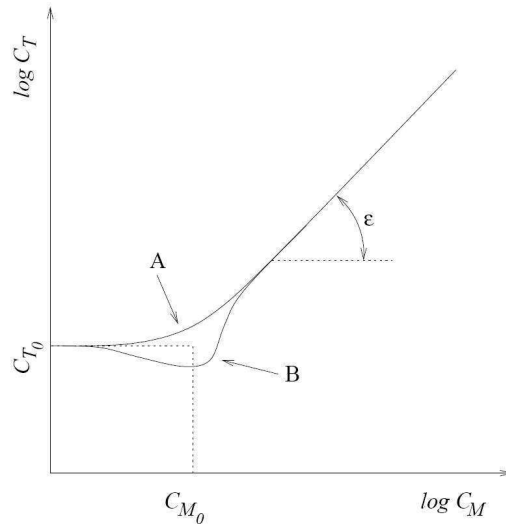
FIGURE 1.7 – Illustration de courbes de masquage classiques. Les valeurs de contraste seuil de la cible C_T sont donnés en fonction des valeurs de contraste du signal masquant C_M . Pour des stimuli dont les caractéristiques ne sont pas trop proches l'effet principal est le masquage (A). Dans le cas où les stimuli sont très proches un effet de facilitation (B) peut apparaître pour des valeurs de contraste C_M pas très grandes.
