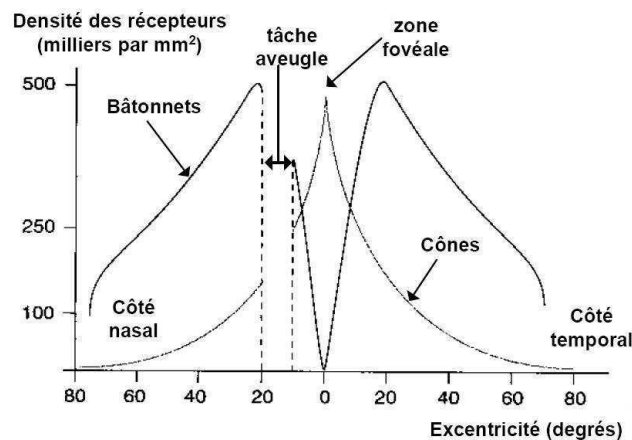
FIGURE A.2 – Répartition des cellules photoréceptrices sur la rétine.
