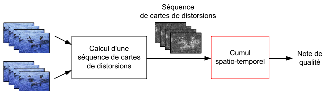
FIGURE 4.8 – Structure générale d'une métrique de qualité de vidéos reposant sur le calcul de séquences de cartes de distorsions.
