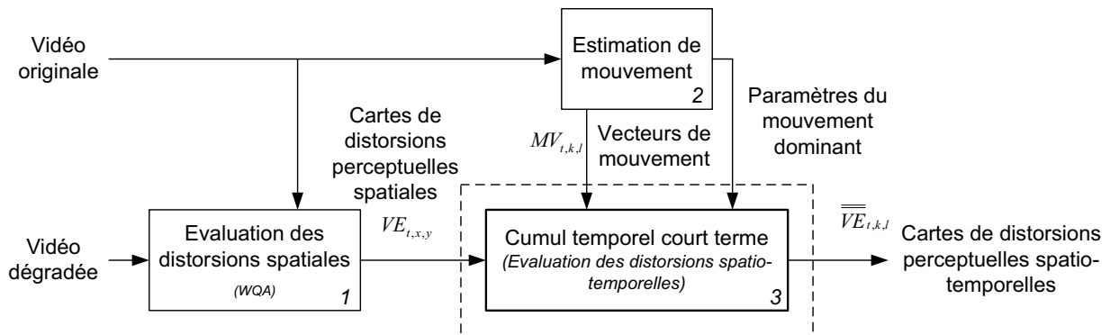
FIGURE 3.2 – Structure générale du modèle de construction de séquences de cartes d'erreurs perceptuelles.
