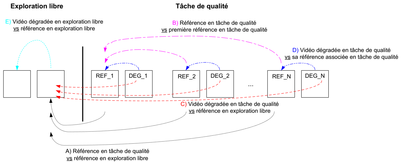
FIGURE 9.6 – Illustration des différentes comparaisons effectuées entre les séquences de saillance.
