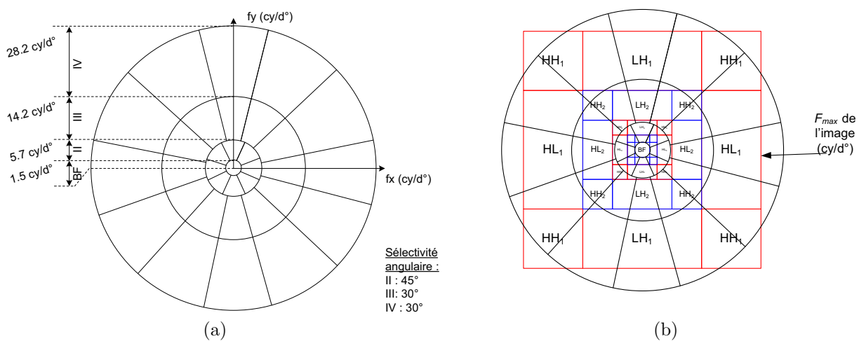
FIGURE 2.12 – (a) Décomposition en canaux perceptuels (DCP). (b) Décomposition en ondelettes dépendante des fréquences spatiales : mise en correspondance de la sous-bande basse fréquence de la DCP et de la DWT, ici le niveau de décomposition est égal à quatre.
