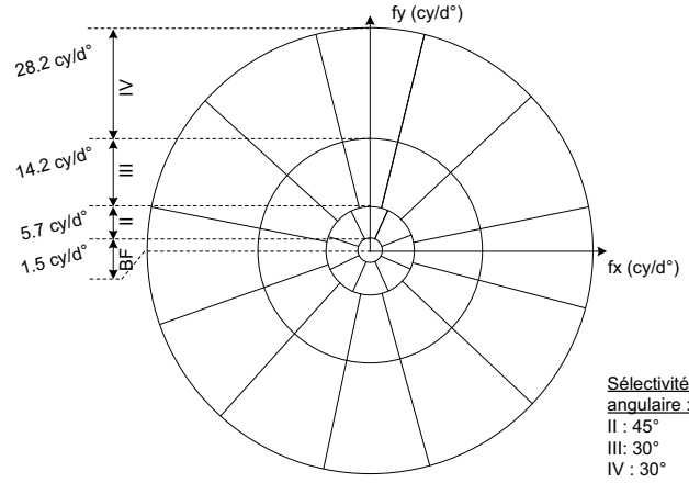
FIGURE 2.8 – Pavage du plan fréquentiel pour la Décomposition en Canaux Perceptuels (DCP) de la composante A. Les dix sept sous-bandes de la DCP sont réparties sur les quatre couronnes (BF, II, III, IV).
