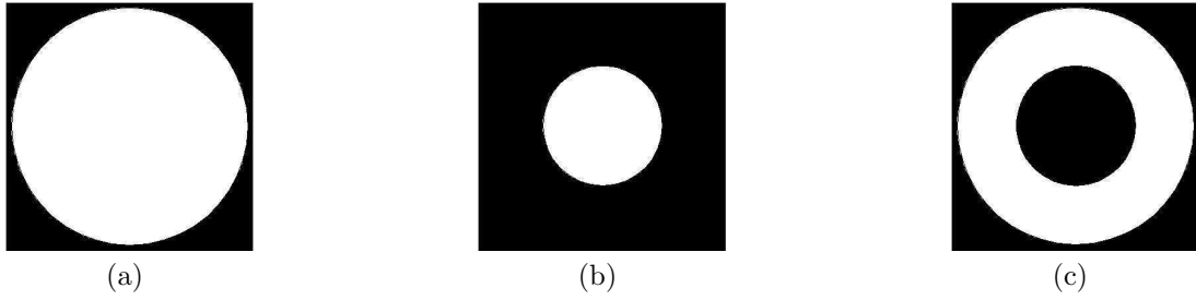
FIGURE B.1 – Construction d'un filtre DoM : les 2 filtres Mesa utilisés en (a) et en (b), et en (c) le filtre DoM résultant (correspondant à la couronne IV de la DCP).
