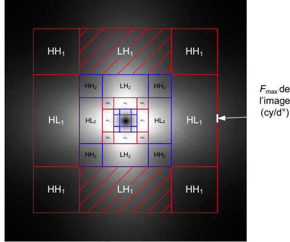
FIGURE 2.14 – Le calcul des valeurs N_{l,o}^{CSF} de chaque sous-bande s'effectue en moyennant les valeurs de la CSF 2D de Daly sur la gamme de fréquences spatiales de chaque sous-bande. Pour la sous-bande LH_1 il s'agit des valeurs de la zone hachurée.
