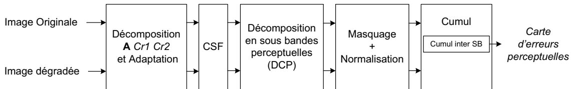
FIGURE 2.4 – Structure du modèle basé Fourier (FQA).
