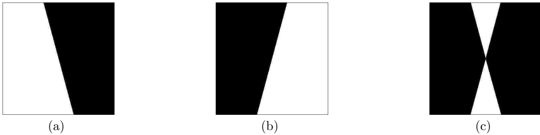
FIGURE B.2 – Construction d'un filtre Fan : les 2 filtres Step utilisés en (a) et en (b), et en (c) le filtre Fan résultant (correspondant à l'orientation 4 de la DCP).
